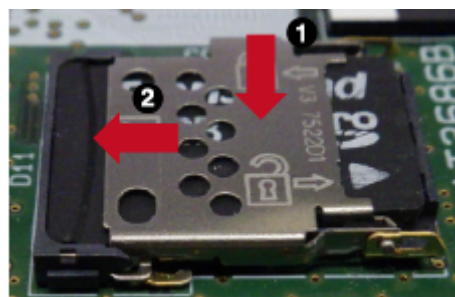
図 3.70 カバーをロックする
