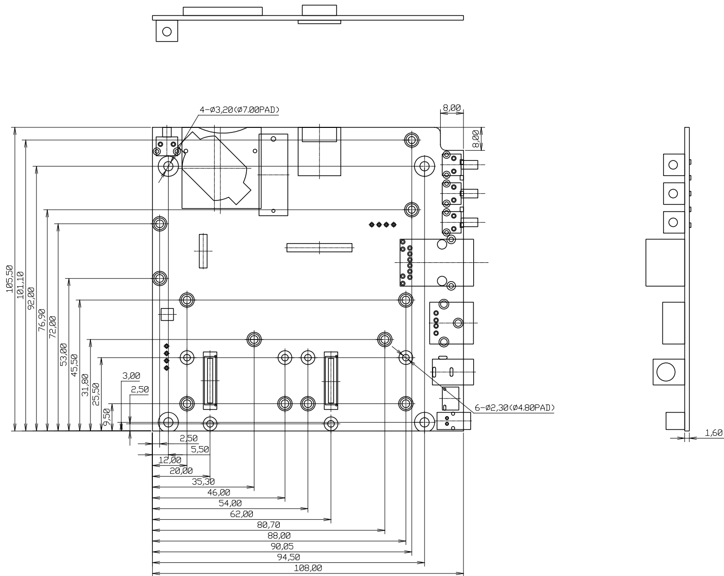
図 17.1 ベースボードの基板形状および固定穴寸法
