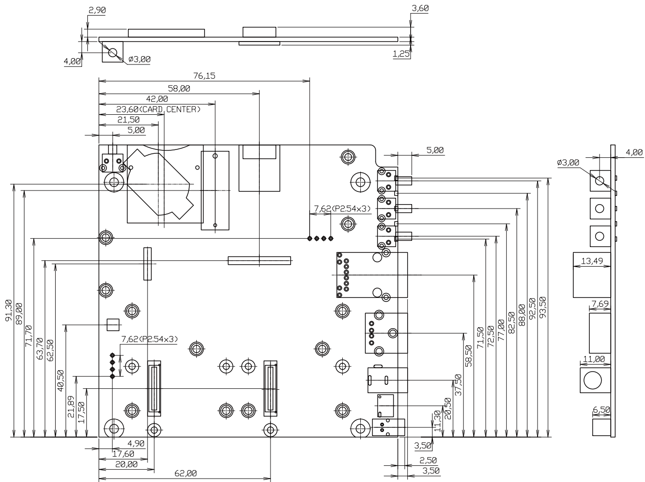
図 17.2 ベースボードのコネクタ中心寸法
