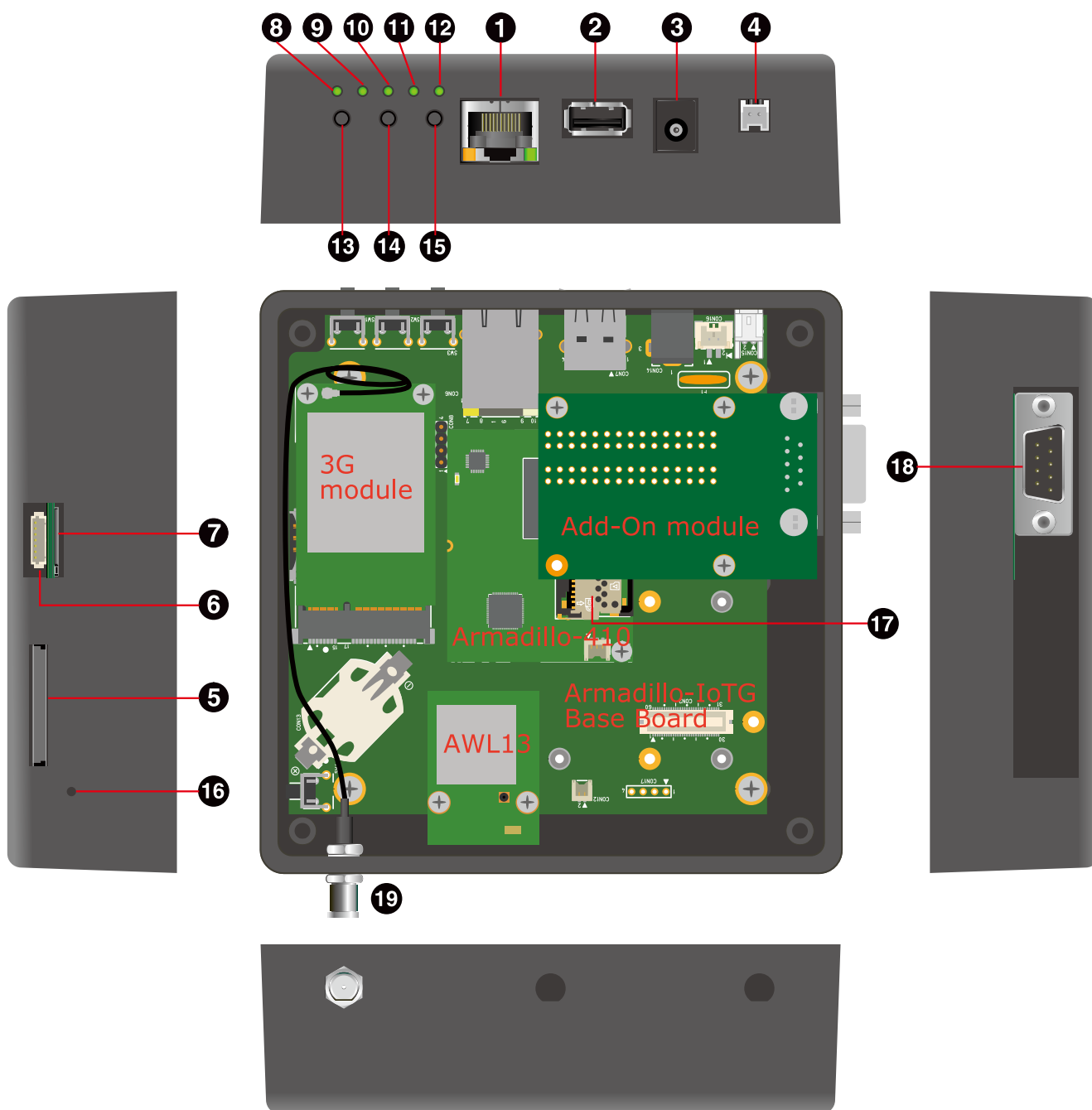
図 3.1 Armadillo-IoT ゲートウェイの外観
