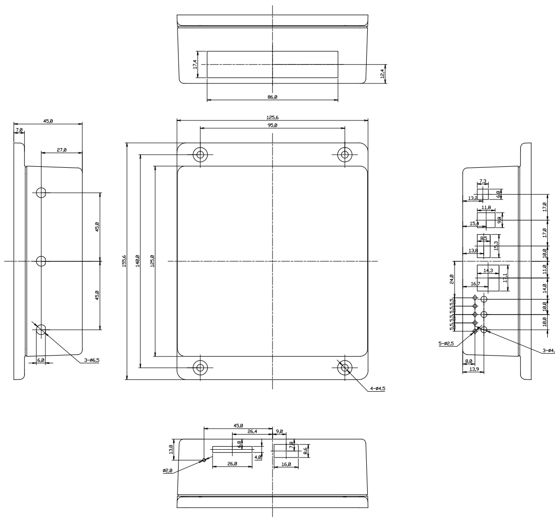
図 19.6 Armadillo-IoT ゲートウェイの筐体 形状図
