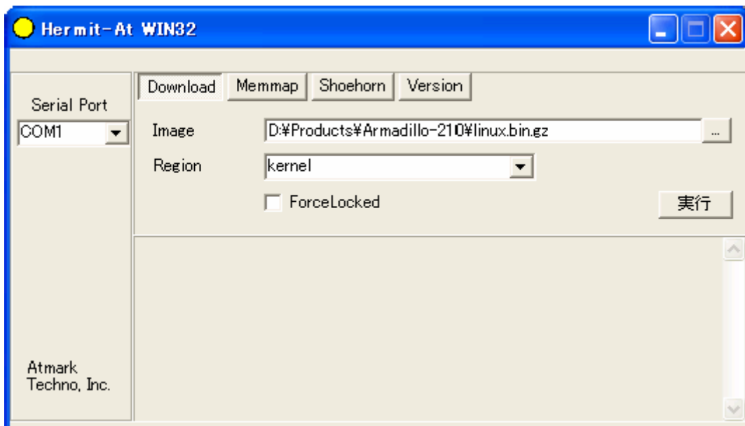
図 5.3. Download 画面
