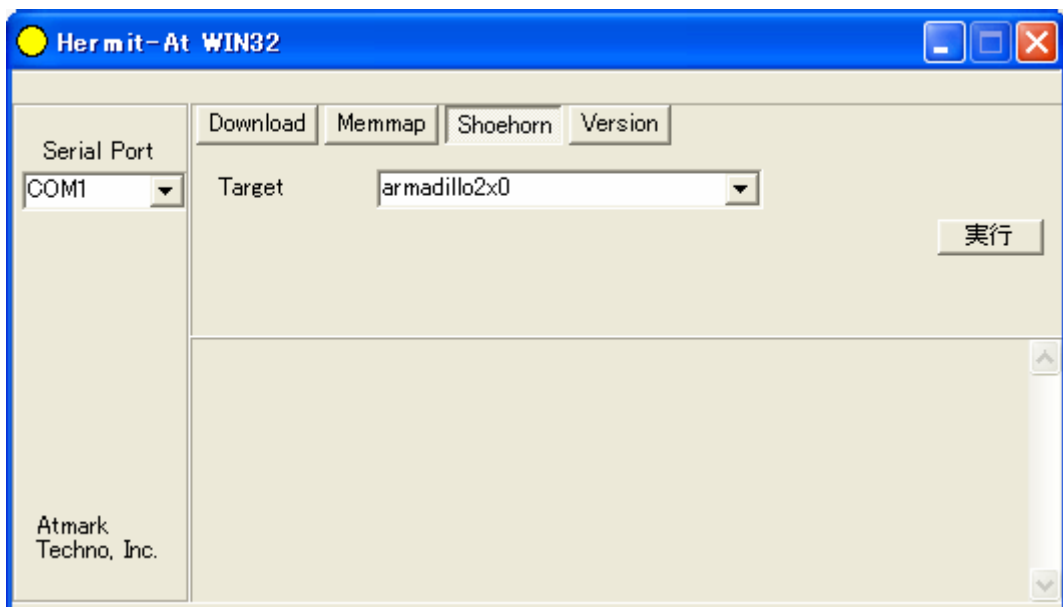
図 6.2. Shoehorn 画面
