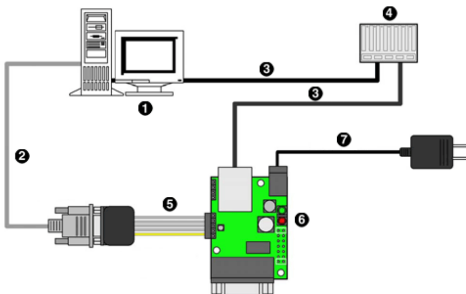
図 2.1. Armadillo-210 接続例
