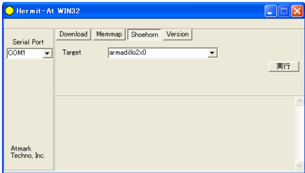
図 6-2 Shoehorn 画面
