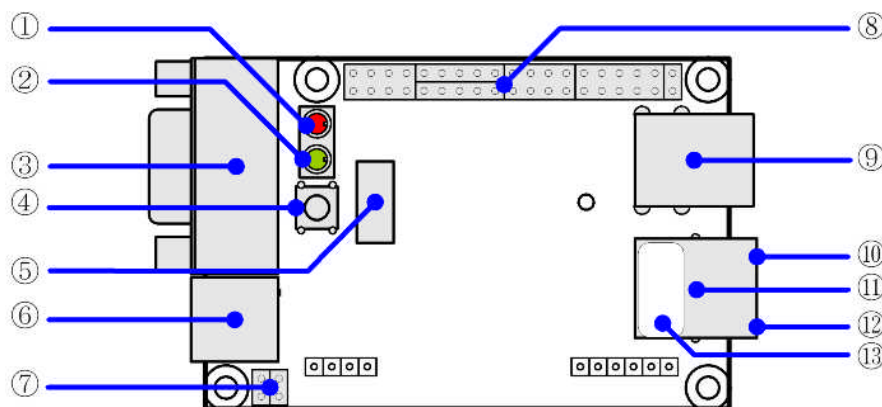
図 3.1. Armadillo-220 のインターフェース
