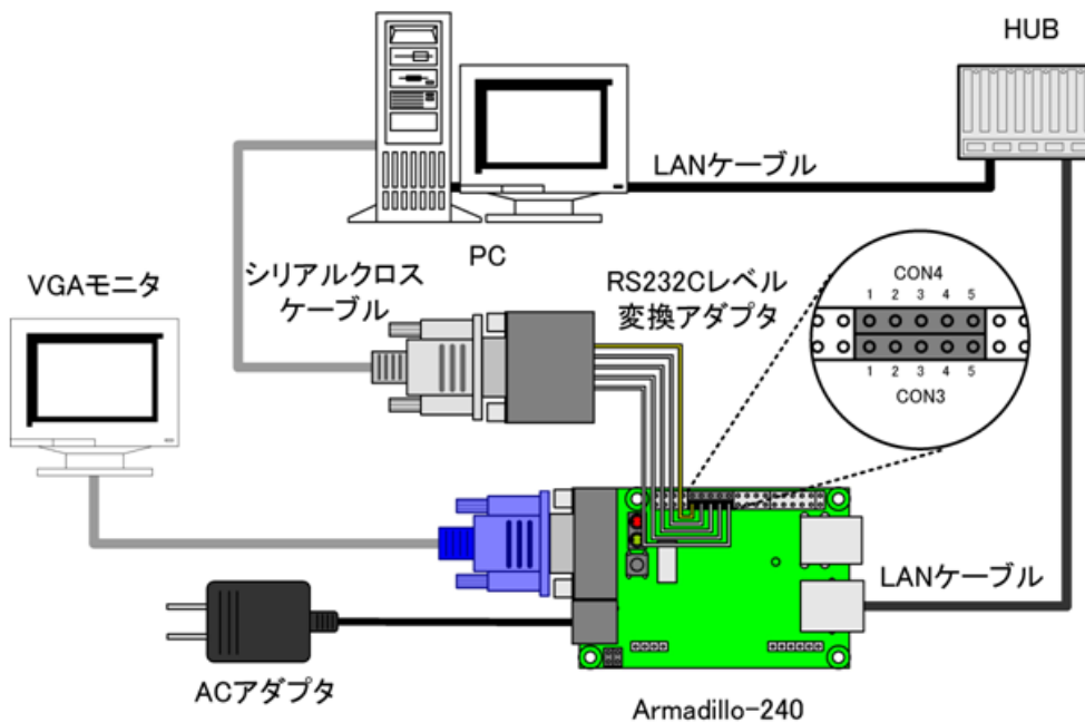
図 3.3 Armadillo-240 接続例
