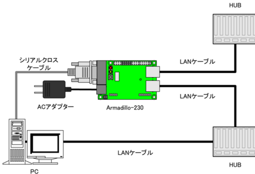
図 3.2 Armadillo-230 接続例
