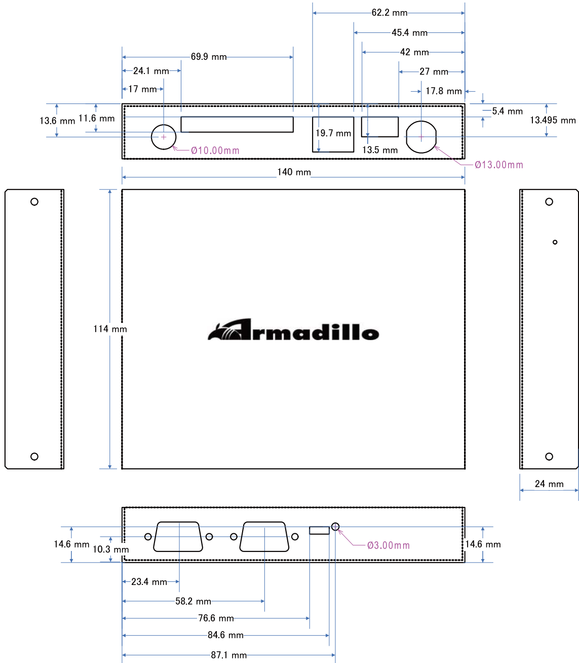
Armadillo-300 ケース形状図
