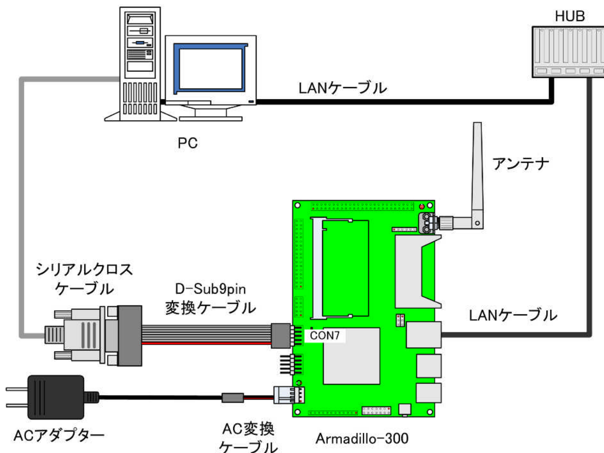
図 3.1. 接続図
