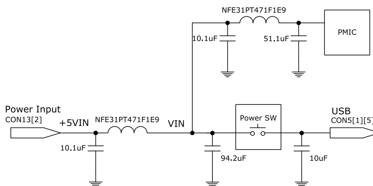
図 9.3 Armadillo-410+Armadillo-410 拡張ボードの電源の入力容量構成
