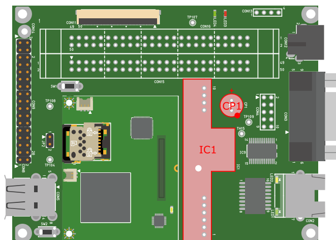
図 9.5 PoE 用部品の実装位置
