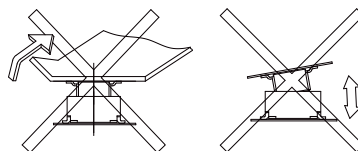
図 9.14 コネクタ抜去時の取扱い上の注意 3
