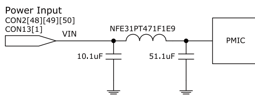
図 5.2 Armadillo-410 の電源の入力容量構成
