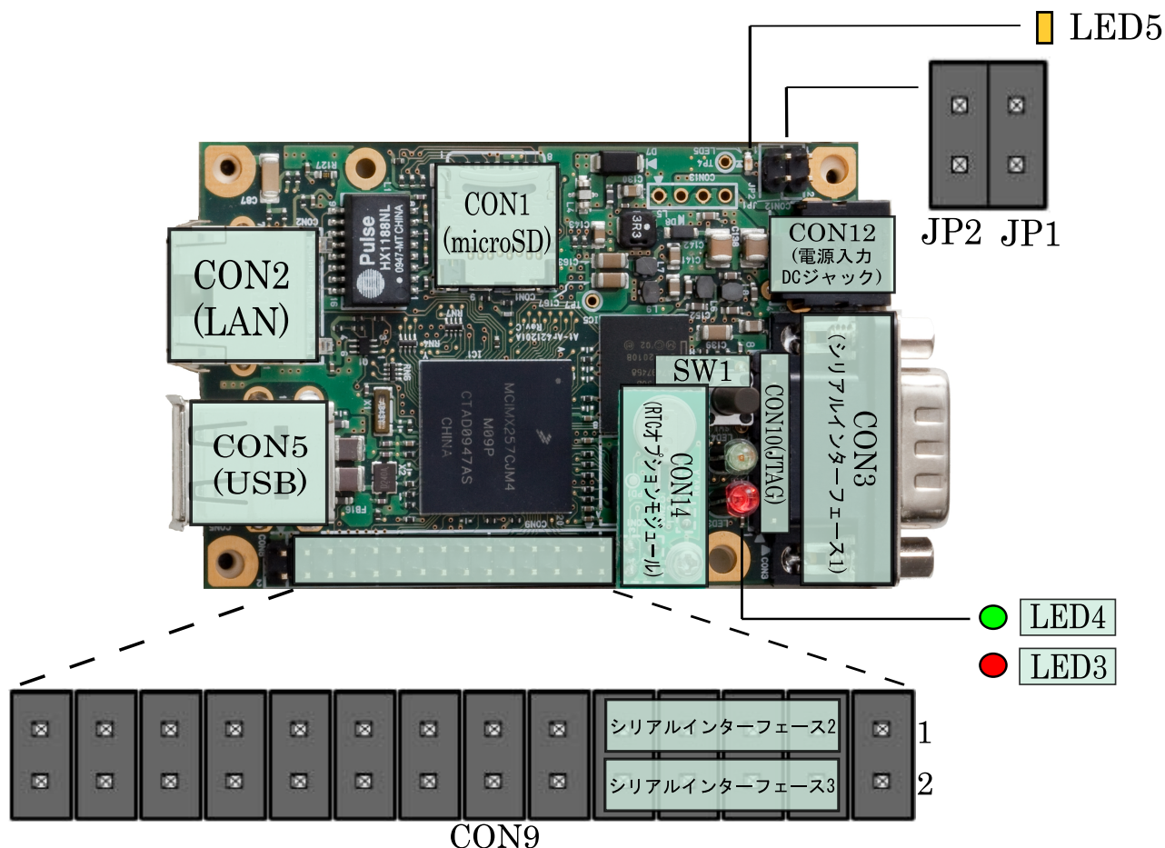
図 2.1 見取り図
