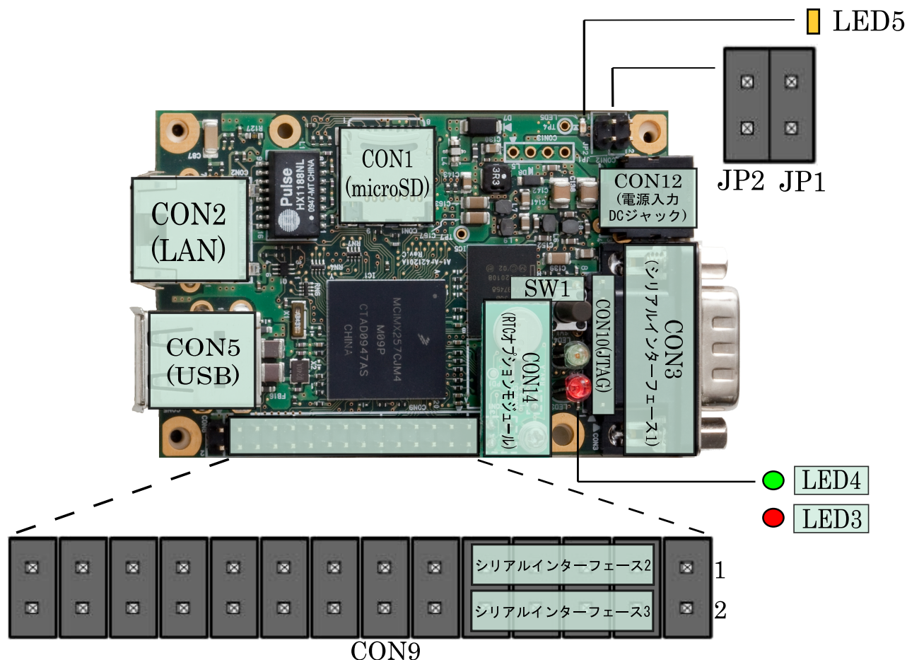
図 3.1 見取り図
