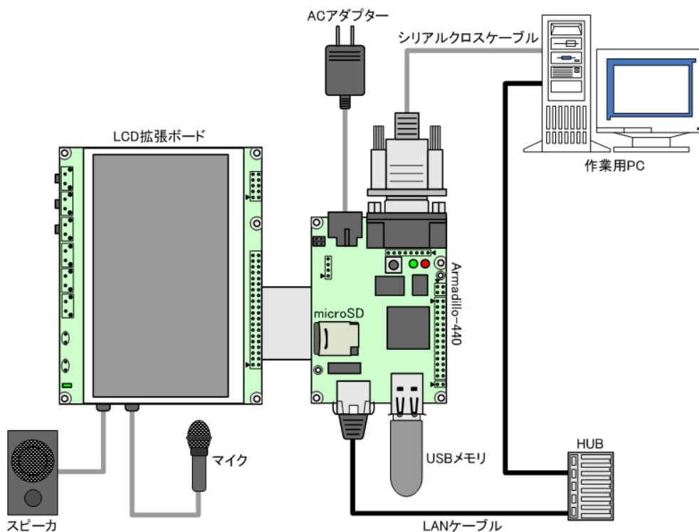
図 3.2 接続図
