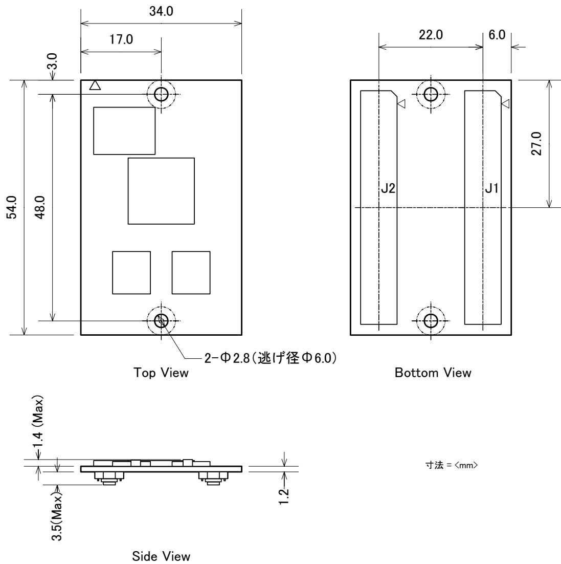
図 6-2 Armadillo-500 CPU モジュールの基板形状
