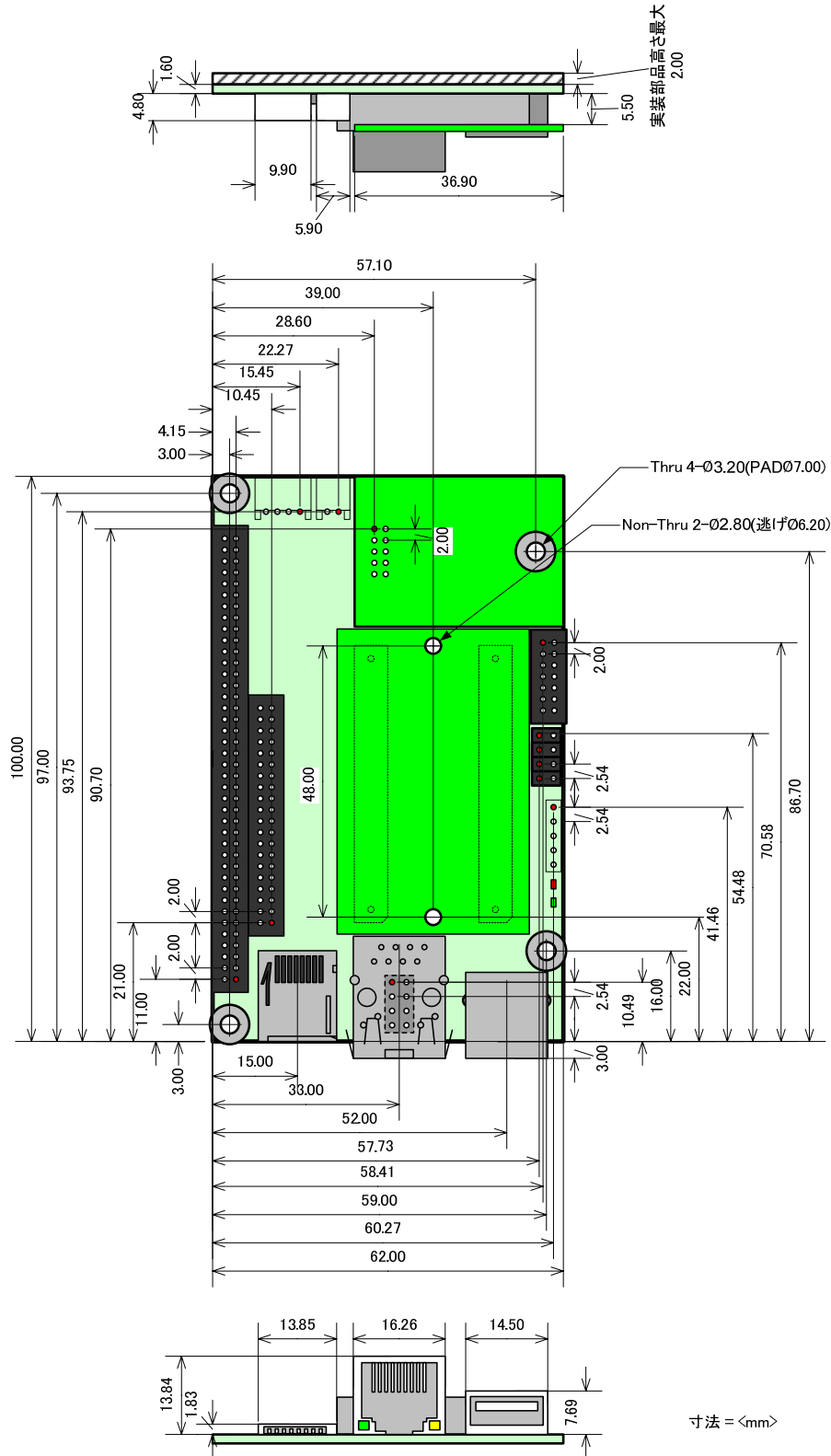
図 6-1 Armadillo-500 FX の基板形状
