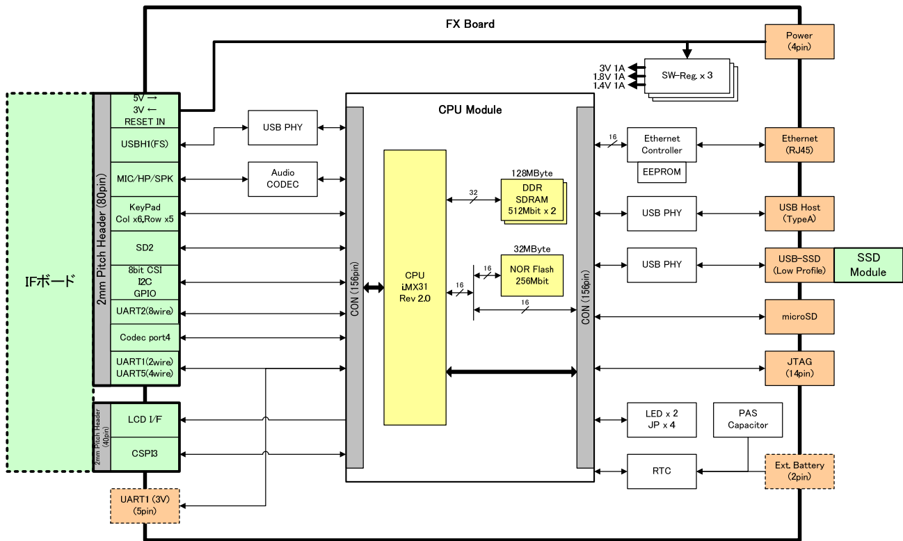
図 3-1 Armadillo-500 FX ブロック図
