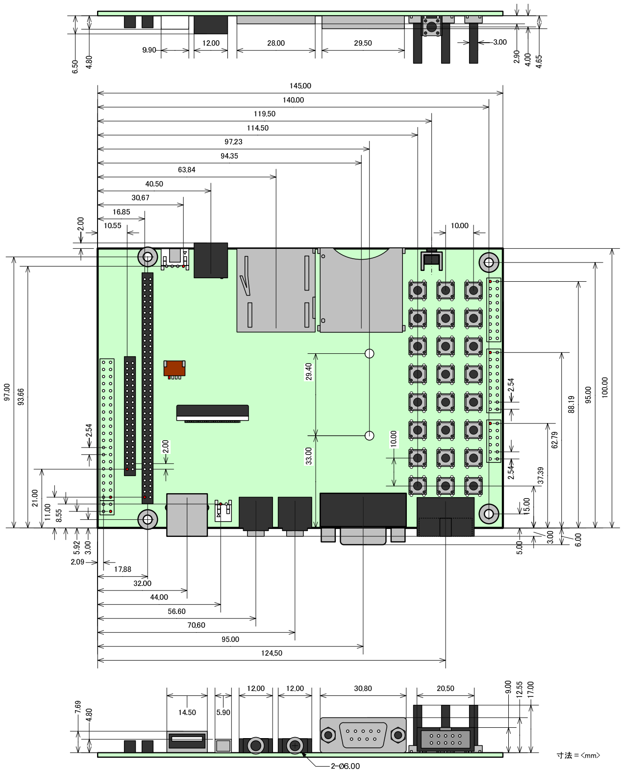
図 5-1 Armadillo-500 FX インターフェースボードの基板形状
