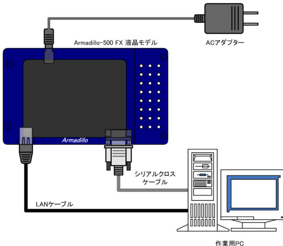
図 2.2. 接続図
