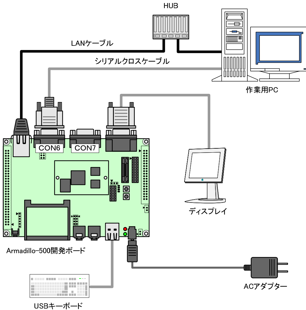
図 2-2 接続図
