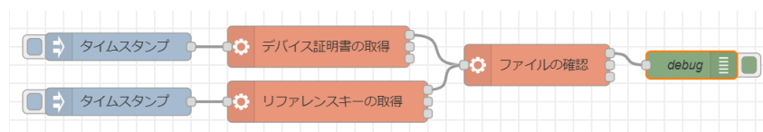
図 4.35 デバイス証明書を取得するフロー
