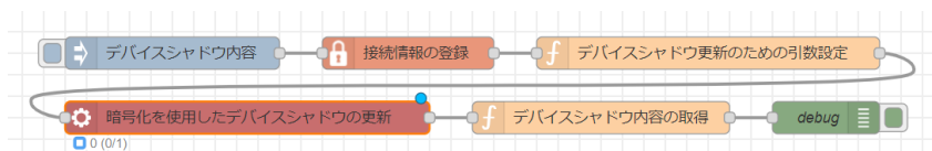
図 4.71 データの暗号化を使用したデバイスシャドウを更新するフロー
