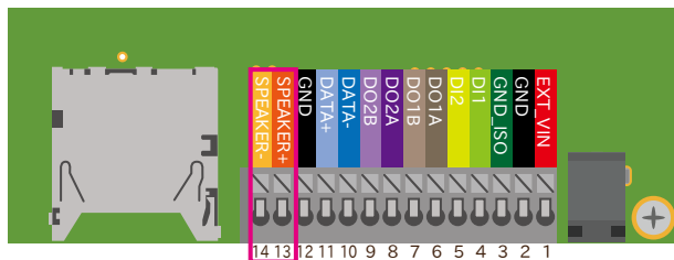
図 18.19 CON13D の配置
