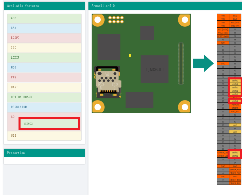
図 20.17 uSDHC2 の選択
