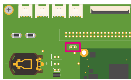
図 18.20 Armadillo-610 拡張ボード CON14
