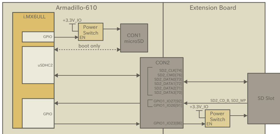
図 19.9 SD 接続例
