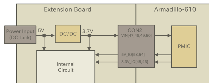
図 19.3 電源回路例
