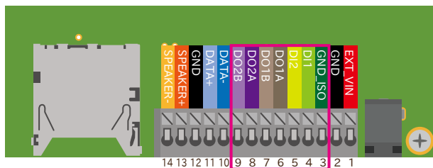
図 18.17 CON13B の配置
