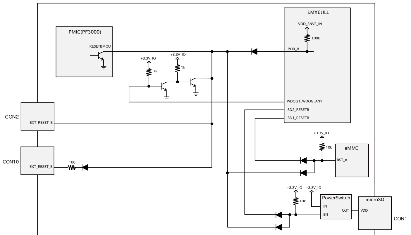
図 15.3 リセット回路の構成
