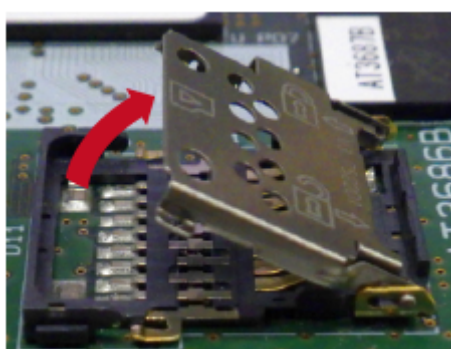
図 16.3 カバーを開ける
