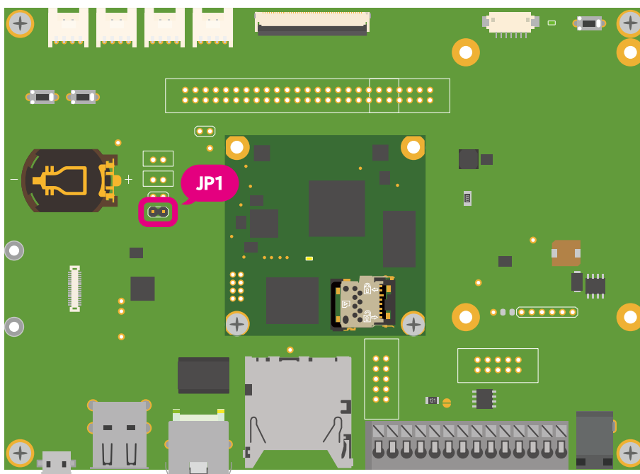
図 4.17 JP1 の位置
