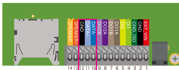
図 18.18 CON13C の配置
