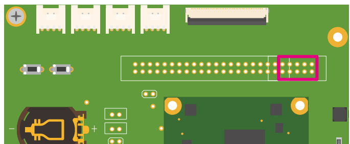
図 18.27 Armadillo-610 拡張ボード CON21
