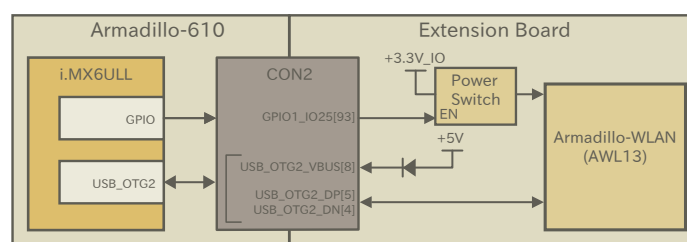
図 19.6 Armadillo-WLAN(AWL13)接続例
