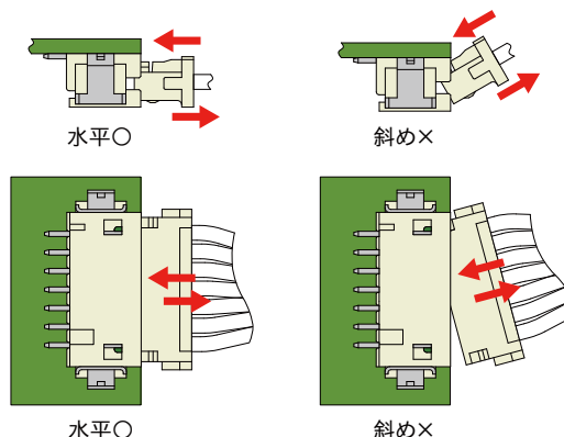
図 4.15 USB シリアル変換アダプタの挿抜角度
