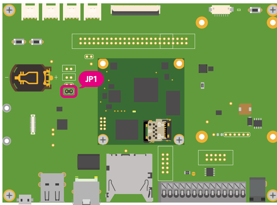
図 4.17 JP1 の位置
