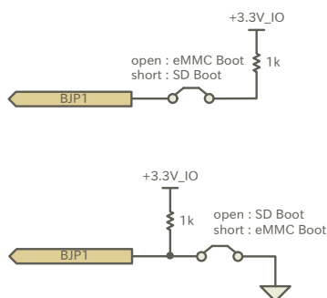
図 19.4 起動設定ジャンパー例
