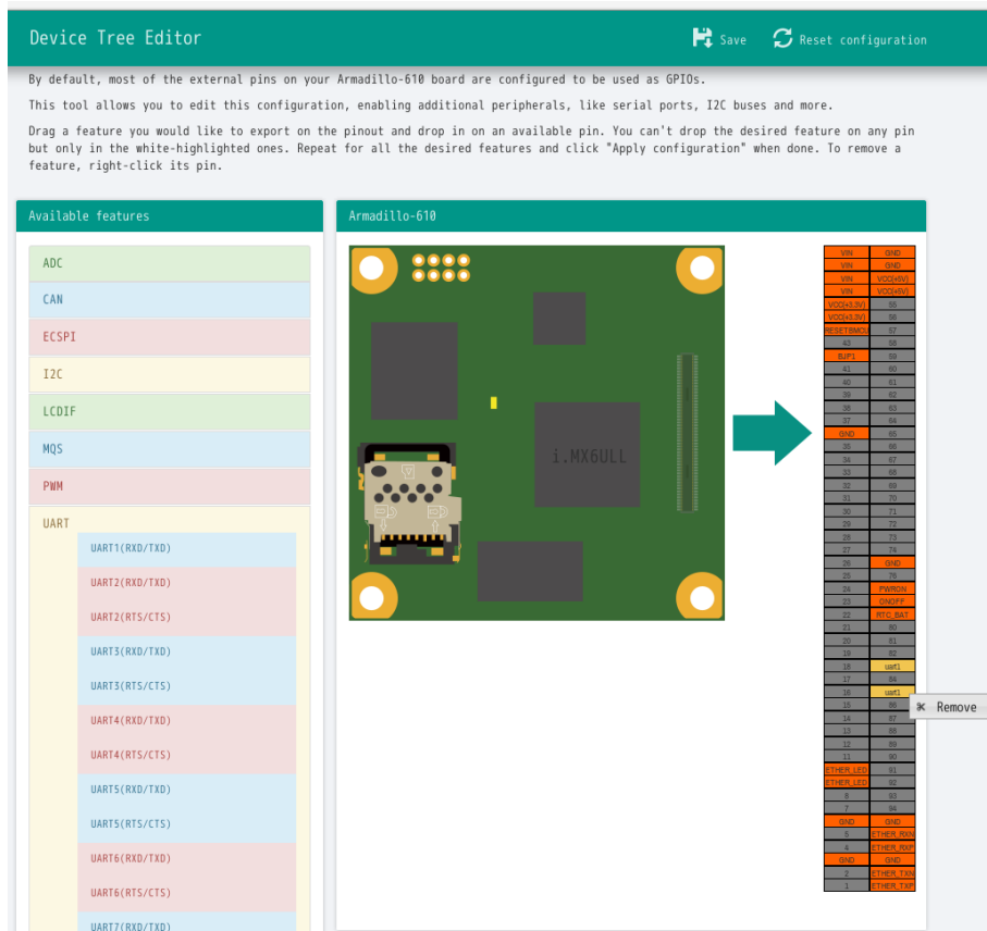
図 20.11 UART1(RXD/TXD)の削除
