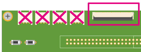
図 18.13 Armadillo-610 拡張ボード CON11
