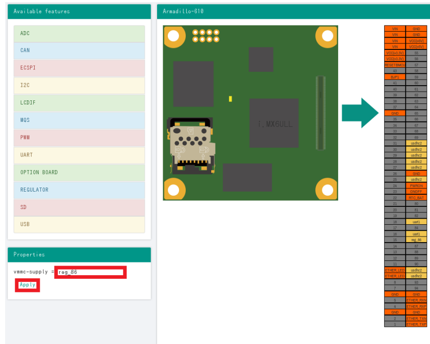
図 20.20 レギュレータの割り当て
