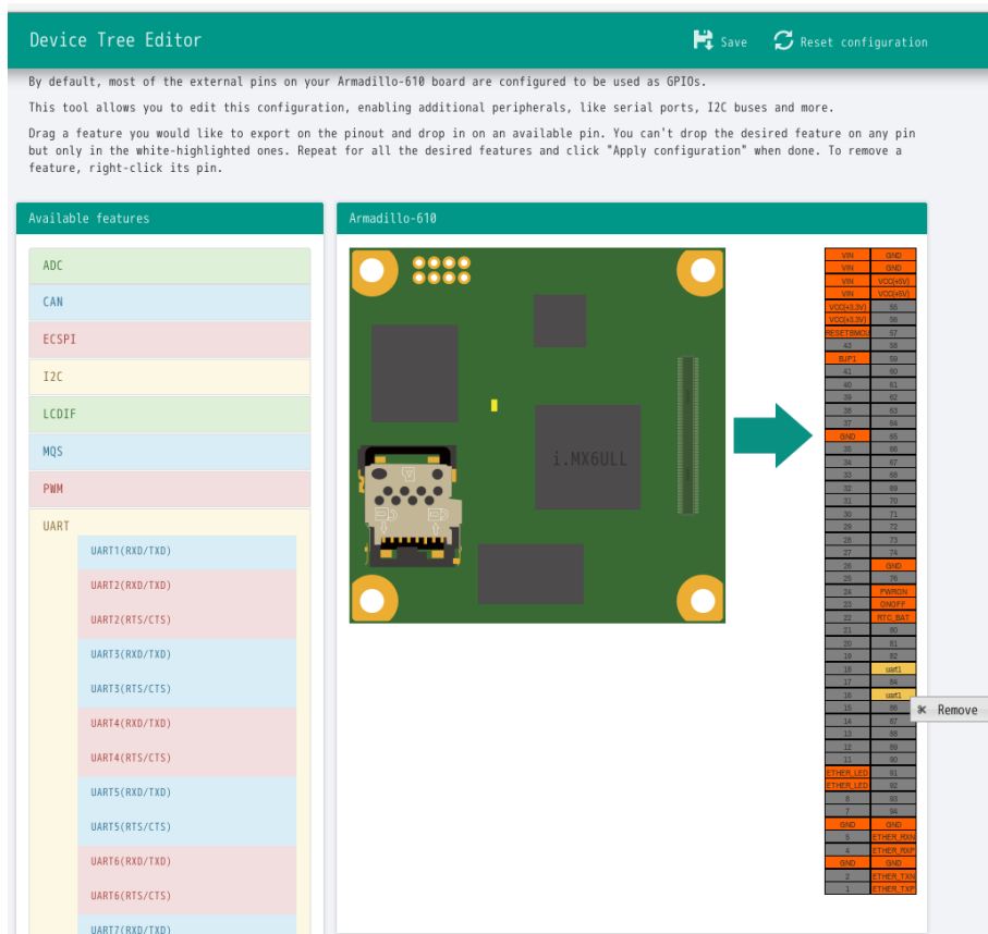
図 20.11 UART1(RXD/TXD)の削除
