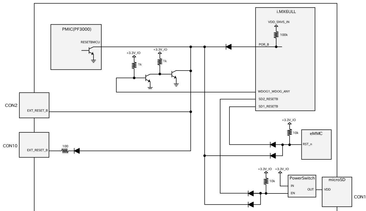
図 6.123 リセット回路の構成
