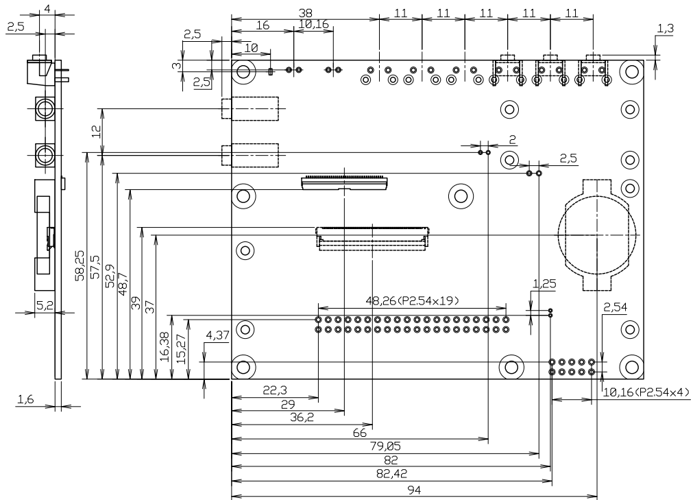
図 6.175 LCD 拡張ボードのコネクタ位置寸法
