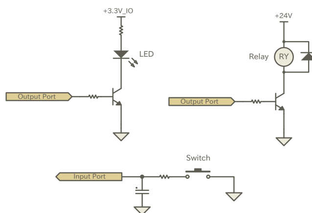
図 3.39 スイッチ、LED、リレー接続例
