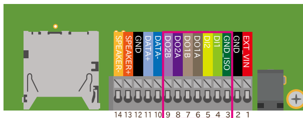
図 6.137 CON13B の配置
