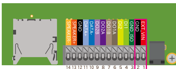
図 6.136 CON13A の配置
