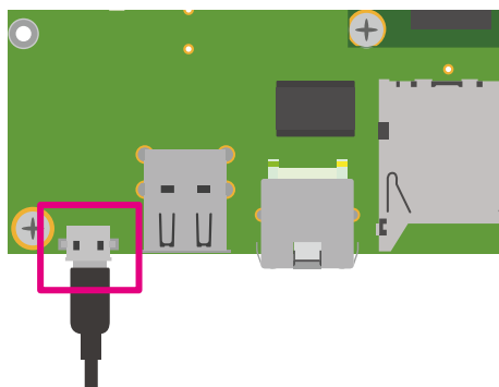
図 6.131 Armadillo-610 拡張ボード CON6
