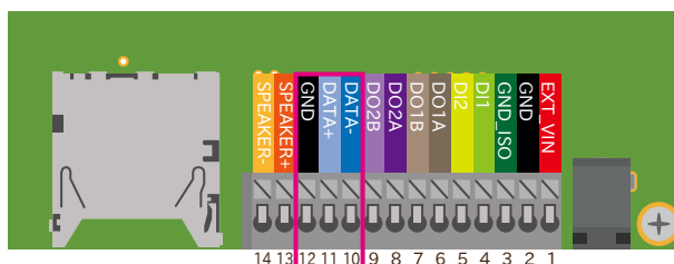
図 6.138 CON13C の配置
