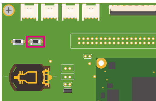
図 6.180 Armadillo-610 拡張ボード SW3
