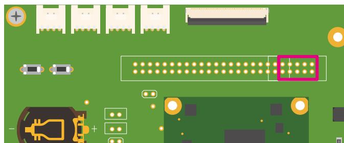
図 6.173 Armadillo-610 拡張ボード CON21
