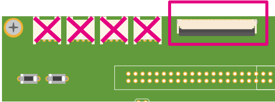
図 6.159 Armadillo-610 拡張ボード CON11
