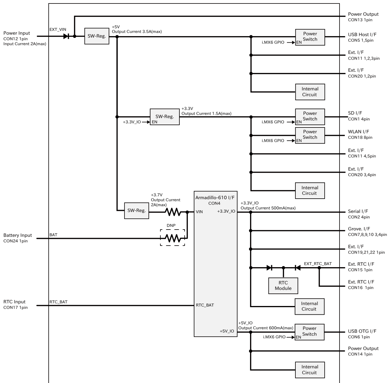
図 6.149 Armadillo-610 拡張ボードの電源回路の構成
