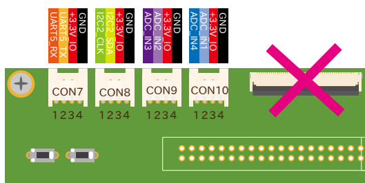
図 6.158 Armadillo-610 拡張ボード CON7、CON8、CON9、CON10
