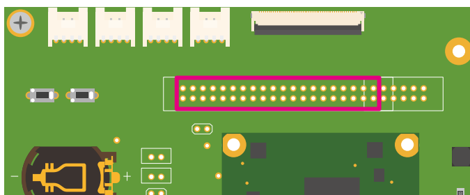
図 6.172 Armadillo-610 拡張ボード CON20
