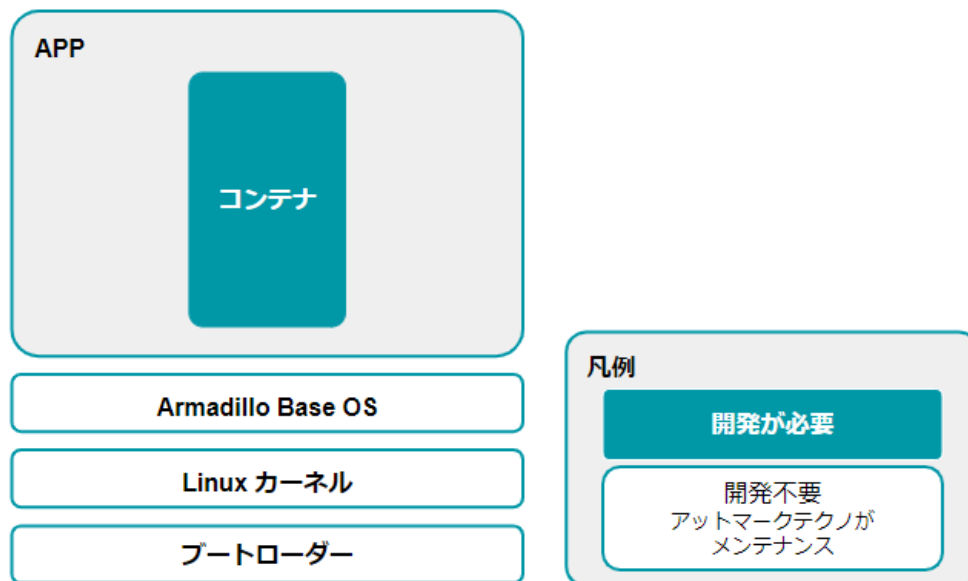
図 3.135 開発者が開発するもの、開発しなくていいもの
