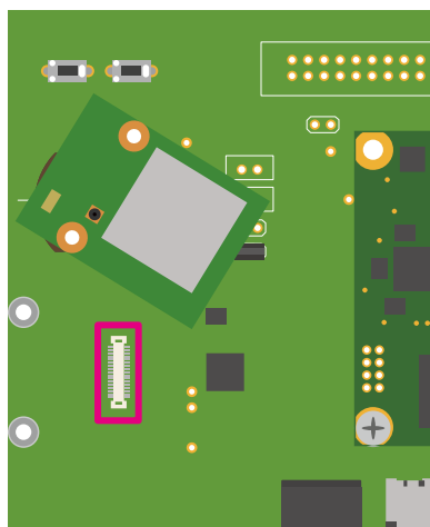
図 6.171 Armadillo-610 拡張ボード CON18
