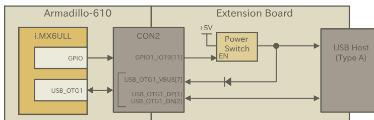
図 3.59 USB Host 接続例
