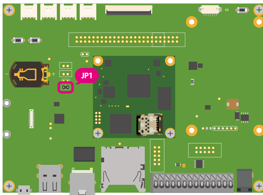
図 3.8 ジャンパピンの位置
