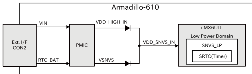
図 6.170 バックアップ電源供給回路
