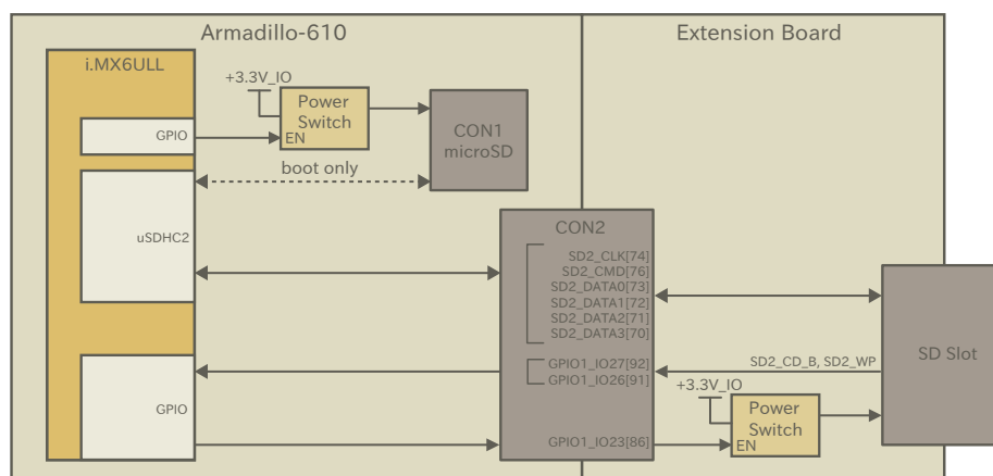
図 3.61 SD 接続例
