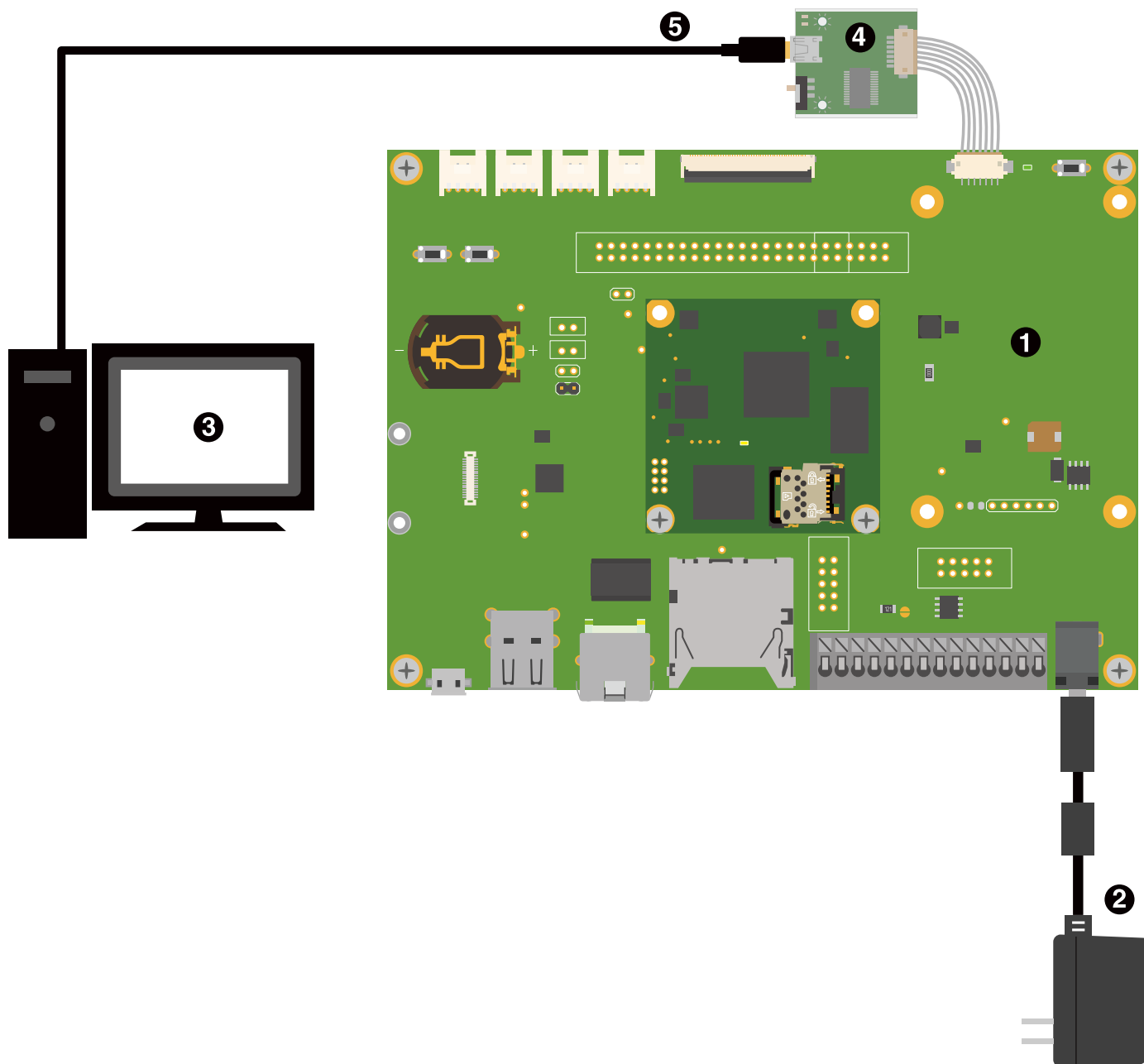
図 3.43 シリアルコンソールを使用する配線例
