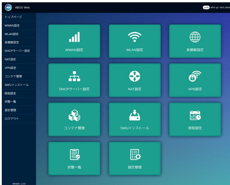
図 3.18 トップページ
