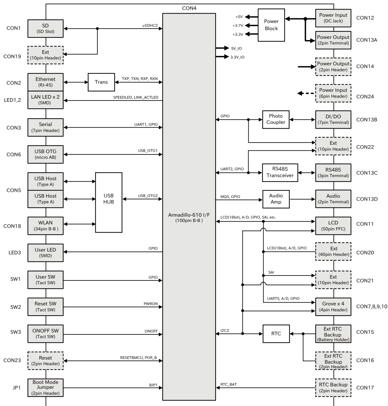
図 6.149 Armadillo-610 拡張ボードのブロック図
