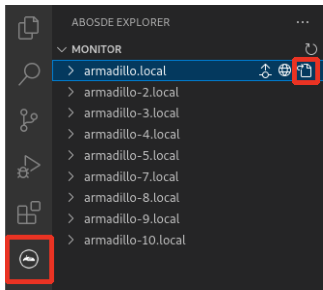
図 3.29 ABOSDE を使用して ssh 接続に使用する IP アドレスを設定する
