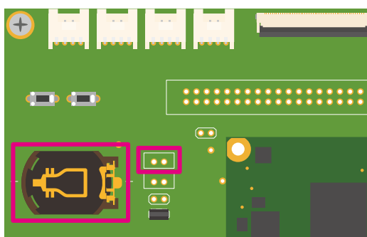
図 6.168 Armadillo-610 拡張ボード CON15、CON16
