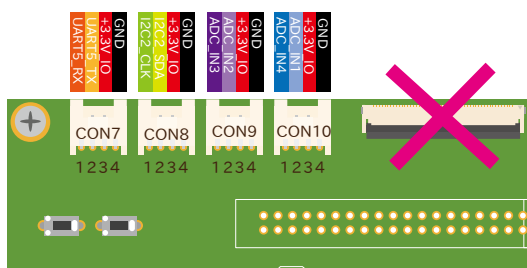
図 6.159 Armadillo-610 拡張ボード CON7、CON8、CON9、CON10
