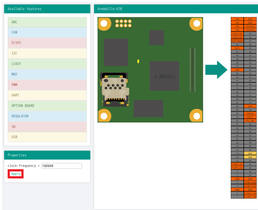
図 3.84 プロパティの保存
