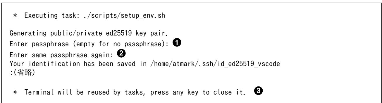
図 3.200 SSH 用の鍵を生成する
