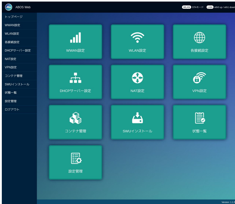
図 3.145 トップページ
