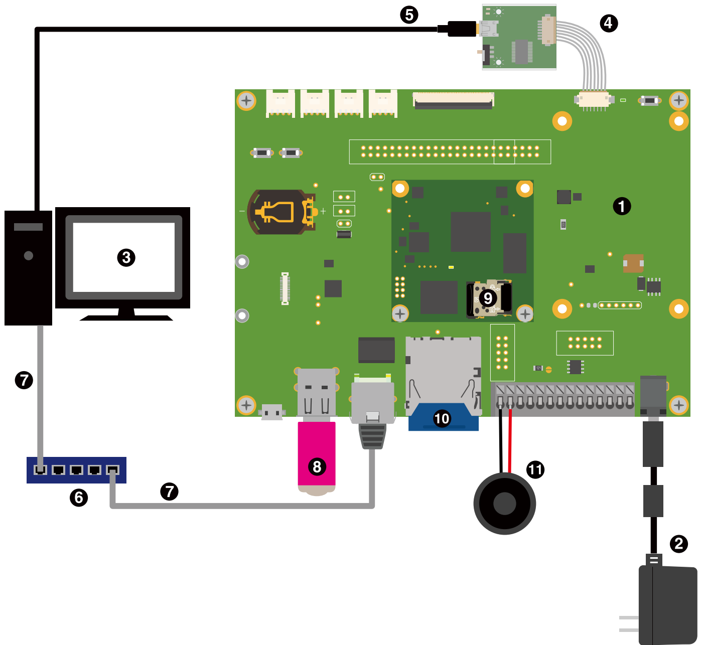
図 3.51 Armadillo-610 開発セットの接続例
