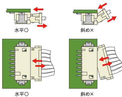
図 3.42 USB シリアル変換アダプタの挿抜角度
