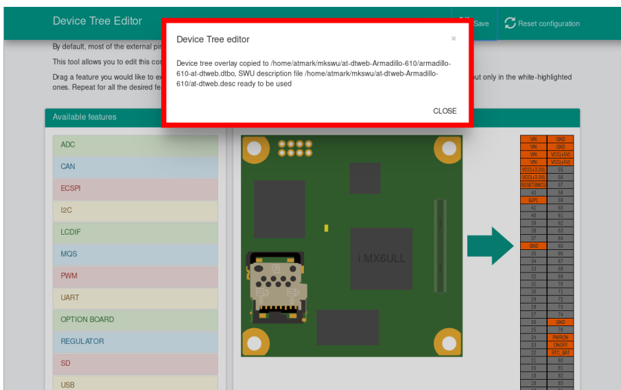
図 3.88 dtbo/desc の生成完了
