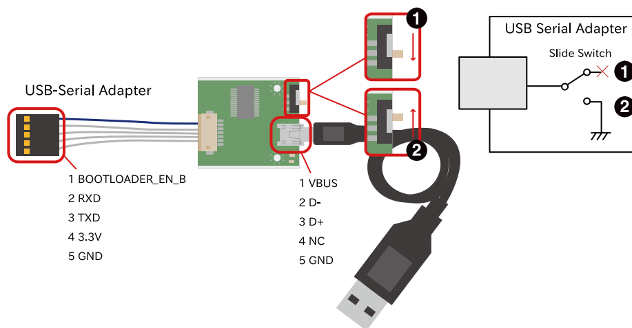
図 6.148 USB シリアル変換アダプタの配線
