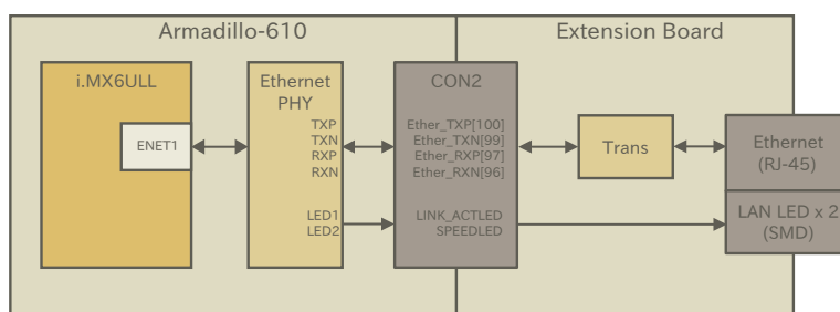
図 3.57 LAN(Ethernet)接続例
