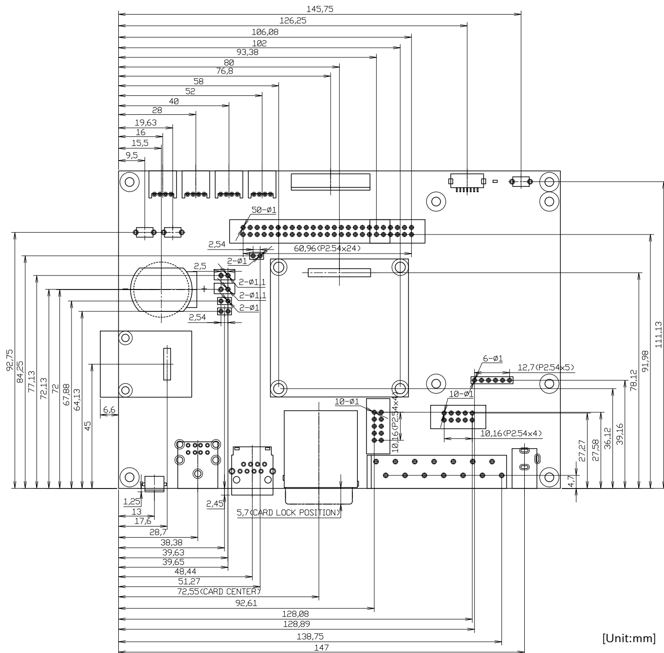
図 6.185 Armadillo-610 拡張ボード コネクタ中心寸法および穴寸法
