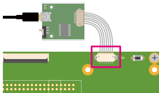
図 6.155 Armadillo-610 拡張ボード CON3
