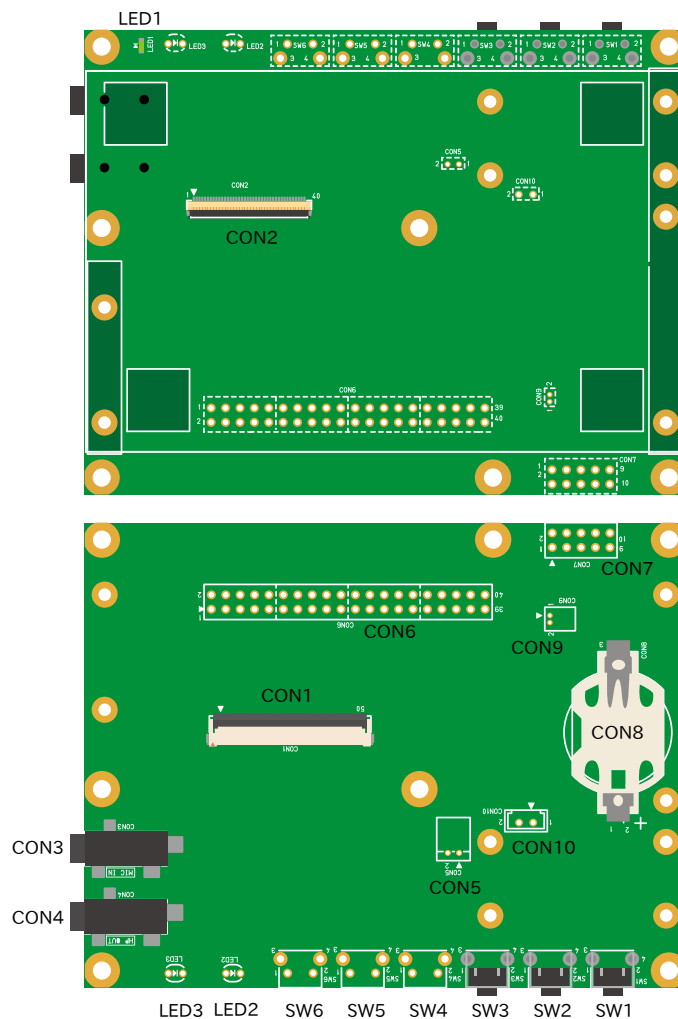
図 6.187 LCD 拡張ボードのインターフェース
