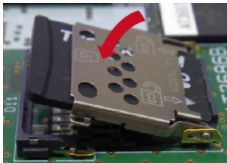
図 3.95 カバーを閉める
