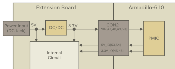
図 3.55 電源回路例
