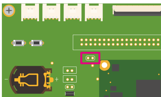
図 6.167 Armadillo-610 拡張ボード CON14
