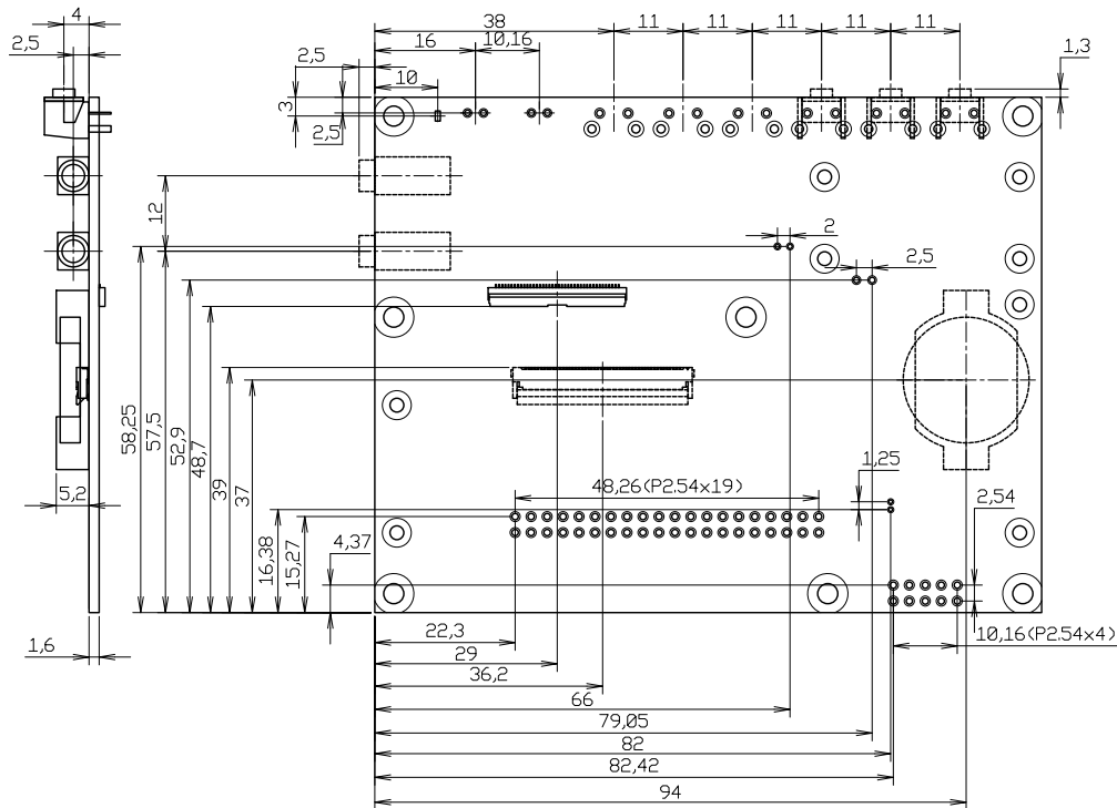
図 6.194 LCD 拡張ボードのコネクタ位置寸法
