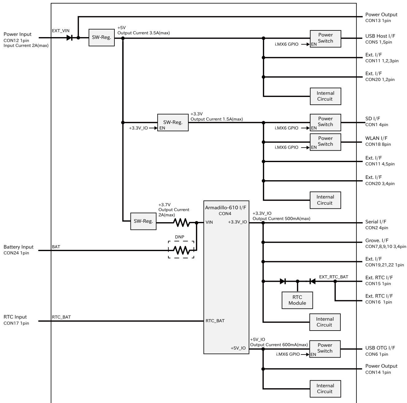
図 6.150 Armadillo-610 拡張ボードの電源回路の構成
