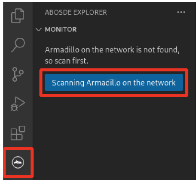
図 3.12 ABOSDE で ローカルネットワーク上の Armadillo をスキャンする
