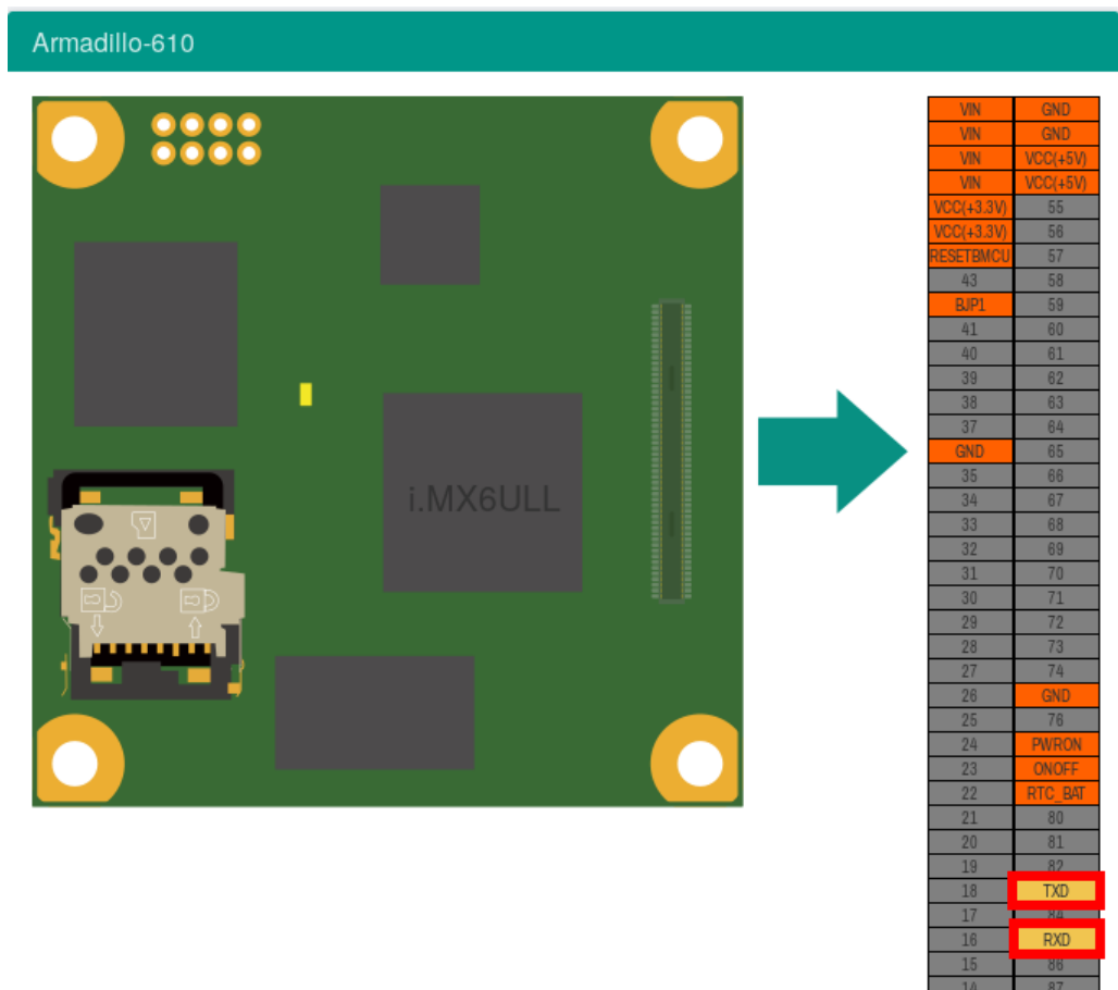
図 3.82 信号名の確認
