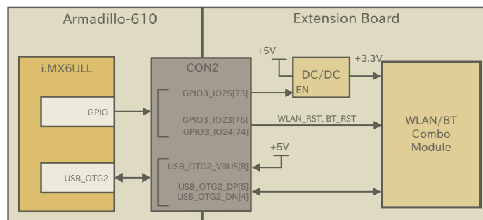
図 3.58 WLAN/BT 接続例
