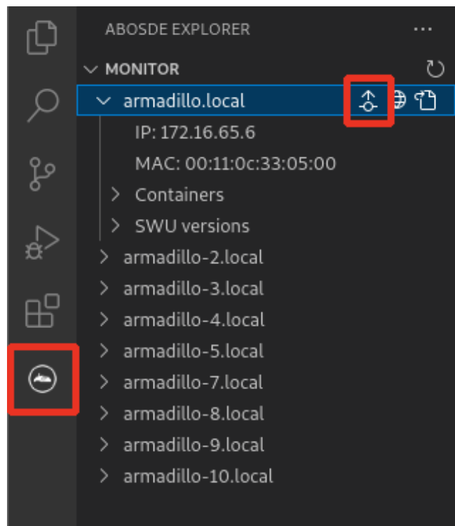
図 3.28 ABOSDE で Armadillo に SWU をインストール
