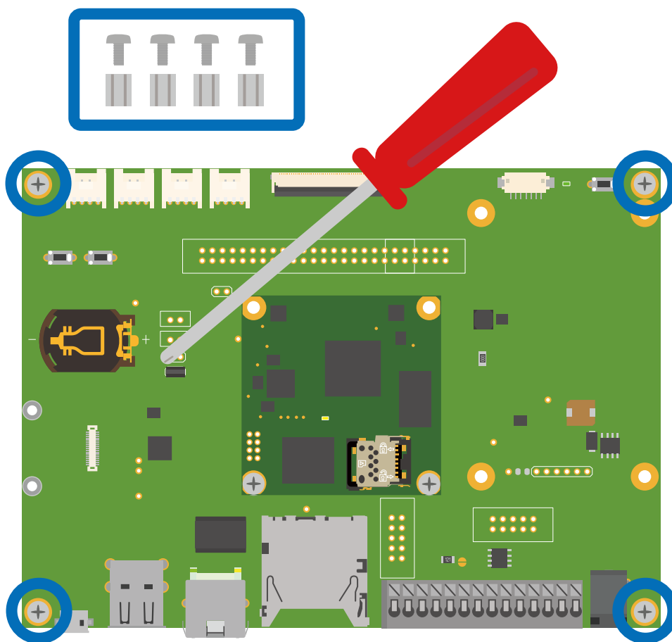
図 3.6 Armadillo-610 開発セットの組み立て
