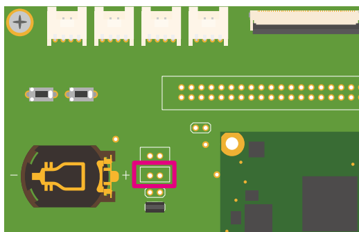
図 6.169 Armadillo-610 拡張ボード CON17
