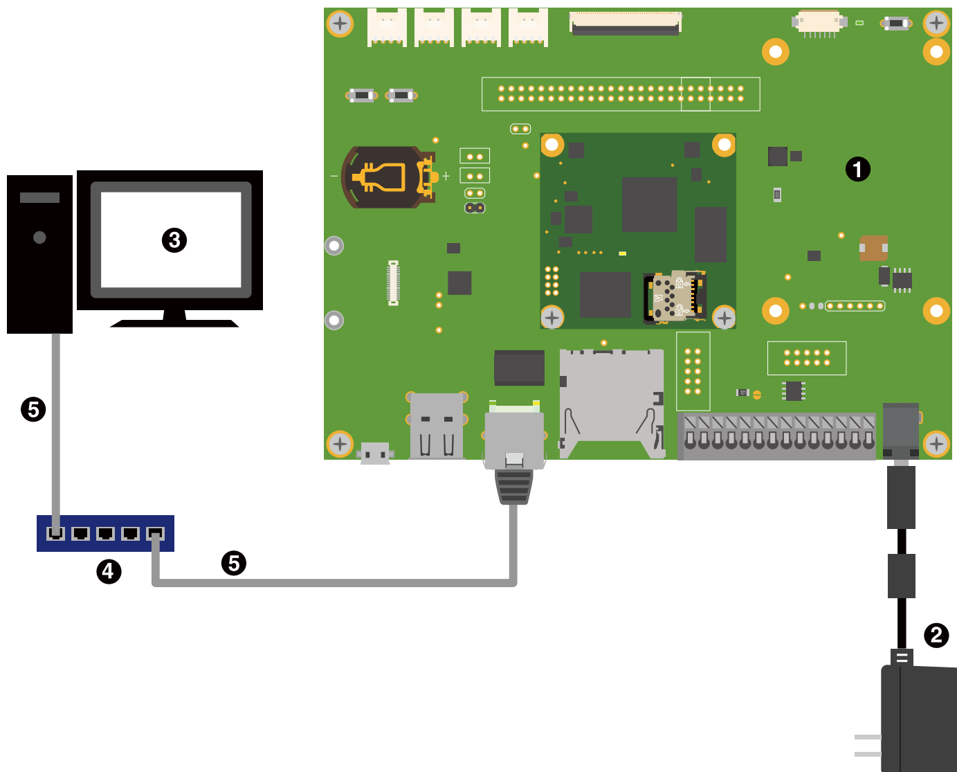
図 3.11 ABOS にアクセスするための接続
