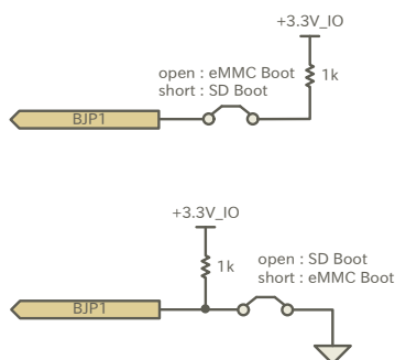
図 3.56 起動設定ジャンパー例
