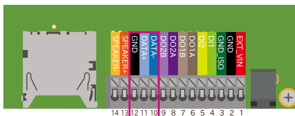
図 6.165 CON13C の配置
