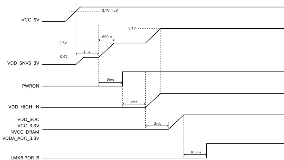
図 3.69 電源シーケンス [6]
