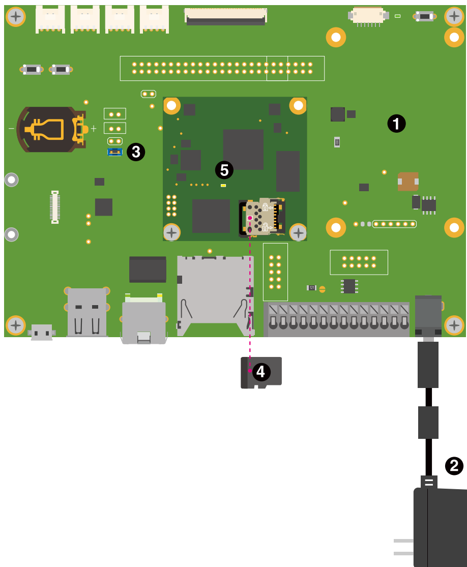
図 3.7 Armadillo-610 を初期化する接続
