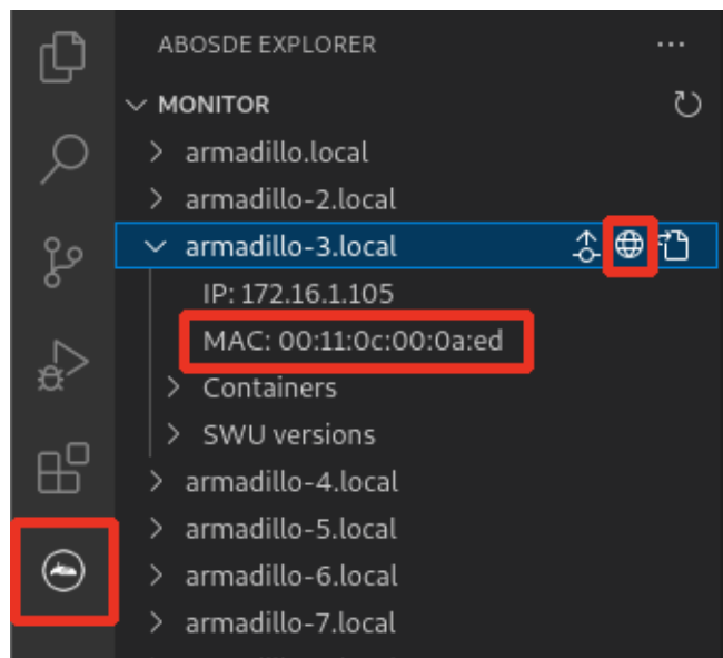
図 3.14 ABOSDE を使用して ABOS Web を開く
