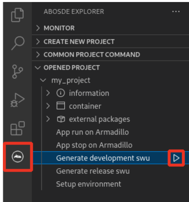
図 3.26 VSCode でコンテナイメージの作成を行う
