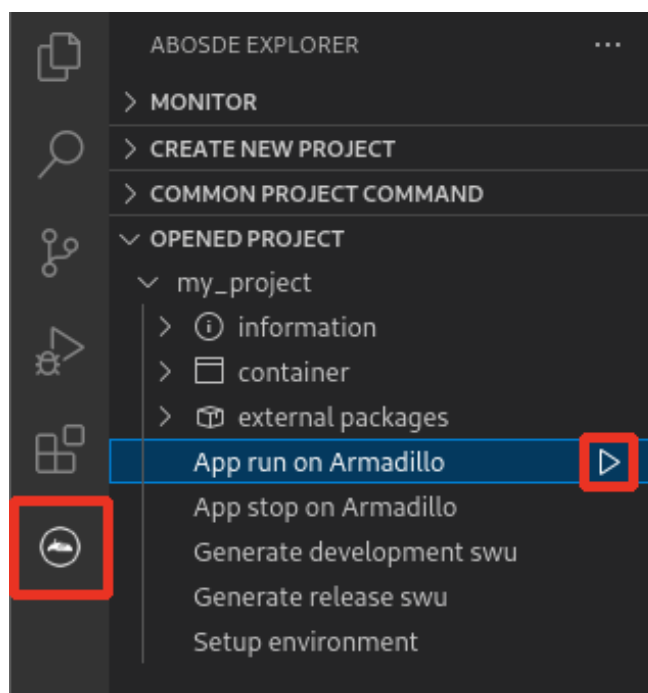
図 3.31 Armadillo 上でアプリケーションを実行する
