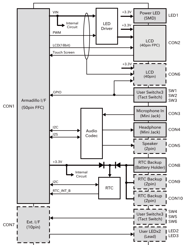
図 6.198 LCD 拡張ボードのブロック図
