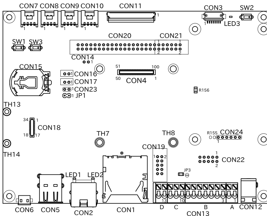
図 6.163 Armadillo-610 拡張ボードのインターフェースの概要
