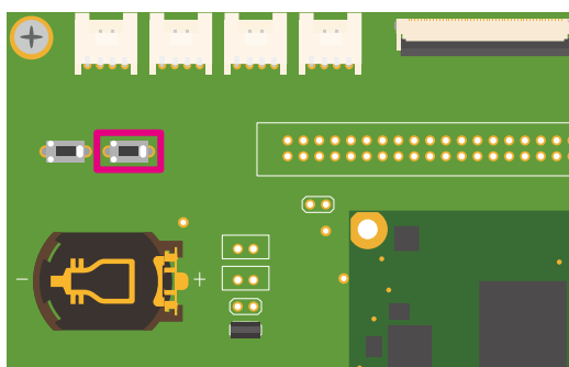
図 6.193 Armadillo-610 拡張ボード SW3
