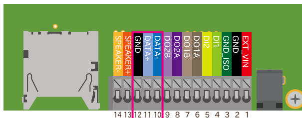
図 6.177 CON13C の配置
