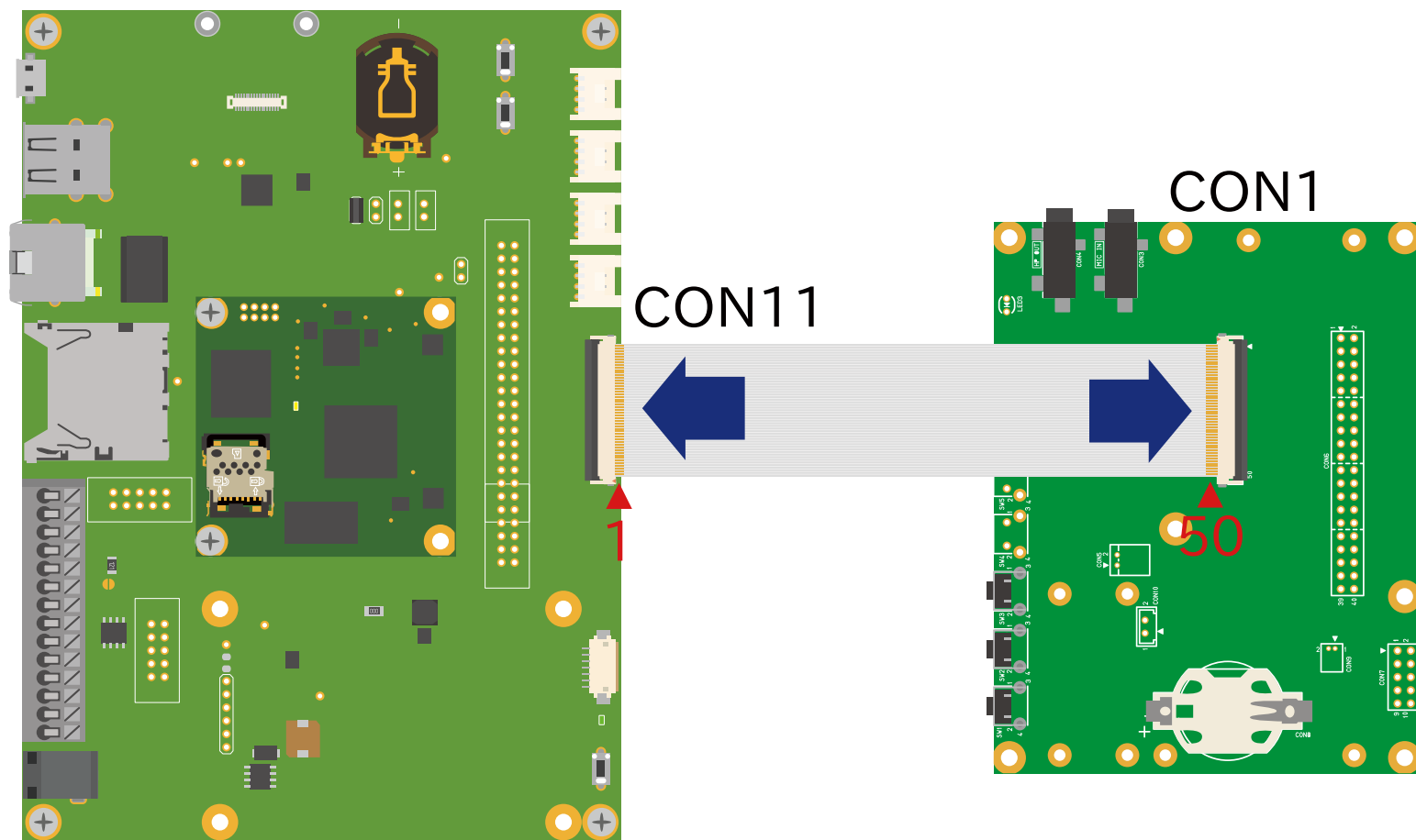
図 6.202 Armadillo-610 と LCD 拡張ボードの接続
