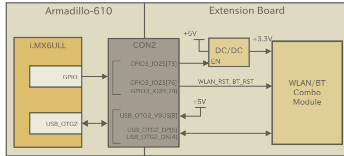
図 3.57 WLAN/BT 接続例
