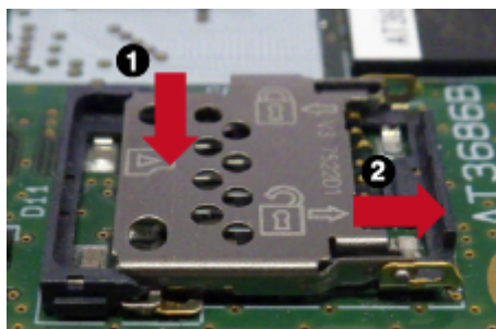
図 3.90 カバーのロックを解除する
