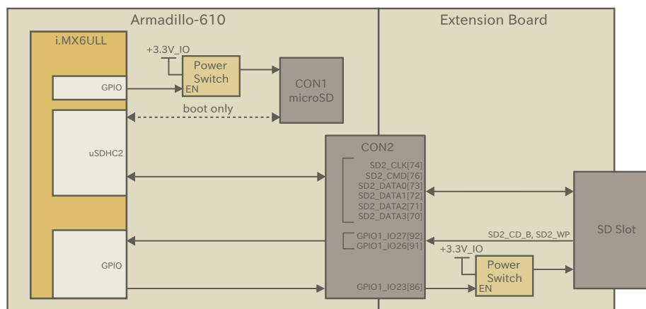
図 3.60 SD 接続例
