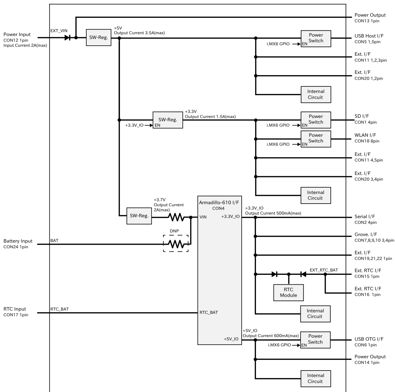
図 6.167 Armadillo-610 拡張ボードの電源回路の構成
