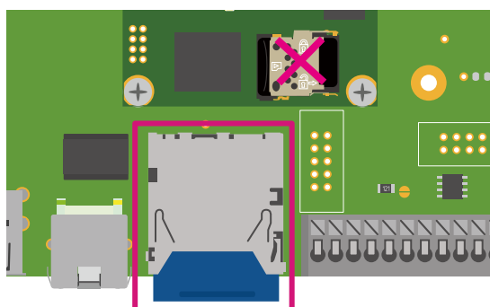
図 6.169 Armadillo-610 拡張ボード CON1
