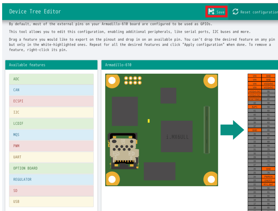
図 3.86 DTS/DTB の生成
