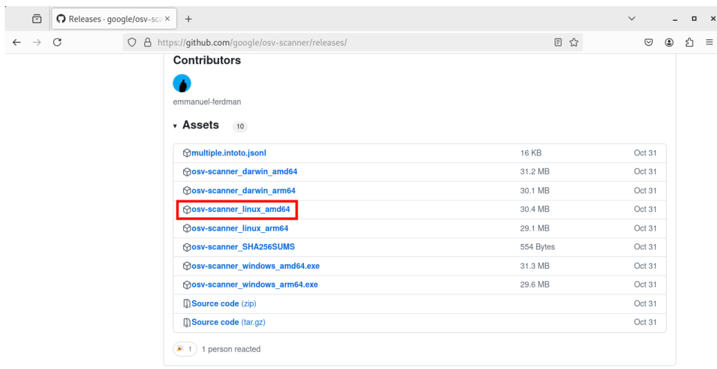
図 3.231 OSV-Scanner の実行ファイルをダウンロード
