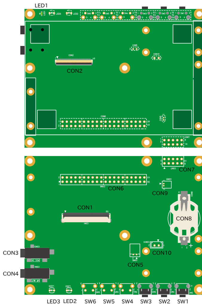
図 6.204 LCD 拡張ボードのインターフェース
