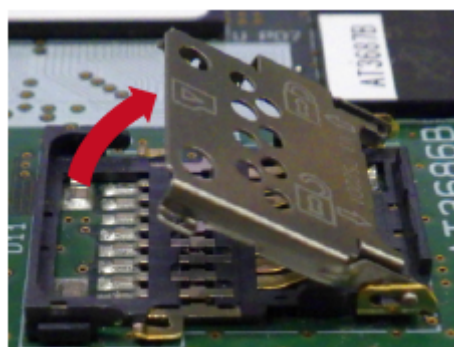
図 3.91 カバーを開ける
