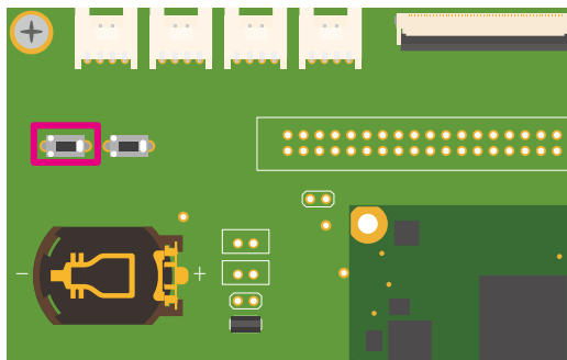
図 6.196 Armadillo-610 拡張ボード SW1
