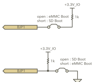
図 3.55 起動設定ジャンパー例
