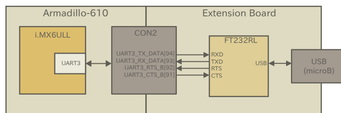
図 3.59 シリアル(UART)接続例
