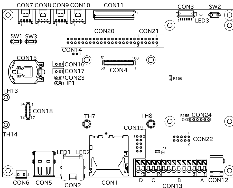
図 6.168 Armadillo-610 拡張ボードのインターフェースの概要
