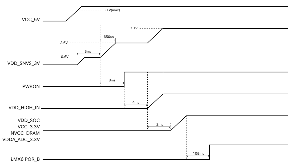
図 3.68 電源シーケンス [6]
