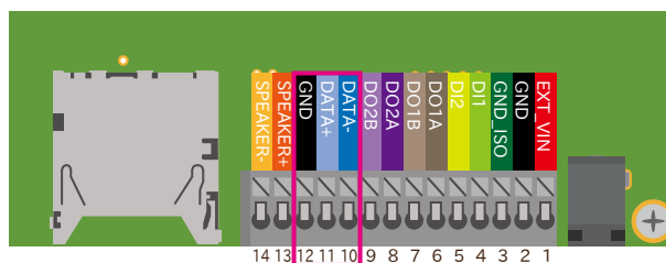
図 6.193 CON13C の配置
