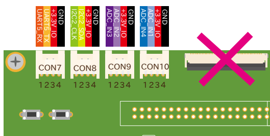
図 6.187 Armadillo-610 拡張ボード CON7、CON8、CON9、CON10
