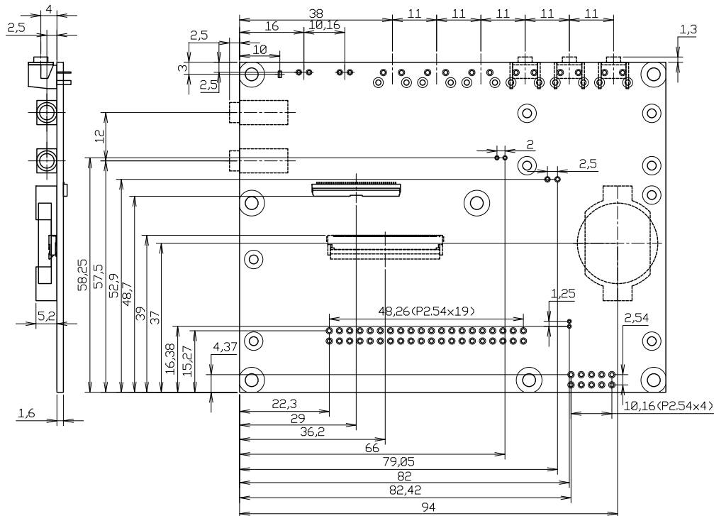
図 6.167 LCD 拡張ボードのコネクタ位置寸法
