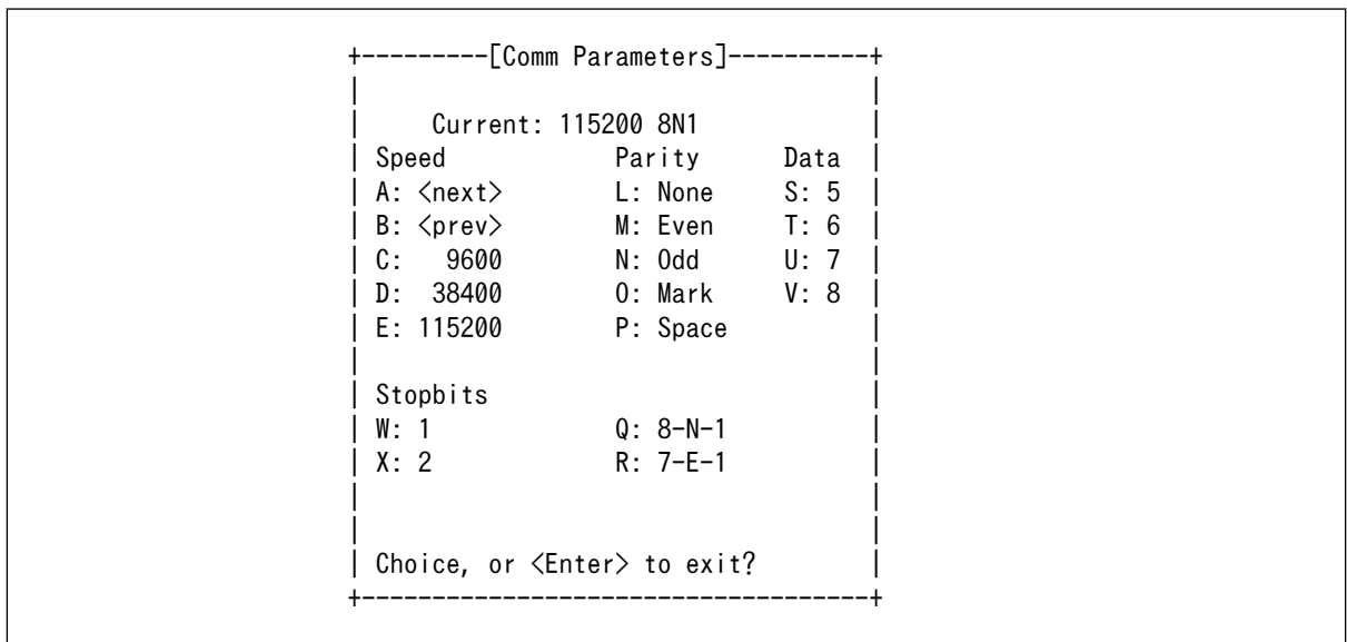
図 3.11 minicom のシリアルポートのパラメータの設定
