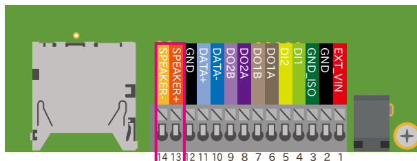
図 6.139 CON13D の配置
