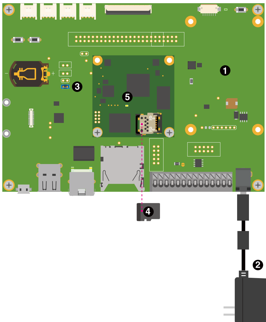
図 3.20 Armadillo-610 を初期化する接続
