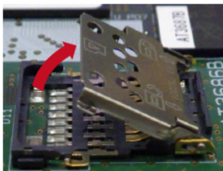
図 3.97 カバーを開ける
