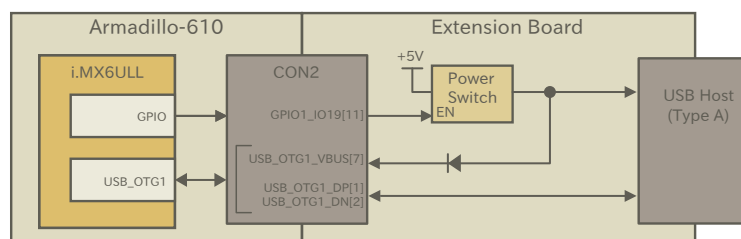
図 3.64 USB Host 接続例
