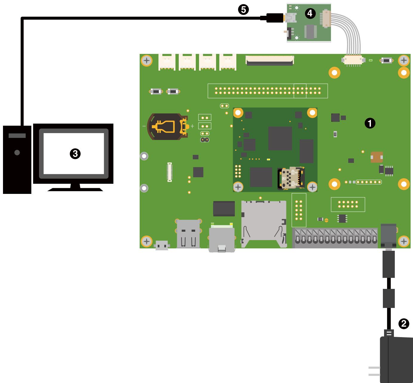
図 3.50 シリアルコンソールを使用する配線例
