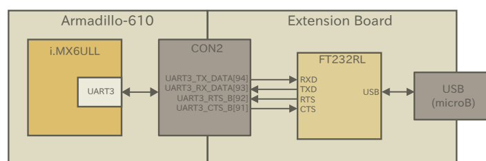
図 3.65 シリアル(UART)接続例
