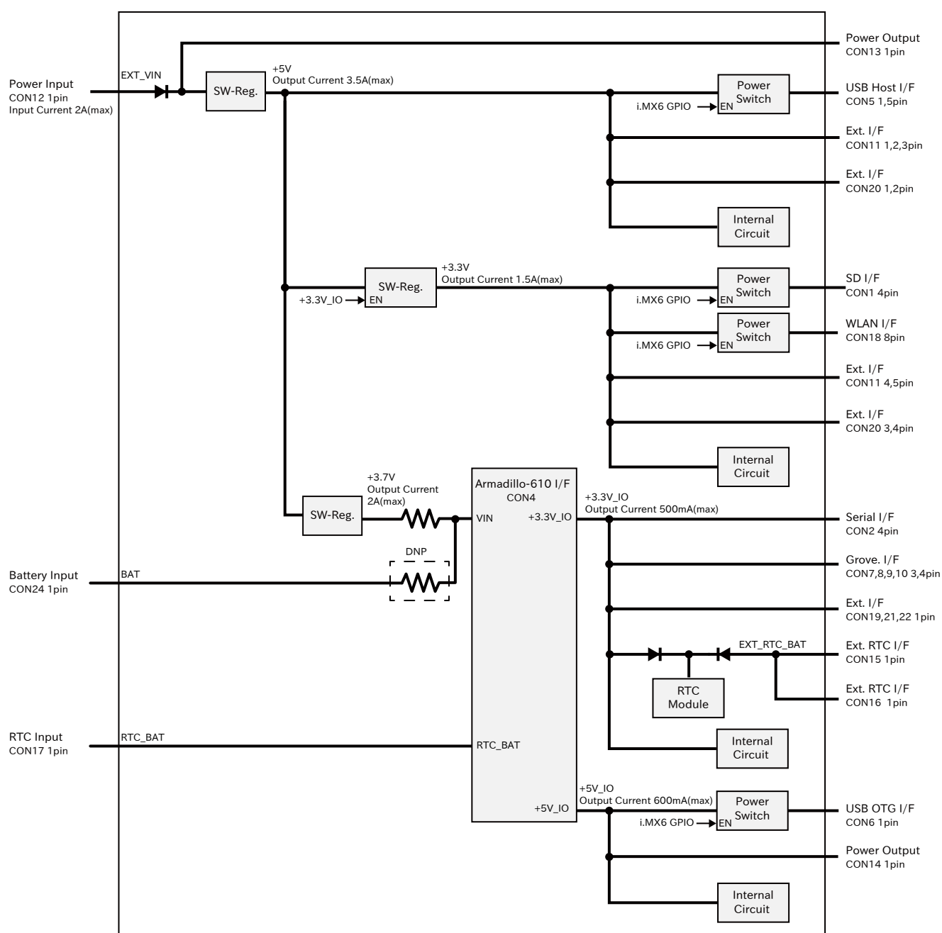
図 6.177 Armadillo-610 拡張ボードの電源回路の構成
