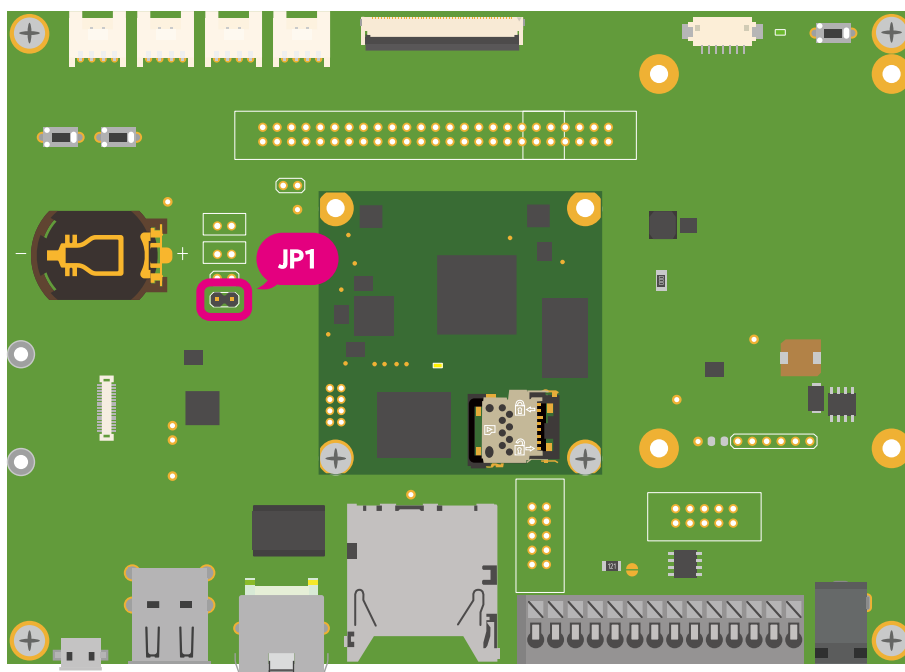
図 3.21 ジャンパピンの位置
