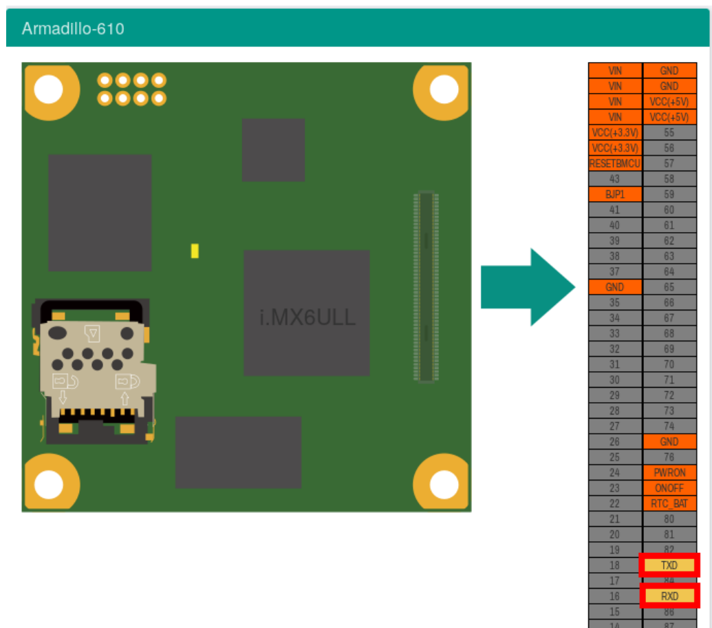
図 3.87 信号名の確認
