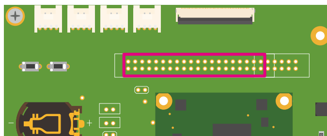
図 6.201 Armadillo-610 拡張ボード CON20
