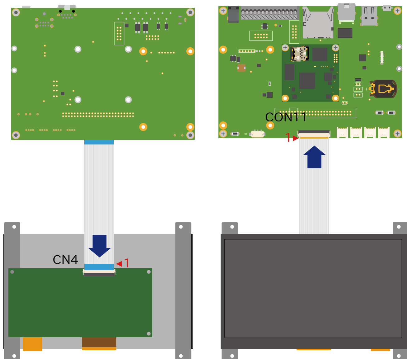
図 3.126 LCD の接続方法
