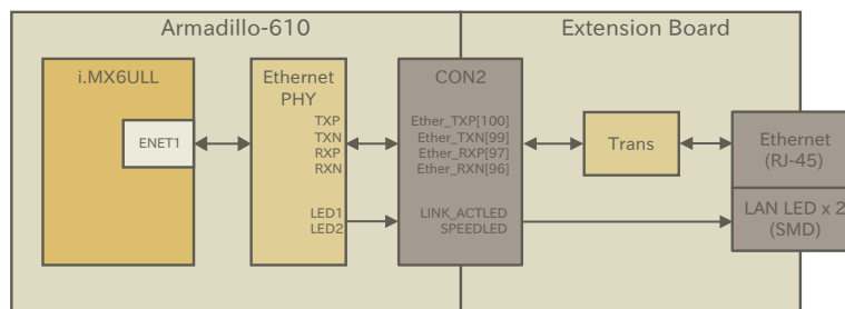
図 3.62 LAN(Ethernet)接続例
