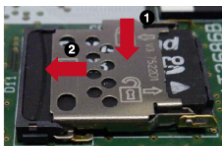
図 3.101 カバーをロックする
