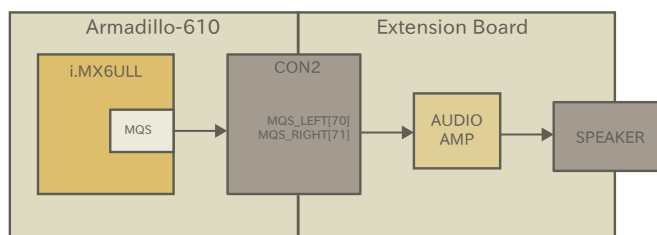
図 3.68 MQS 接続例
