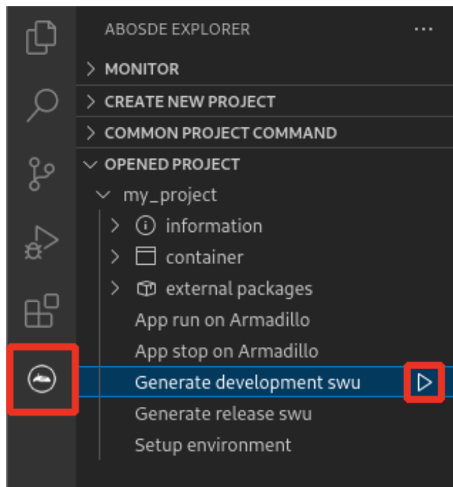
図 3.39 VS Code でコンテナイメージの作成を行う
