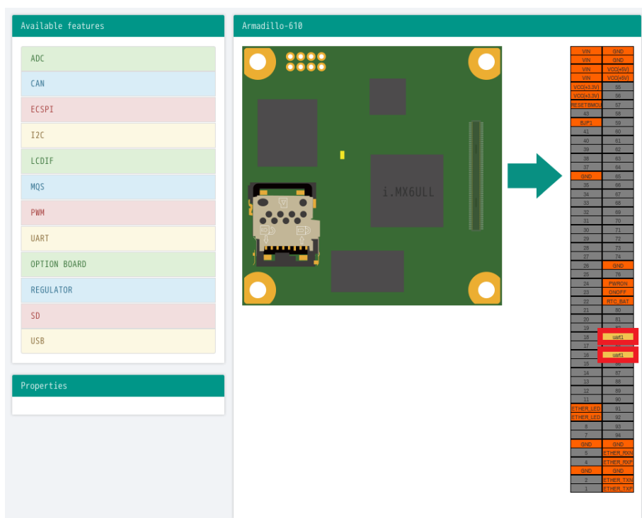
図 3.86 CON2 83/85 ピンへのドロップ
