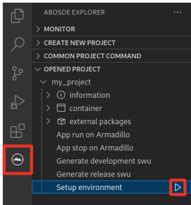
図 3.36 VS Code で初期設定を行う
