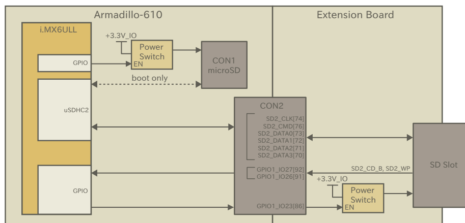
図 3.66 SD 接続例
