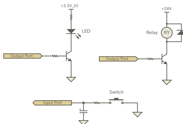
図 3.67 スイッチ、LED、リレー接続例
