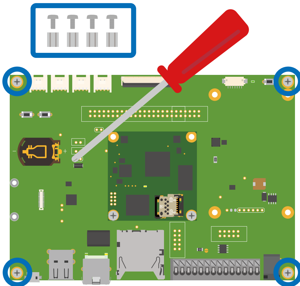
図 3.19 Armadillo-610 開発セットの組み立て
