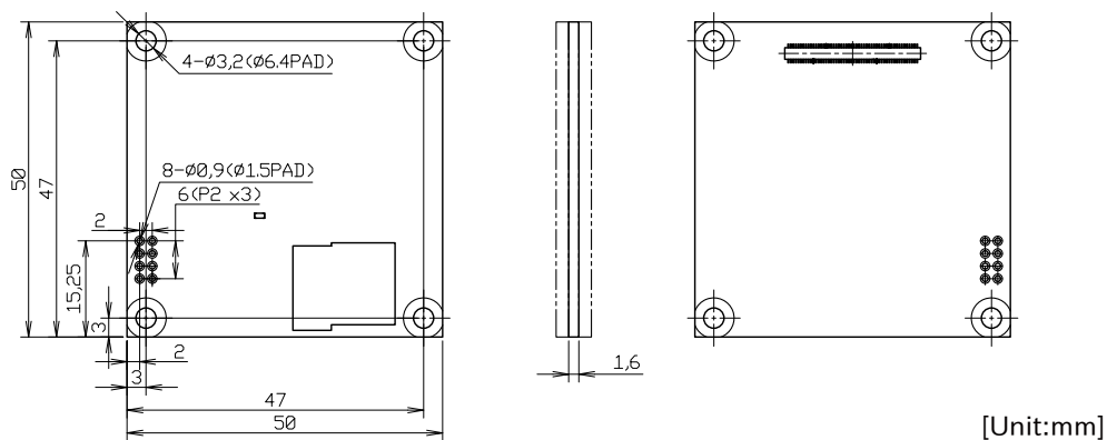
図 3.78 基板形状および固定穴寸法
