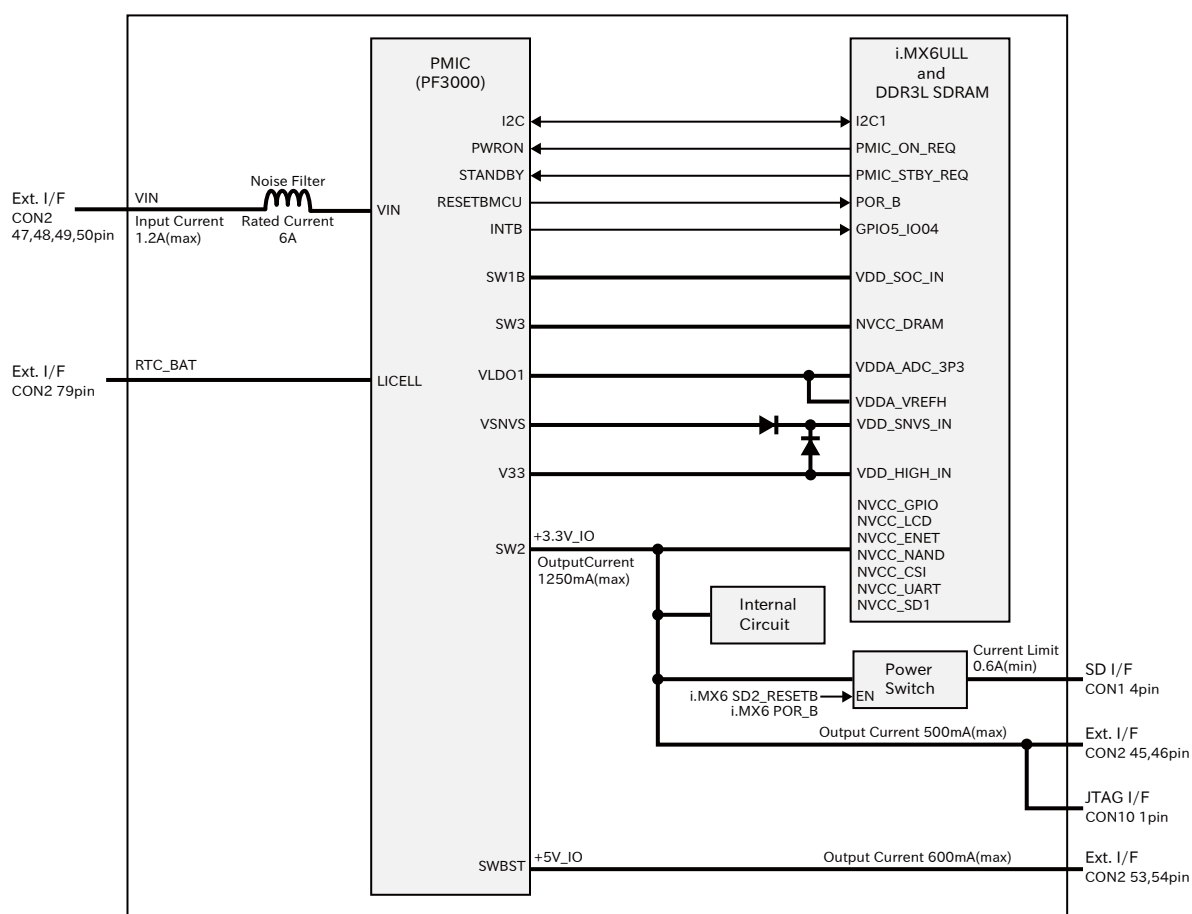
図 3.73 電源回路の構成
