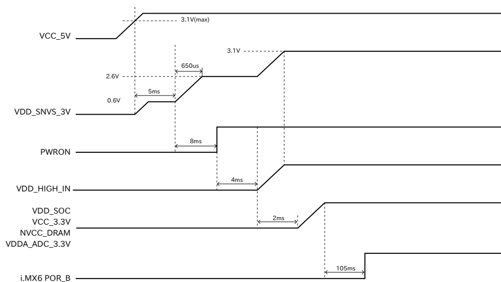
図 3.74 電源シーケンス [5]
