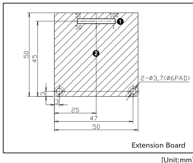
図 3.71 拡張ボード推奨レイアウト
