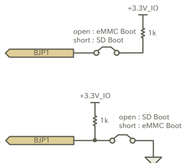
図 3.61 起動設定ジャンパー例
