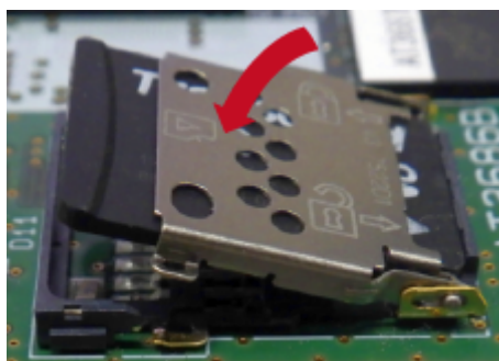
図 3.100 カバーを閉める
