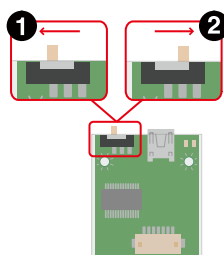
図 3.48 スライドスイッチの設定
