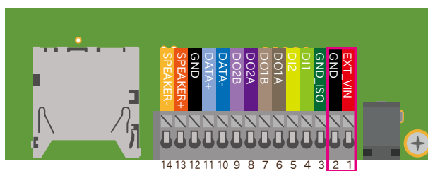
図 6.190 CON13A の配置
