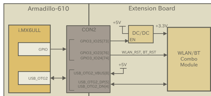
図 3.63 WLAN/BT 接続例
