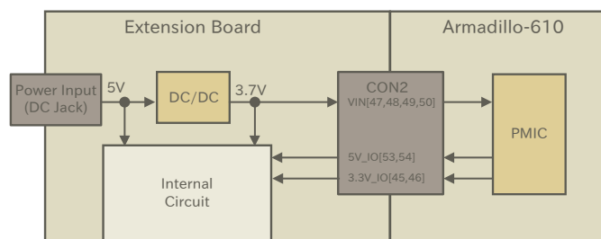
図 3.60 電源回路例
