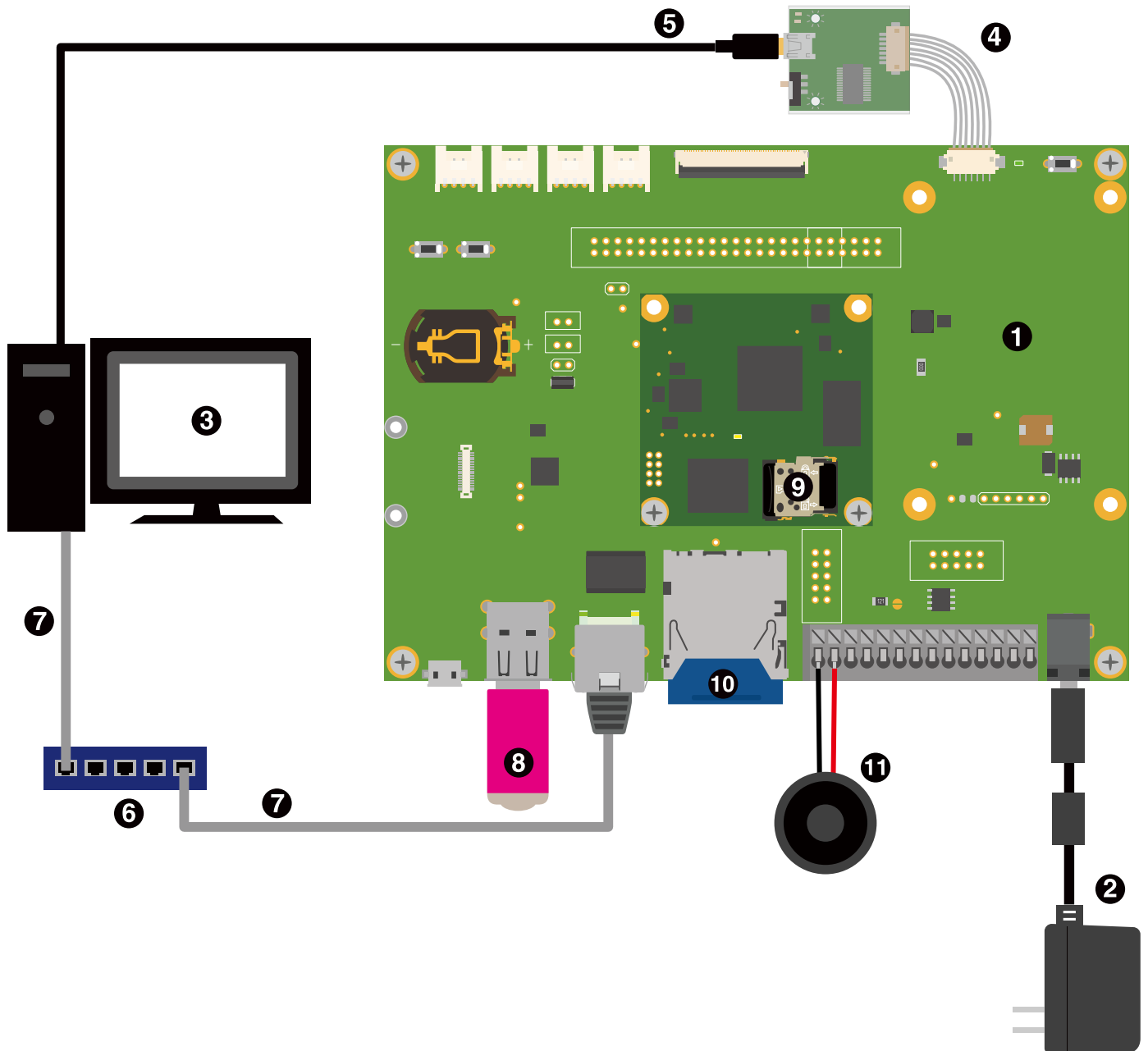
図 3.15 Armadillo-610 開発セットの接続例
