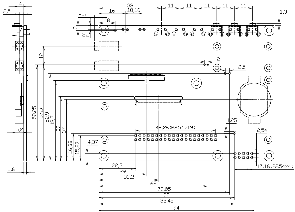
図 6.170 LCD 拡張ボードのコンネクタ位置寸法
