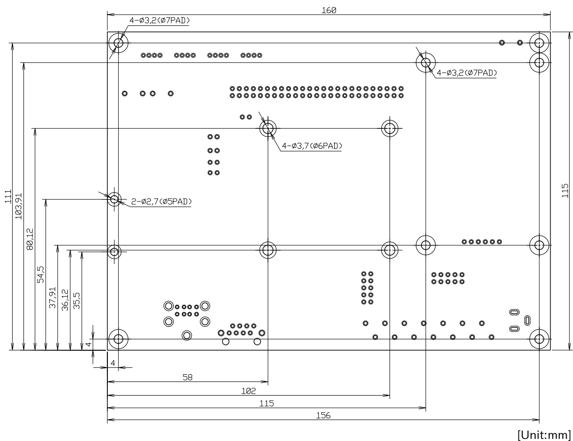
図 6.160 Armadillo-610 拡張ボード 基板形状および固定穴寸法
