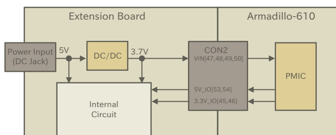
図 3.29 電源回路例
