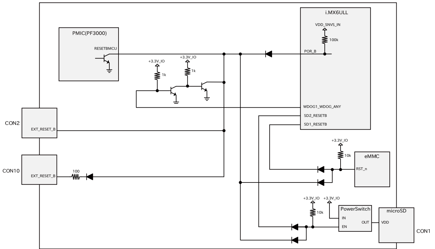
図 3.44 リセット回路の構成
