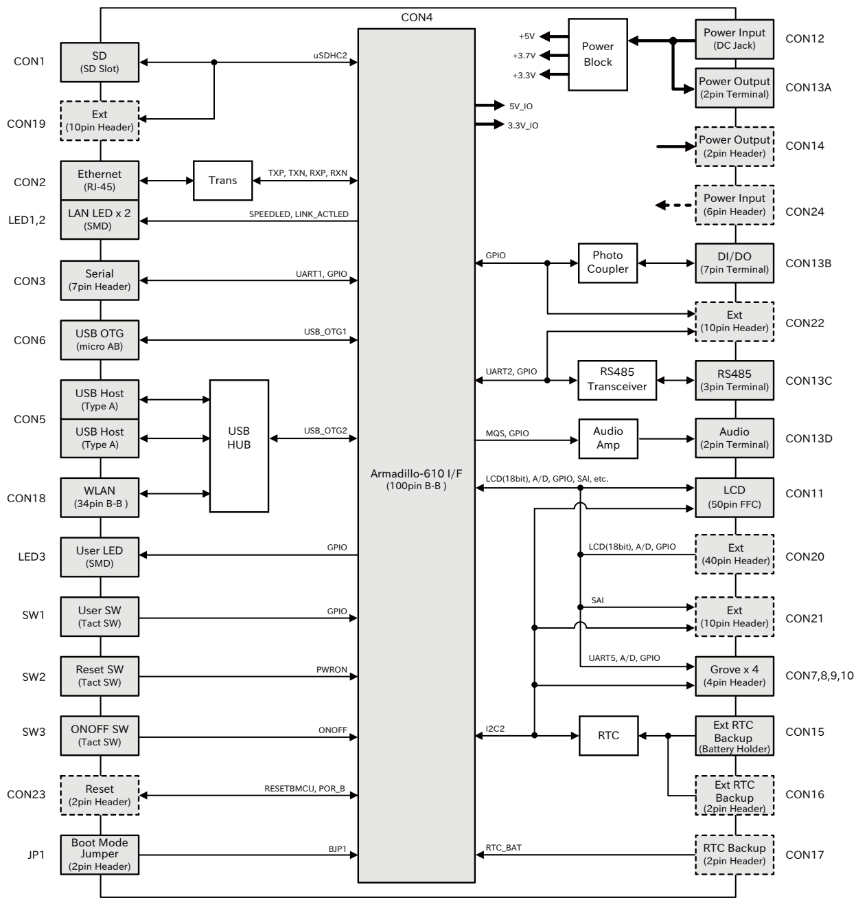
図 6.137 Armadillo-610 拡張ボードのブロック図
