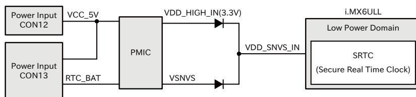
図 16.6 バックアップ電源供給
