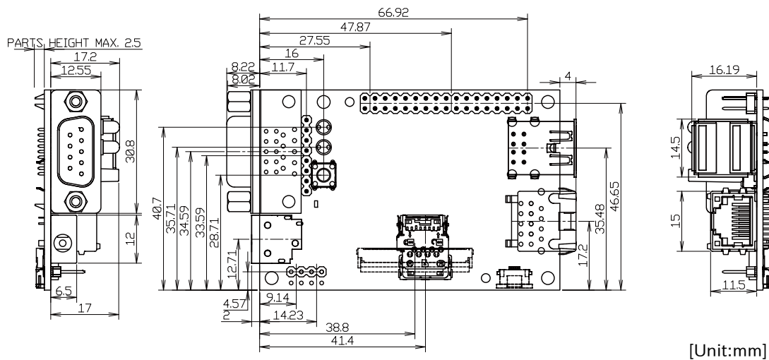
図 3.28 コネクタ中心寸法
