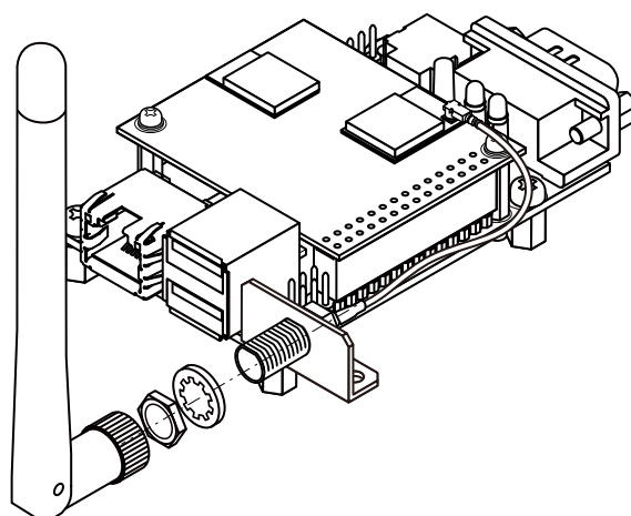
図 6.140 外付けアンテナの組み立て(OP-MNT-ANT-MET-00 使用)
