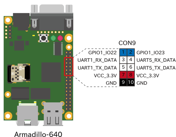
図 6.122 Armadillo-640 のシリアル信号線
