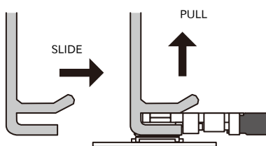
図 6.150 挿抜治具によるアンテナケーブルコネクタの抜去
