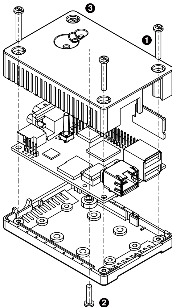
図 6.123 Armadillo-600 シリーズ オプションケース(樹脂製)の組み立て
