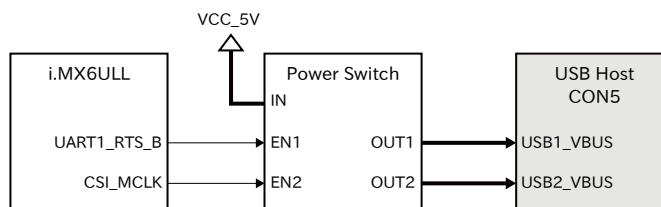
図 3.54 USB ホストインターフェースの電源制御
