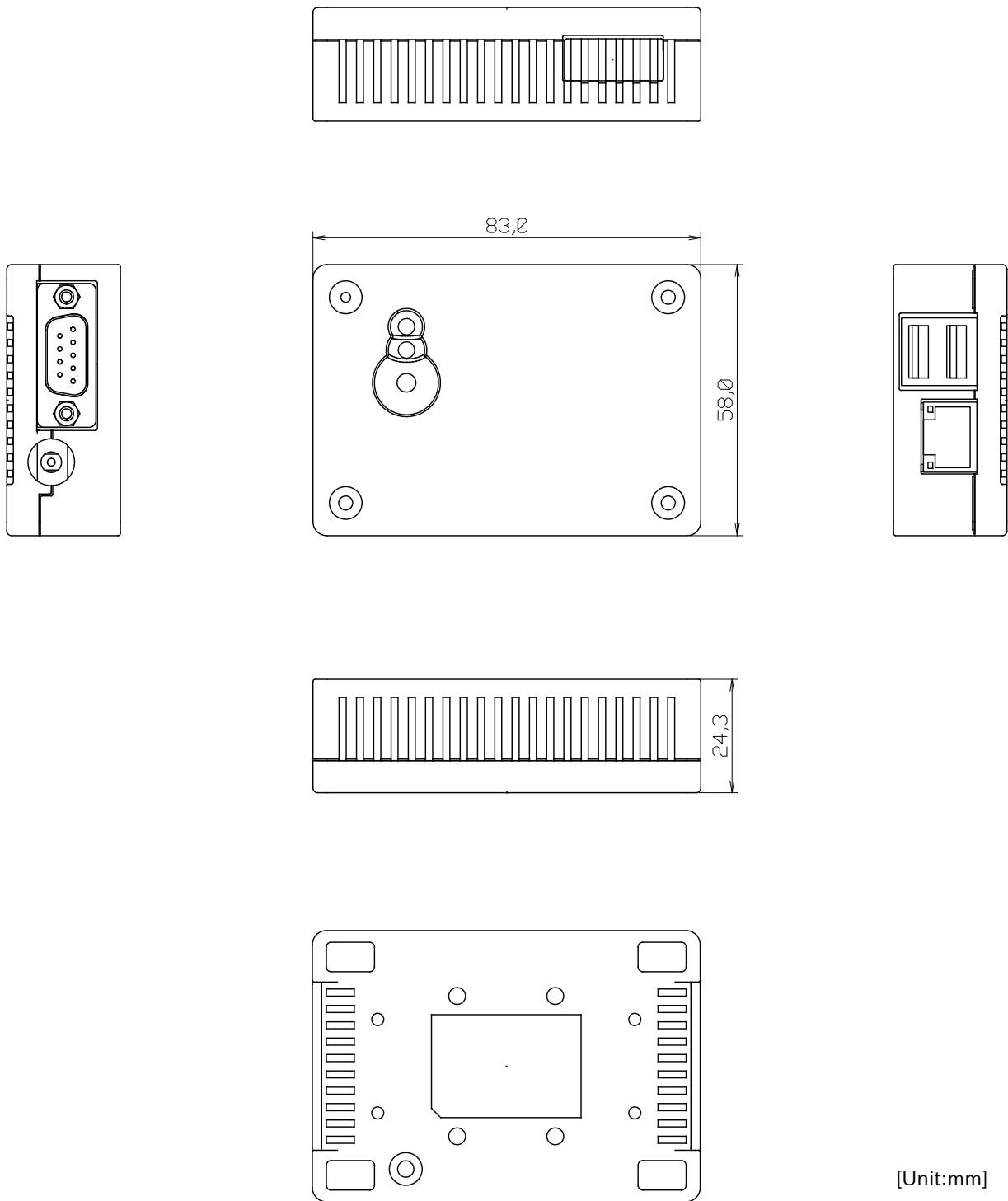
図 6.124 樹脂ケース形状図
