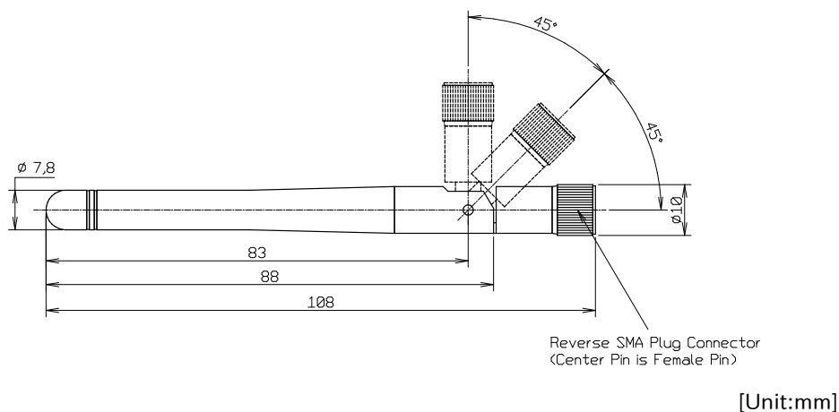
図 6.151 無線 LAN 用 外付けアンテナ 08 形状図
