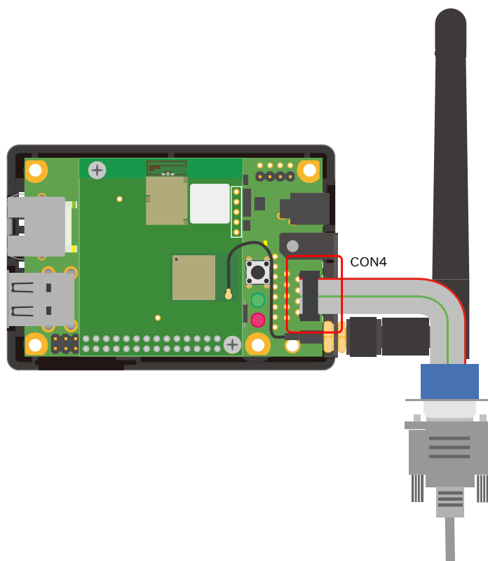
図 6.144 CON4 をシリアルコンソールとして使用する場合の接続例
