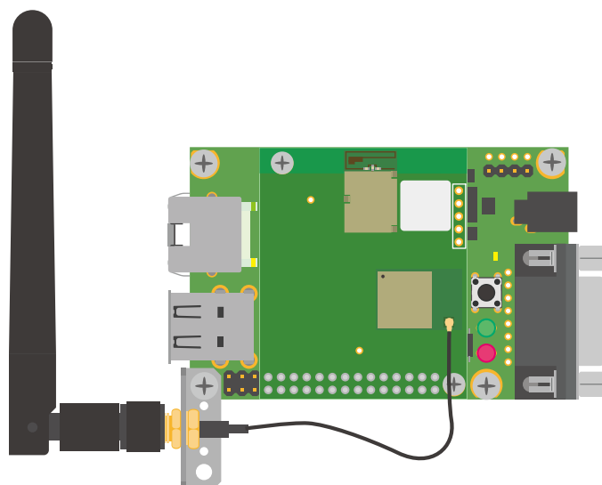
図 6.155 Armadillo-640 へのアンテナ固定金具の固定
