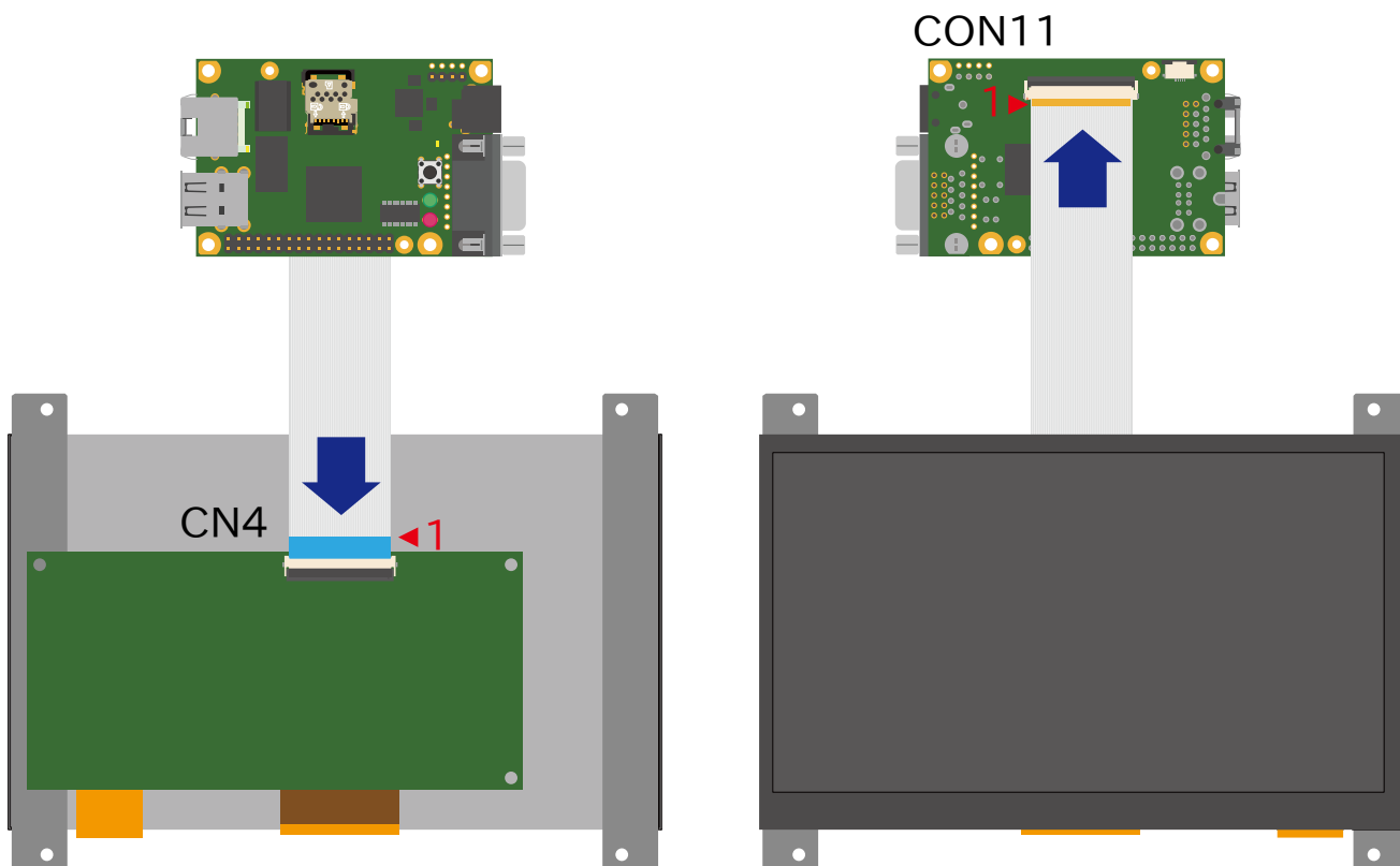
図 3.89 LCD の接続方法
