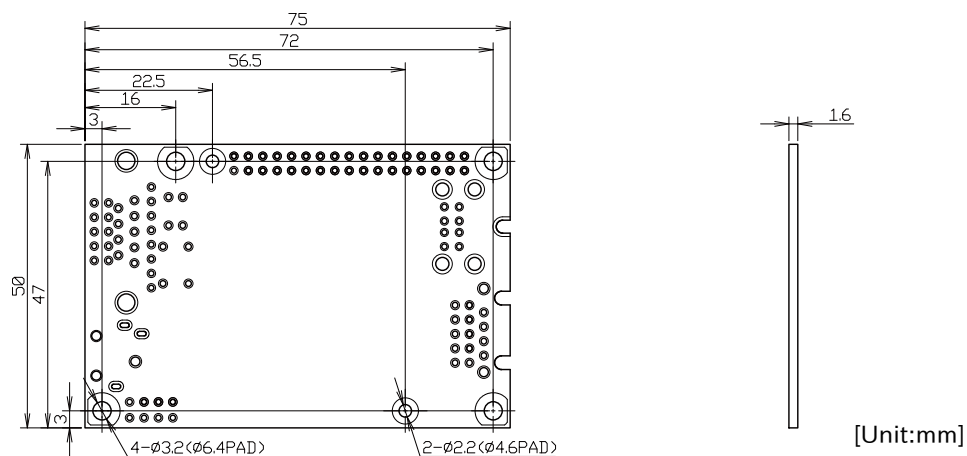
図 3.27 基板形状および固定穴寸法
