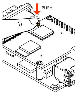
図 6.149 アンテナケーブルコネクタの嵌合
