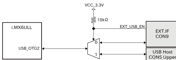
図 3.53 USB OTG2 の接続先の変更
