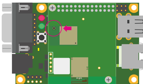
図 6.146 Sterling LWB5+上のコネクタの位置
