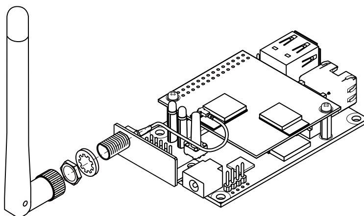
図 6.141 外付けアンテナの組み立て(オプションケース対応のアンテナ固定金具使用)
