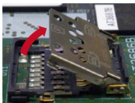
図 3.46 カバーを開ける
