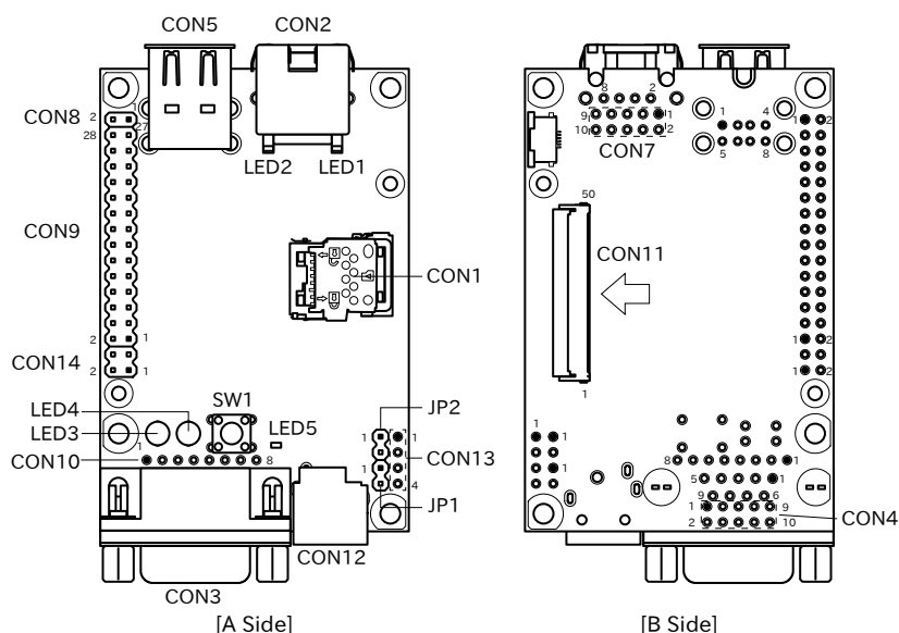
図 3.44 Armadillo-640 のインターフェース
