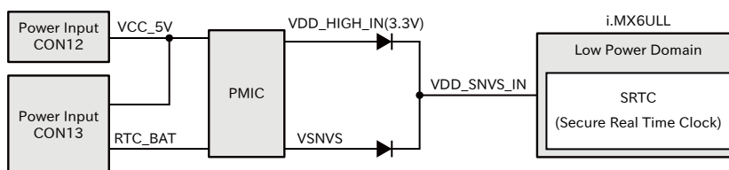
図 3.92 バックアップ電源供給
