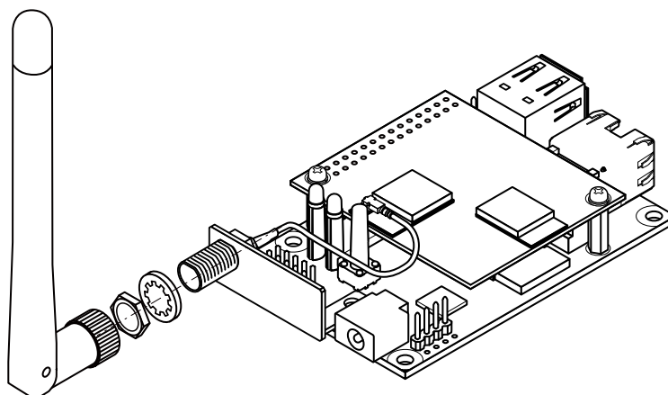
図 6.167 外付けアンテナの組み立て(オプションケース対応のアンテナ固定金具使用)
