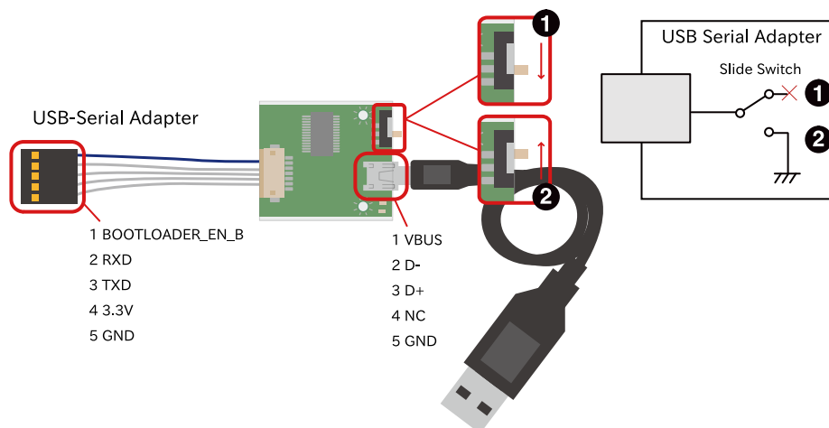
図 6.121 USB シリアル変換アダプタの配線
