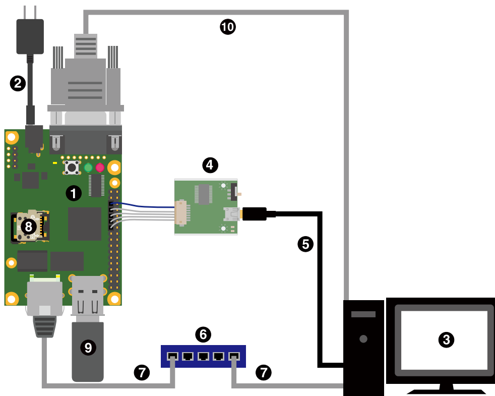
図 3.57 Armadillo-640 の接続例
