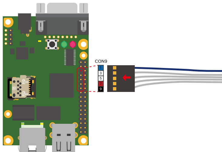
図 3.48 CON9-USB シリアル変換アダプタ接続図
