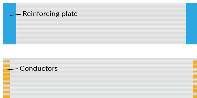
図 3.124 フレキシブルフラットケーブルの形状
