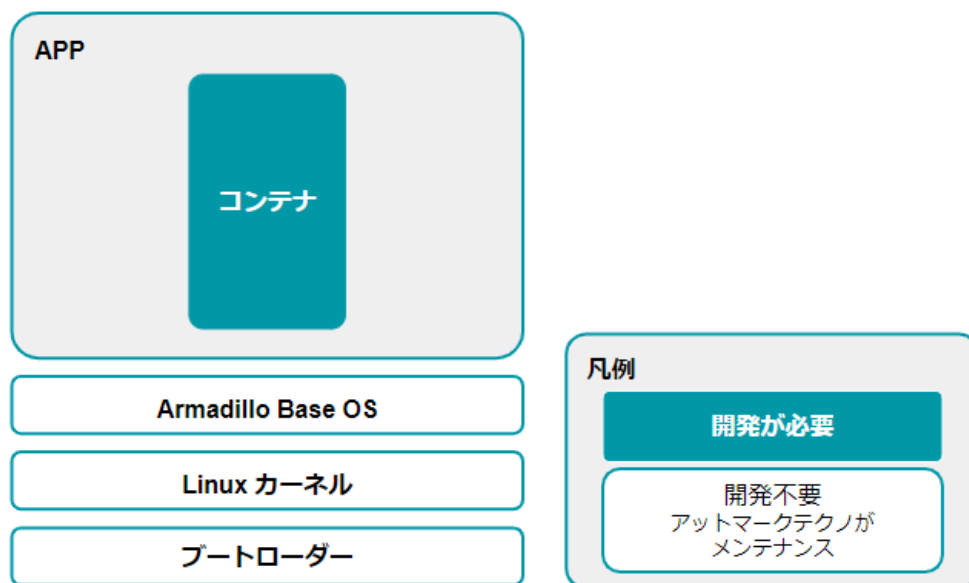
図 3.139 開発者が開発するもの、開発しなくていいもの
