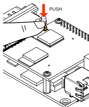
図 6.216 アンテナケーブルコネクタの嵌合
