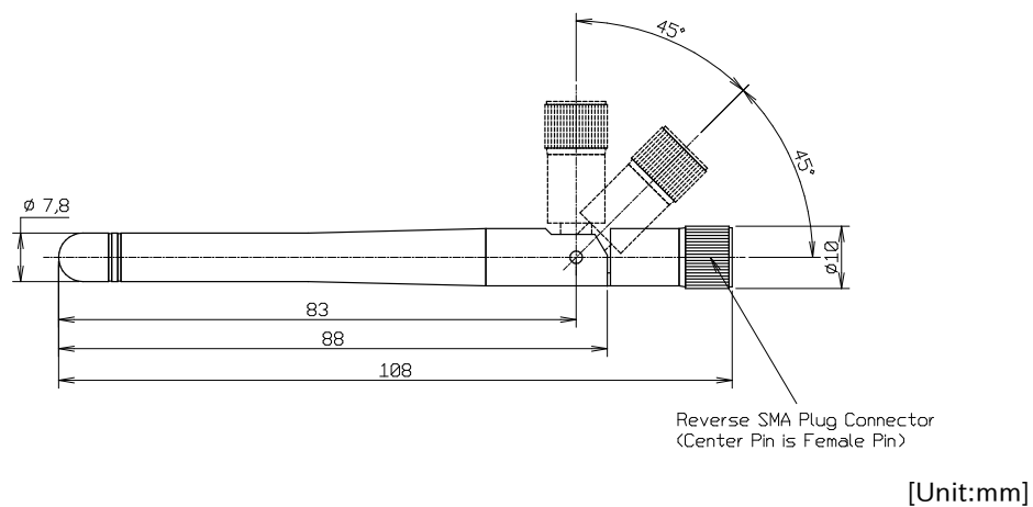
図 6.218 無線 LAN 用 外付けアンテナ 08 形状図
