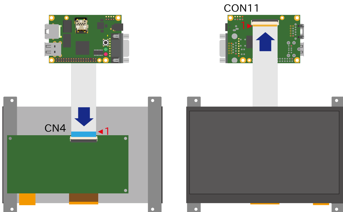
図 3.124 LCD の接続方法
