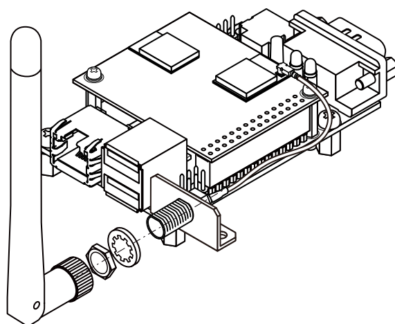
図 6.207 外付けアンテナの組み立て(OP-MNT-ANT-MET-00 使用)
