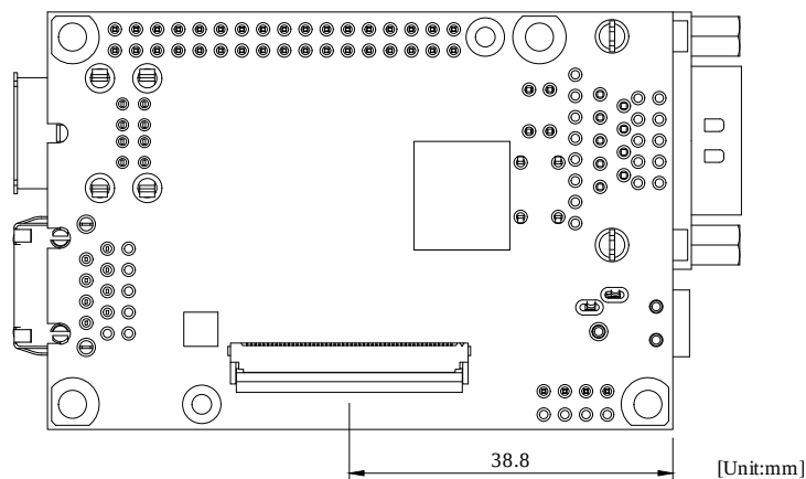
図 3.61 コネクタ中心寸法(B 面側)
