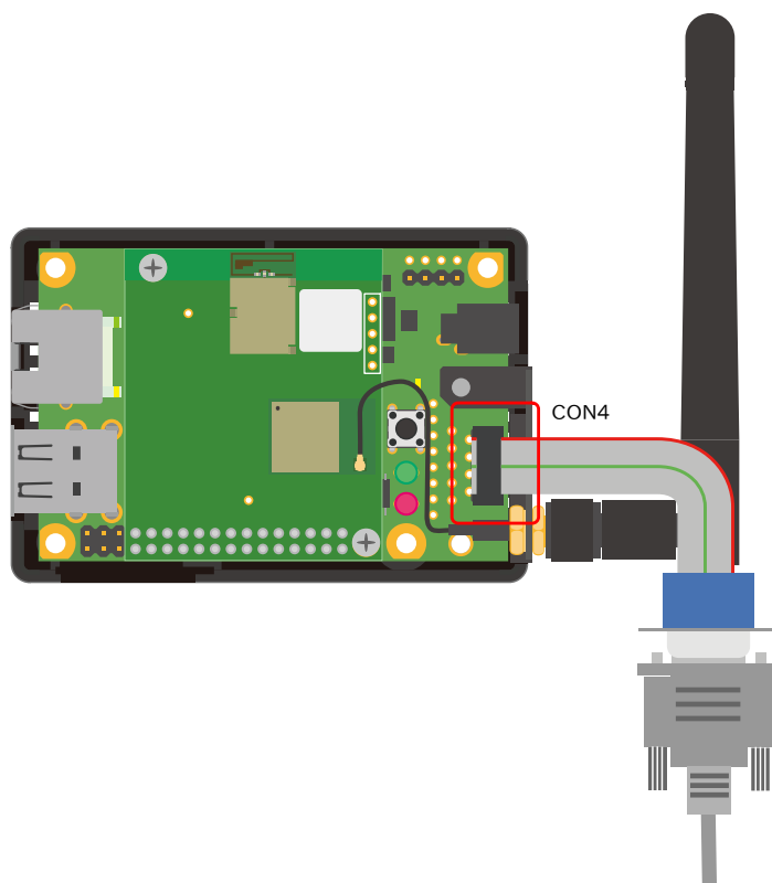
図 6.211 CON4 をシリアルコンソールとして使用する場合の接続例
