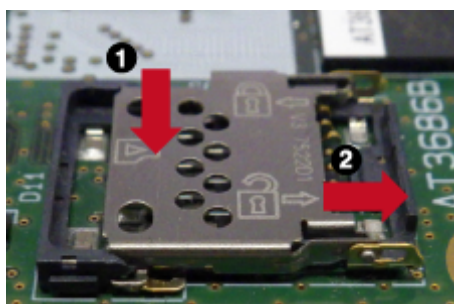
図 3.78 カバーのロックを解除する
