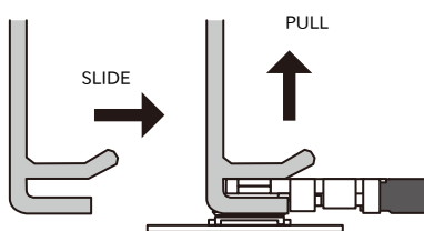
図 6.217 挿抜治具によるアンテナケーブルコネクタの抜去
