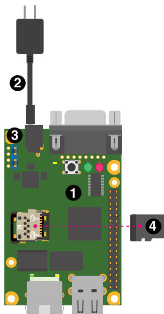
図 3.19 Armadillo-640 を初期化する接続
