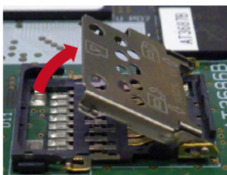
図 3.79 カバーを開ける
