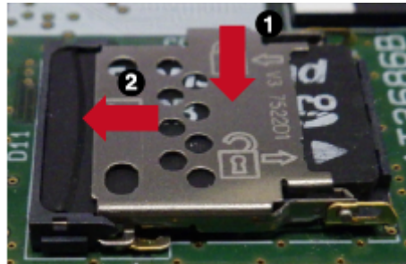
図 3.83 カバーをロックする
