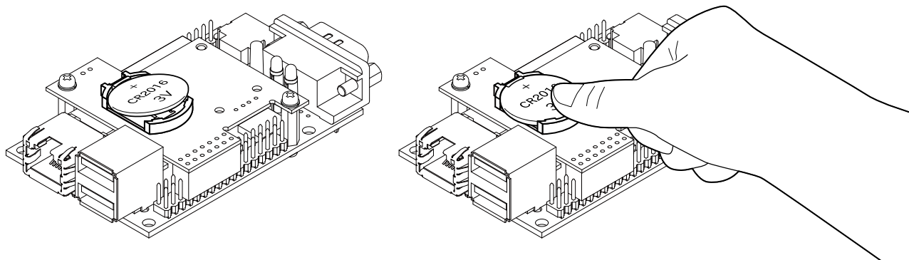
図 6.199 電池ホルダに電池を取り付ける
