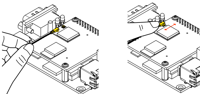
図 6.215 アンテナケーブルコネクタのセット
