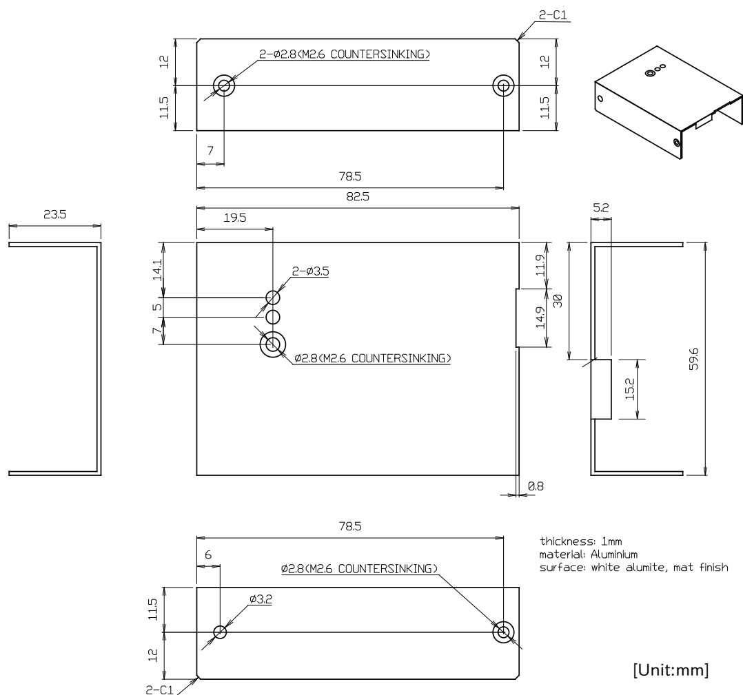
図 6.193 金属ケース(上板)寸法図
