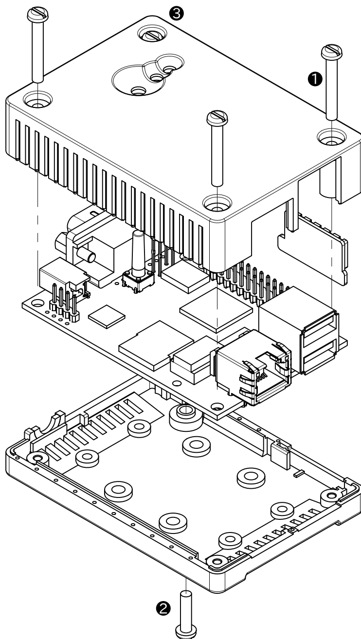
図 6.190 Armadillo-600 シリーズ オプションケース(樹脂製)の組み立て
