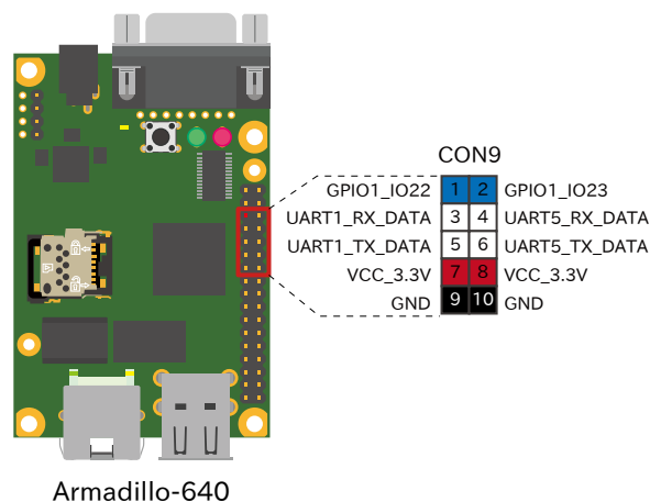
図 6.189 Armadillo-640 のシリアル信号線
