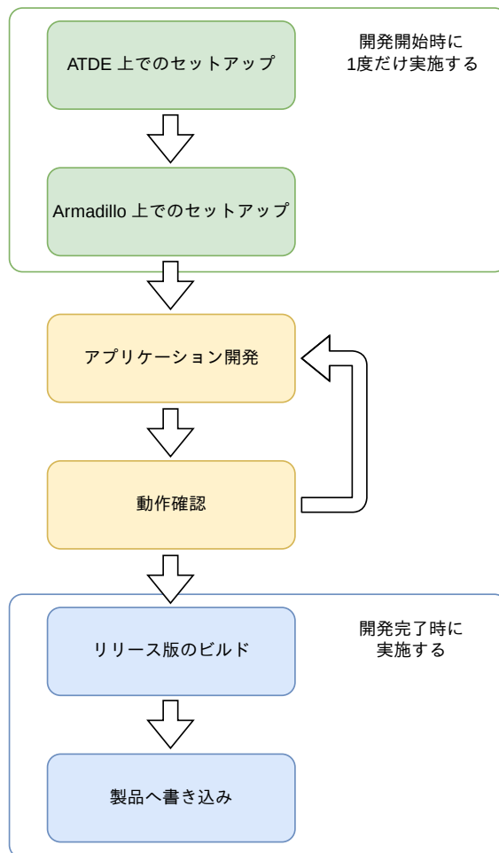
図 3.211 C 言語によるアプリケーション開発の流れ
