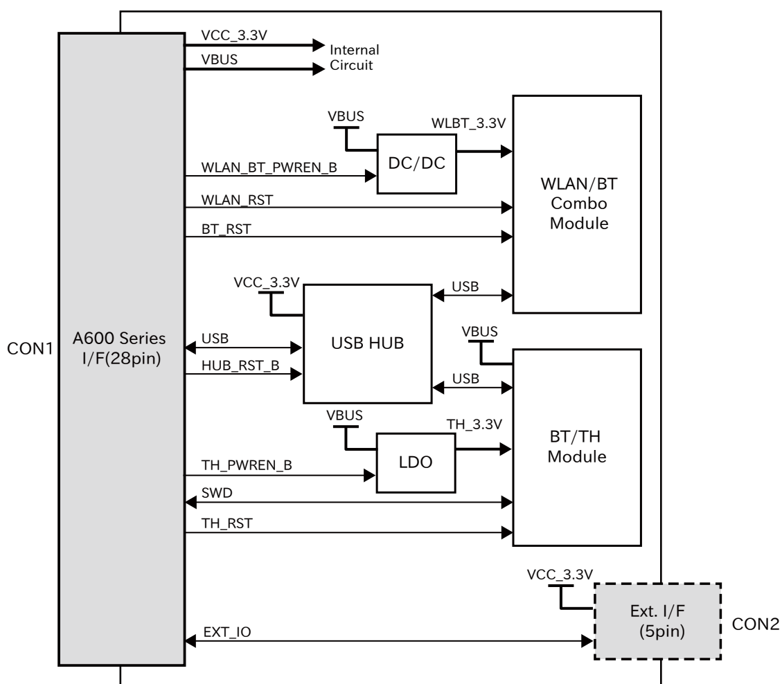
図 6.203 WLAN コンボ、BT/TH オプションモジュールのブロック図
