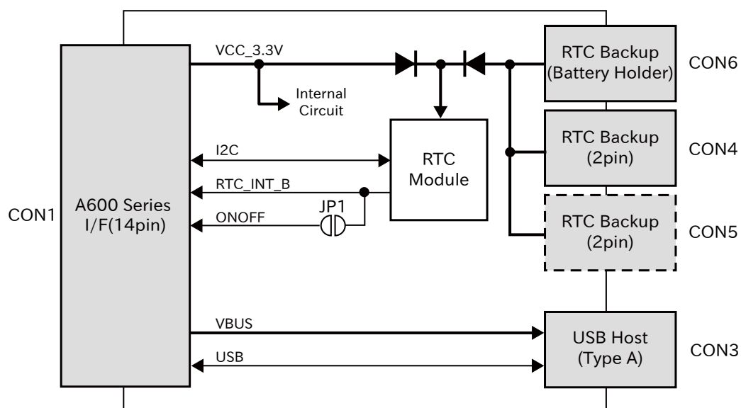
図 6.195 RTC オプションモジュールのブロック図
