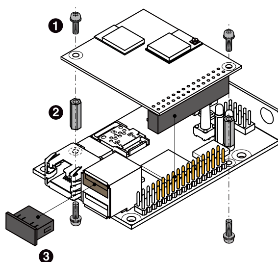
図 6.206 WLAN コンボ、BT/TH オプションモジュールの組み立て
