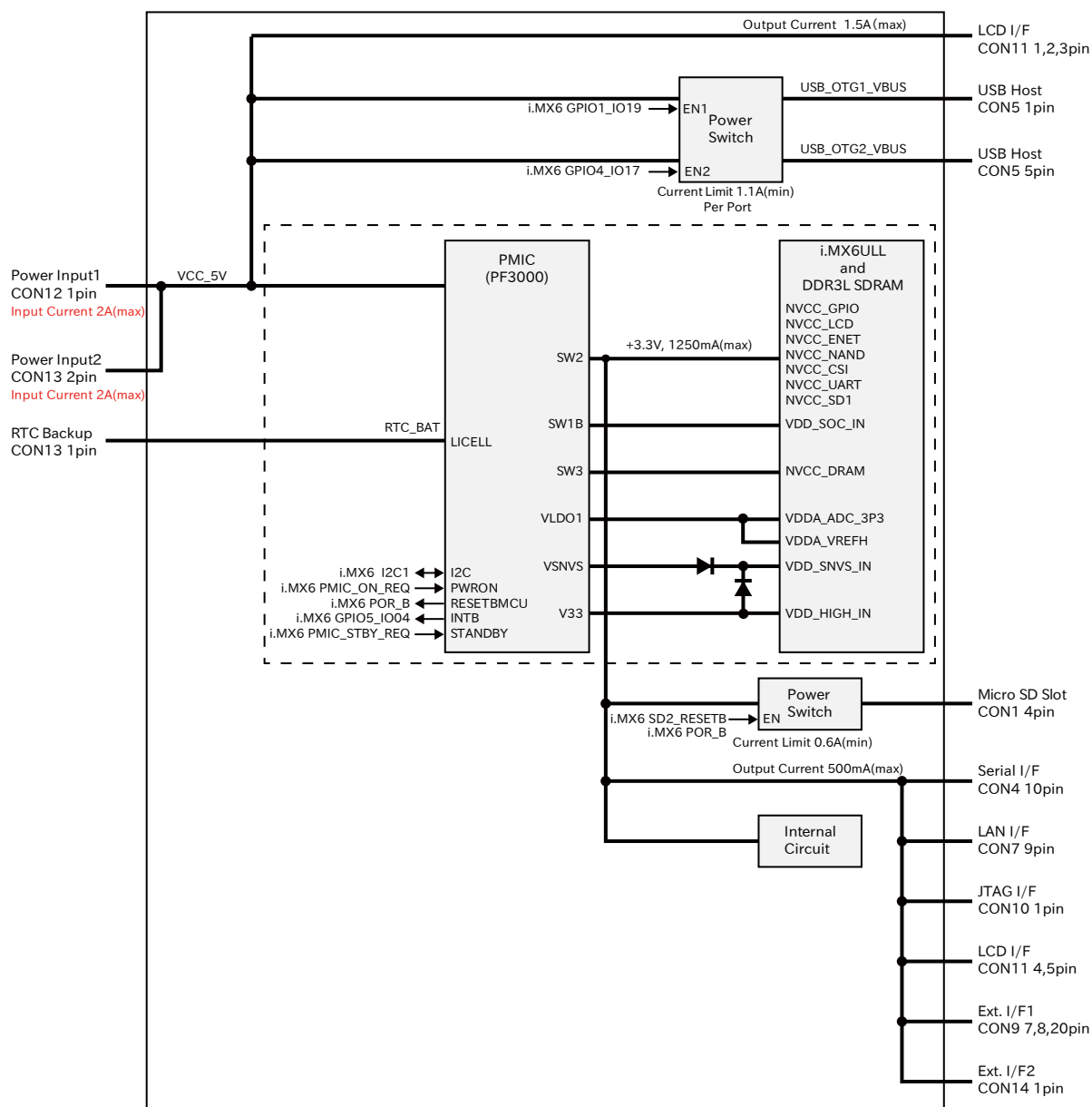
図 3.57 電源回路の構成
