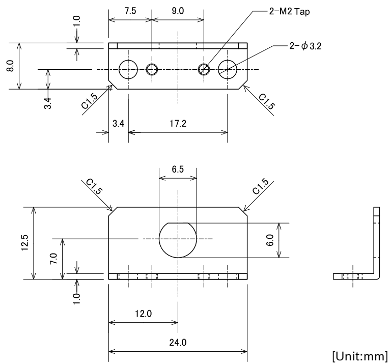
図 6.225 アンテナ固定金具 形状図
