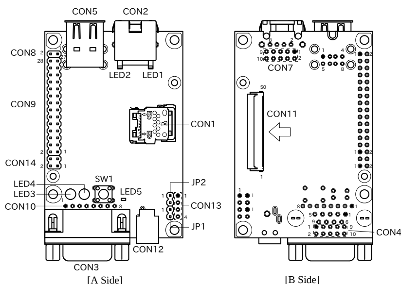
図 3.77 Armadillo-640 のインターフェース
