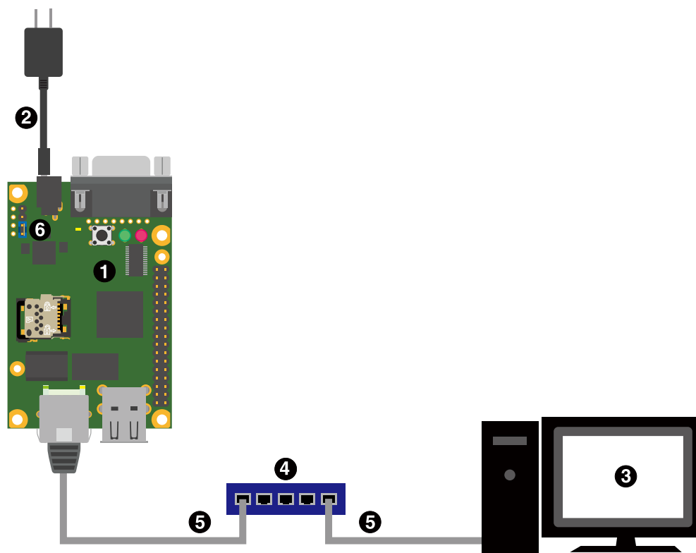
図 3.23 ABOS にアクセスするための接続
