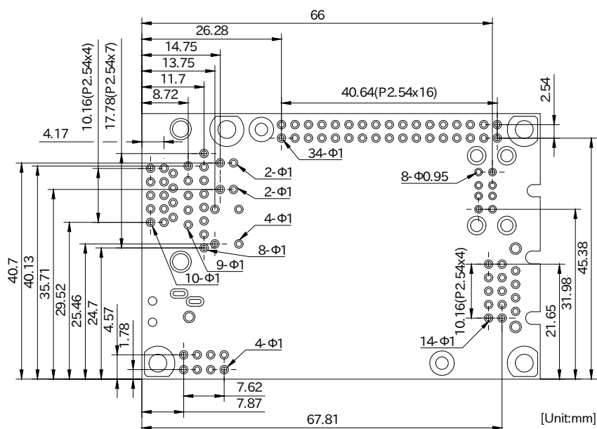
図 3.62 コネクタ穴寸法
