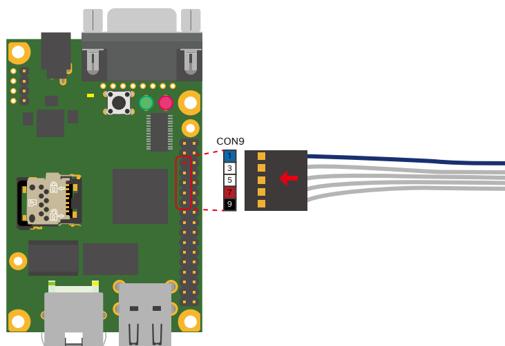
図 3.48 CON9-USB シリアル変換アダプタ接続図
