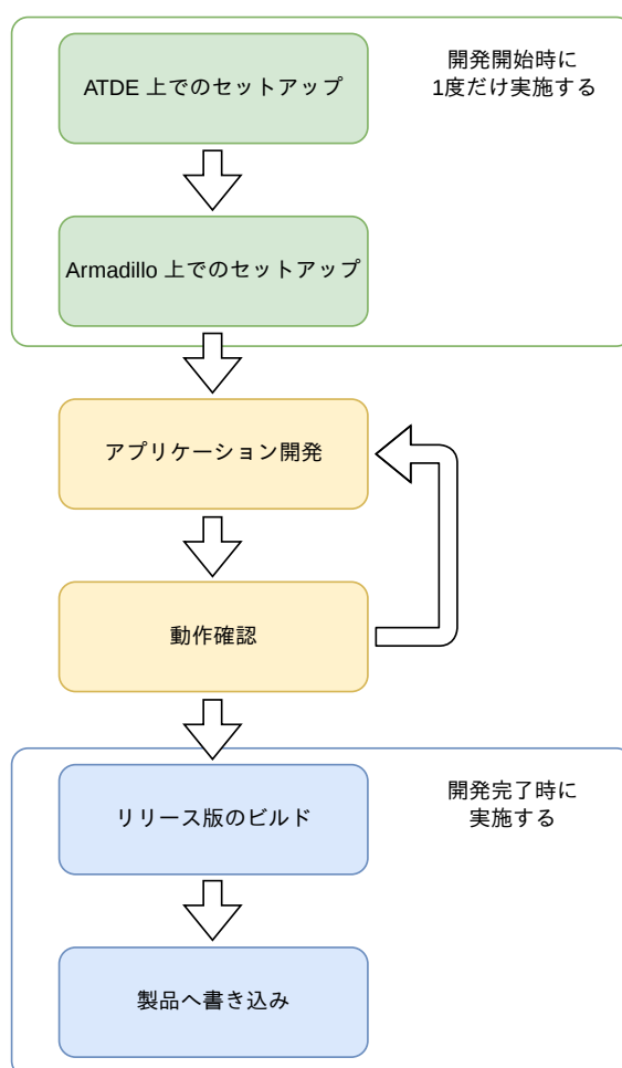
図 3.178 CUI アプリケーション開発の流れ
