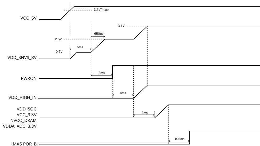
図 3.58 電源シーケンス
