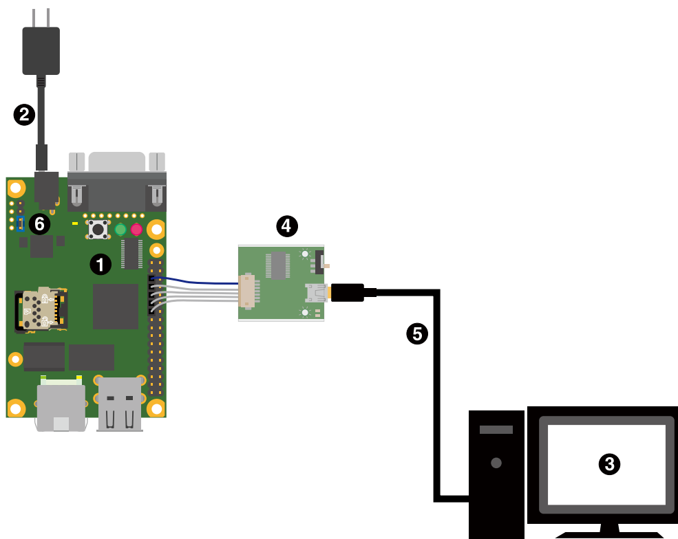
図 3.49 シリアルコンソールを使用する配線例
