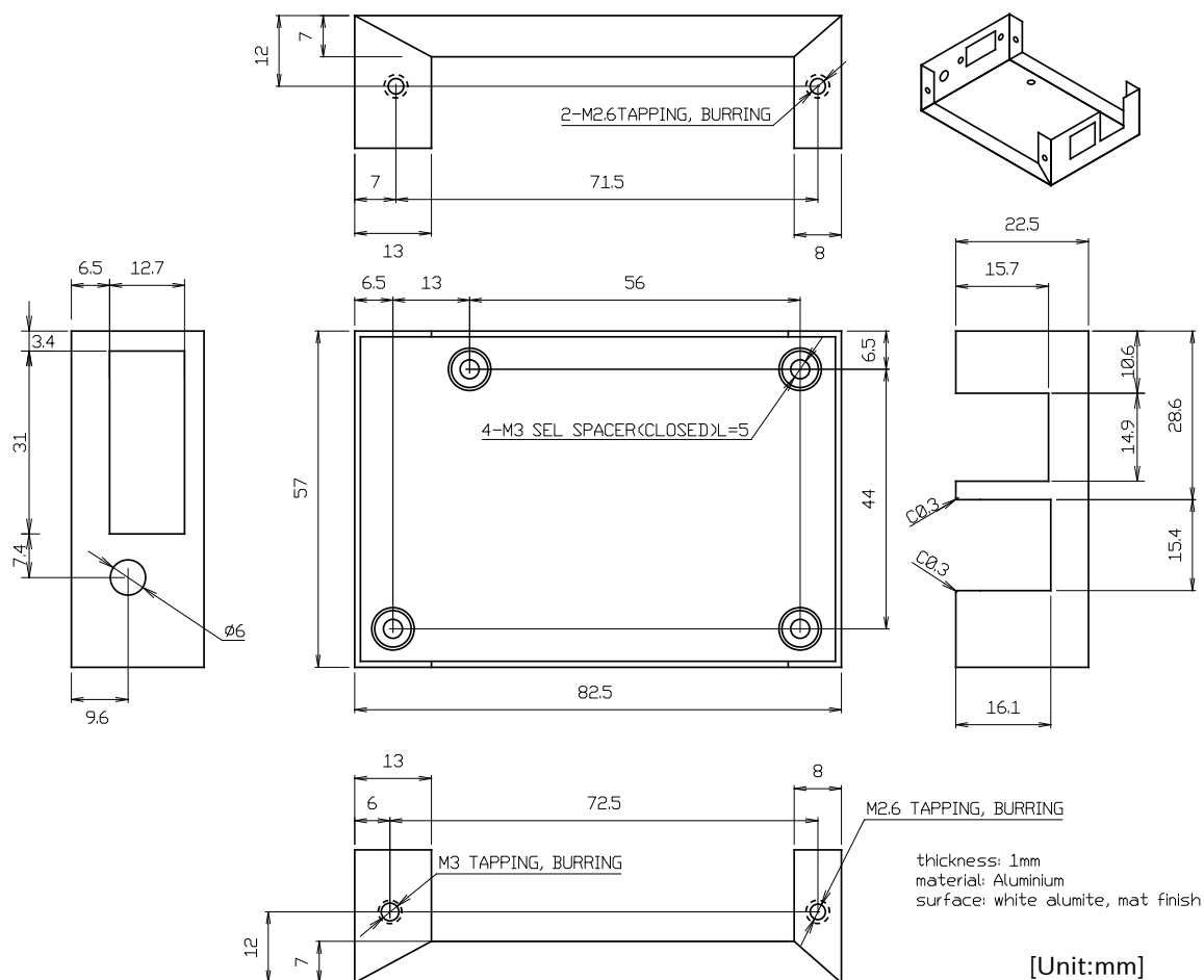
図 6.194 金属ケース(下板)寸法図
