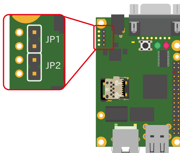
図 3.20 ジャンパピンの位置
