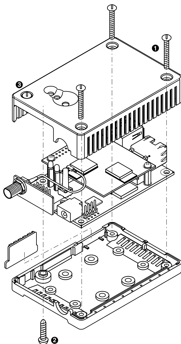
図 6.209 ケースの組み立て
