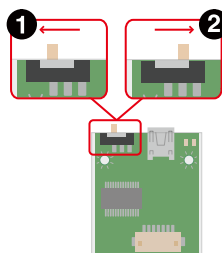
図 3.47 スライドスイッチの設定
