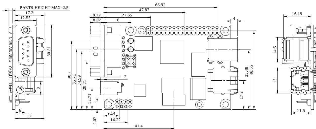
図 3.60 コネクタ中心寸法(A 面側)
