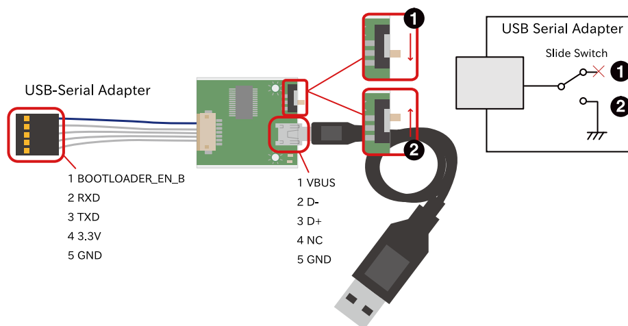
図 6.188 USB シリアル変換アダプタの配線
