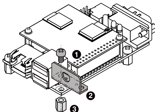
図 6.223 Armadillo-640 へのアンテナ固定金具の固定
