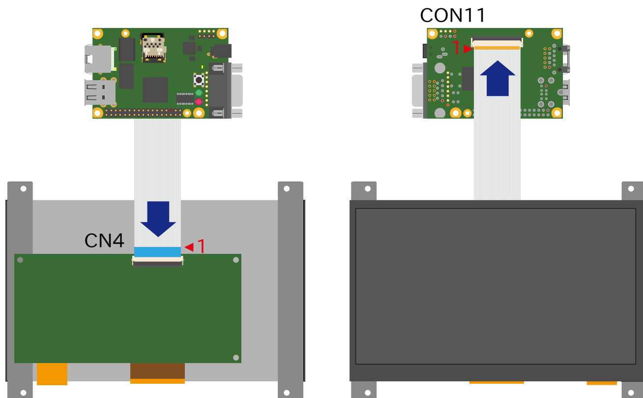
図 3.118 LCD の接続方法
