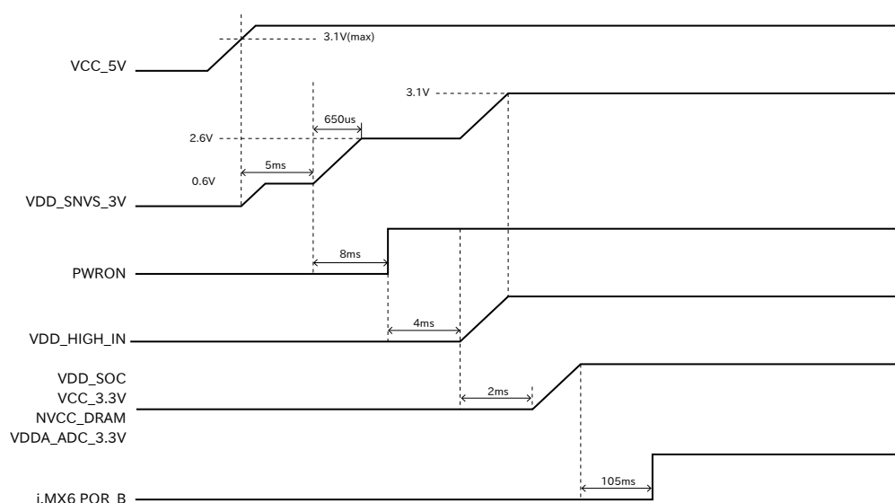
図 3.52 電源シーケンス
