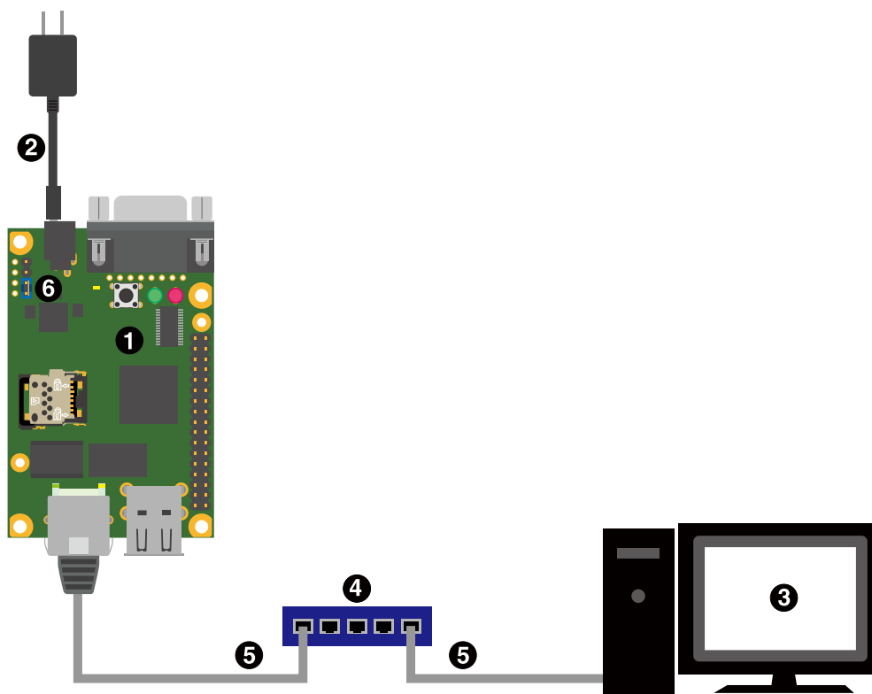
図 3.17 ABOS にアクセスするための接続
