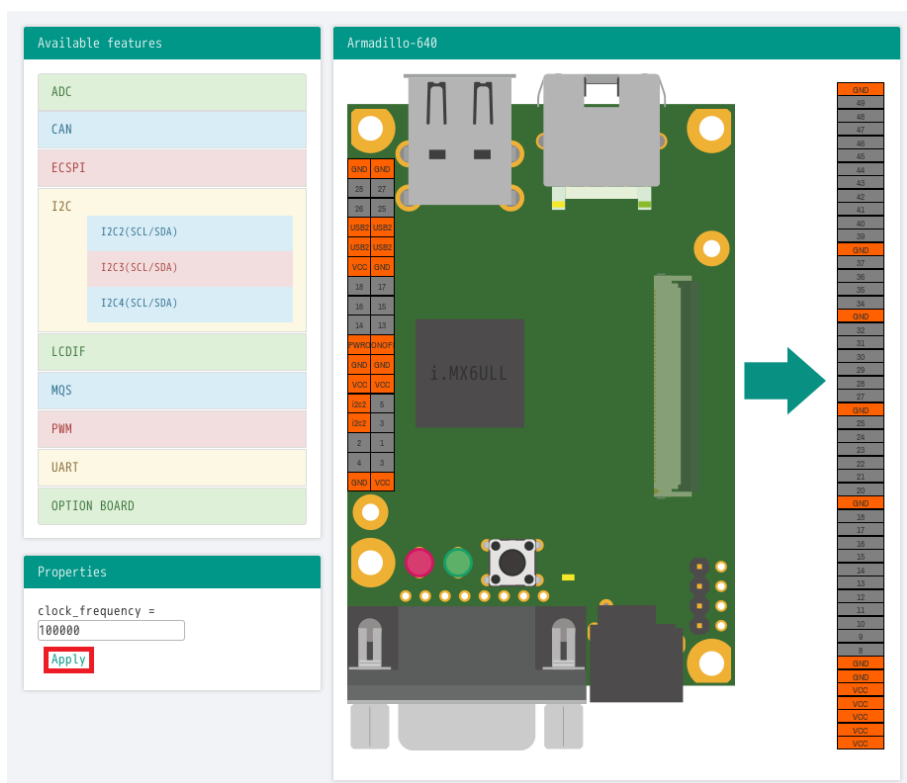
図 3.65 プロパティの保存
