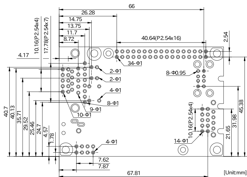
図 3.56 コネクタ穴寸法
