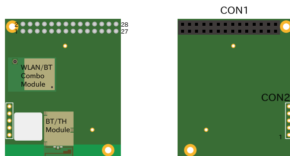
図 6.217 WLAN コンボ、BT/TH オプションモジュールのインターフェース
