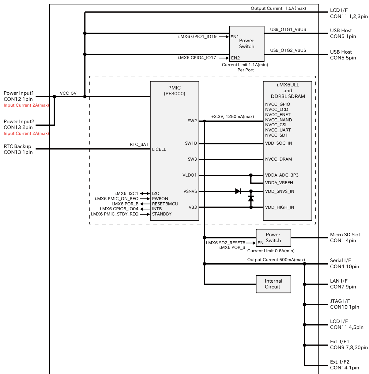
図 3.51 電源回路の構成
