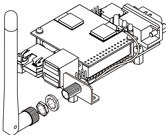
図 6.220 外付けアンテナの組み立て(OP-MNT-ANT-MET-00 使用)
