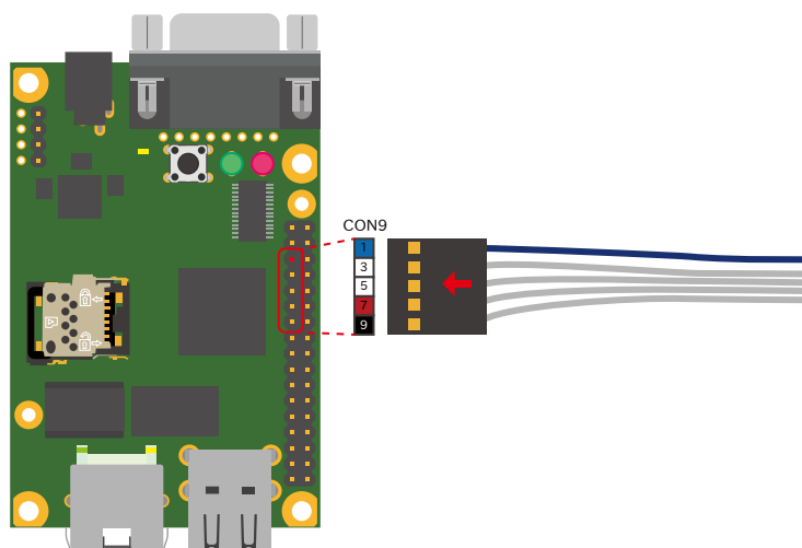
図 3.42 CON9-USB シリアル変換アダプタ接続図
