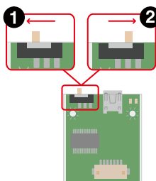
図 3.41 スライドスイッチの設定
