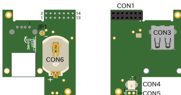
図 6.206 RTC オプションモジュールのインターフェース
