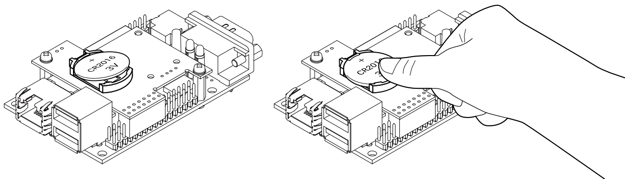
図 6.209 電池ホルダに電池を取り付ける
