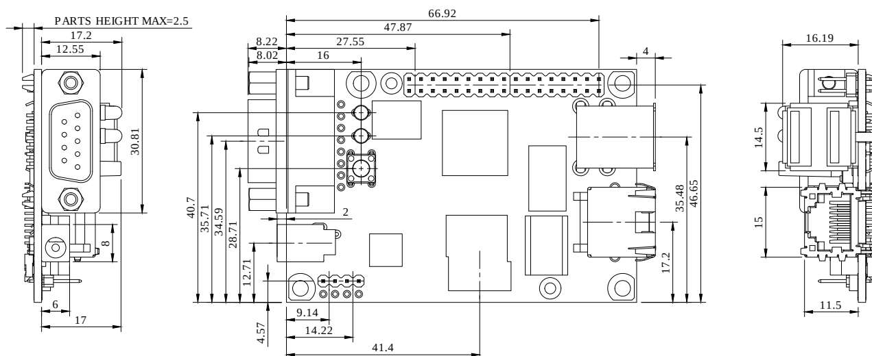
図 3.54 コネクタ中心寸法(A 面側)
