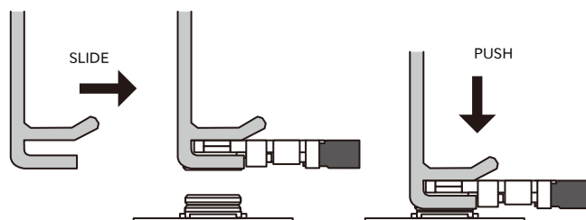
図 6.227 挿抜治具によるアンテナケーブルコネクタの嵌合
