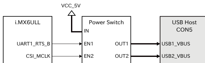
図 3.81 USB ホストインターフェースの電源制御
