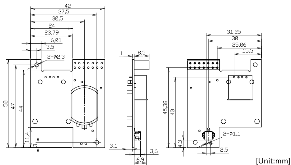
図 6.211 RTC オプションモジュール形状
