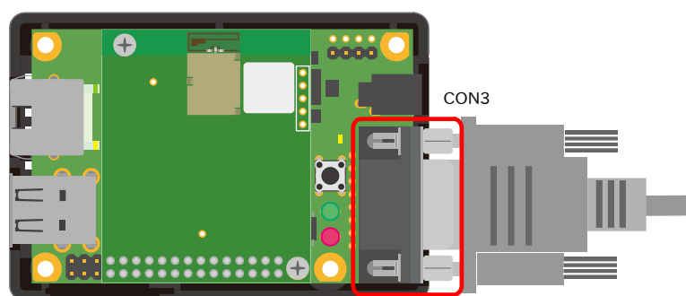
図 6.225 CON3 をシリアルコンソールとして使用する場合の接続例
