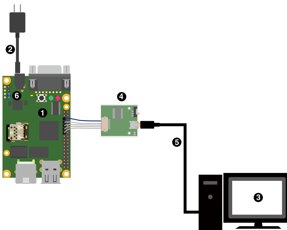
図 3.43 シリアルコンソールを使用する配線例
