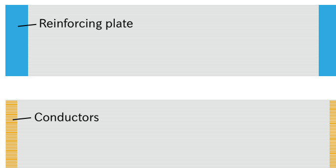
図 3.119 フレキシブルフラットケーブルの形状
