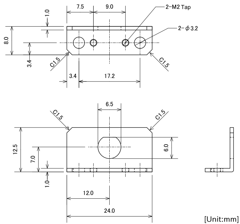
図 6.238 アンテナ固定金具 形状図
