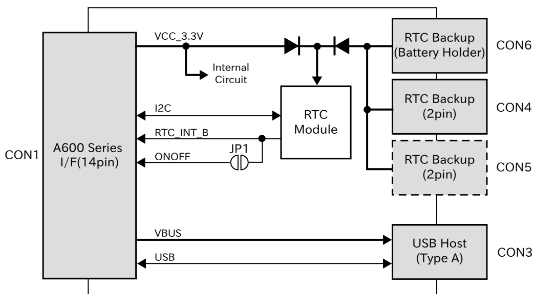
図 6.205 RTC オプションモジュールのブロック図
