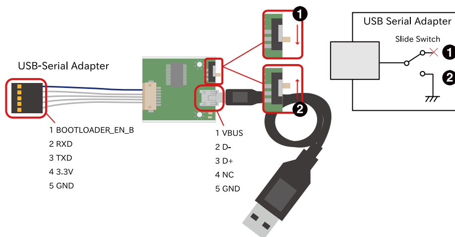
図 6.198 USB シリアル変換アダプタの配線
