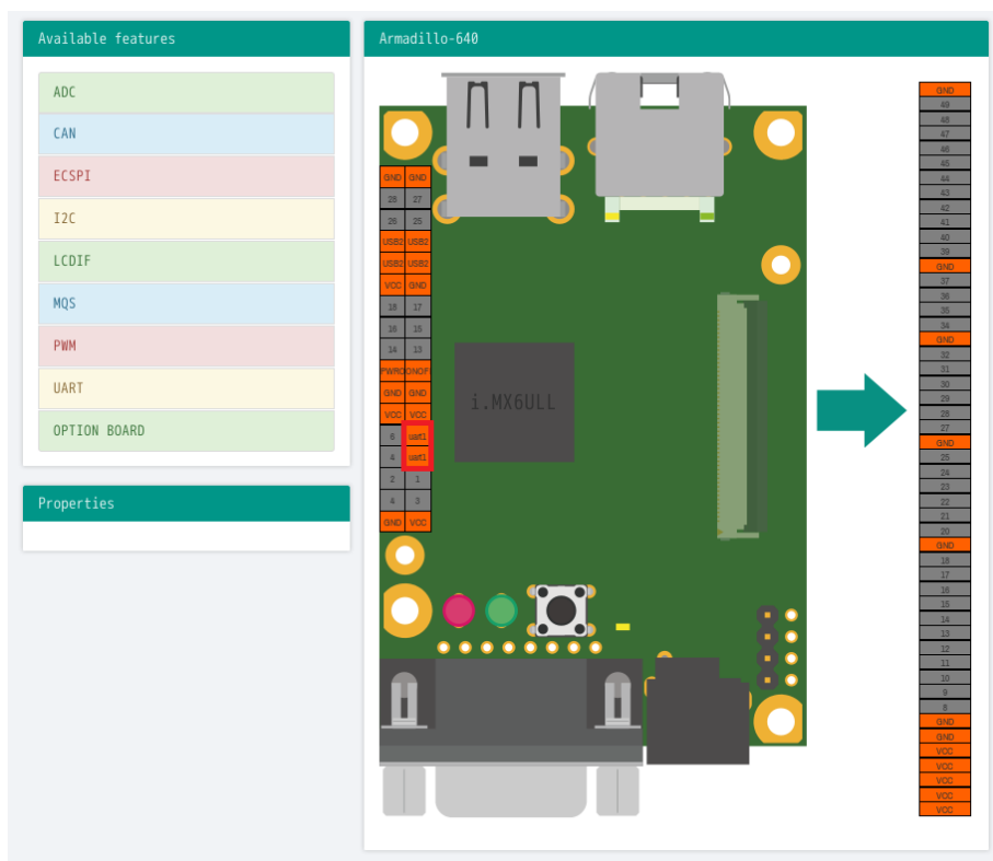
図 3.62 CON9 3/5 ピンへのドロップ
