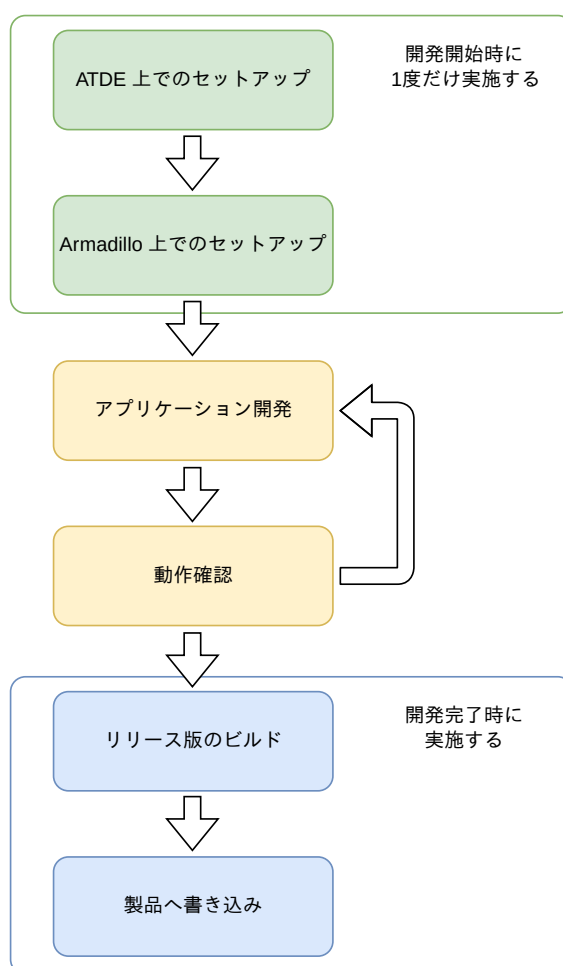
図 3.172 CUI アプリケーション開発の流れ
