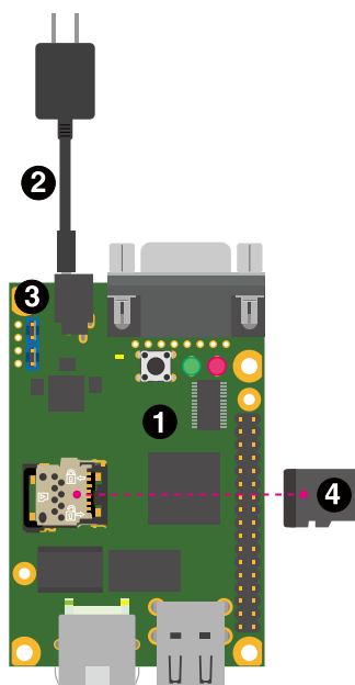
図 3.13 Armadillo-640 を初期化する接続
