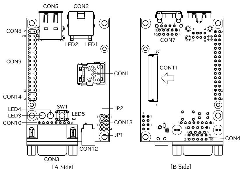
図 3.71 Armadillo-640 のインターフェース
