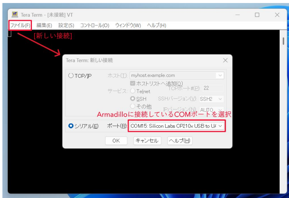
図 3.46 Armadillo を接続している COM ポートを指定
