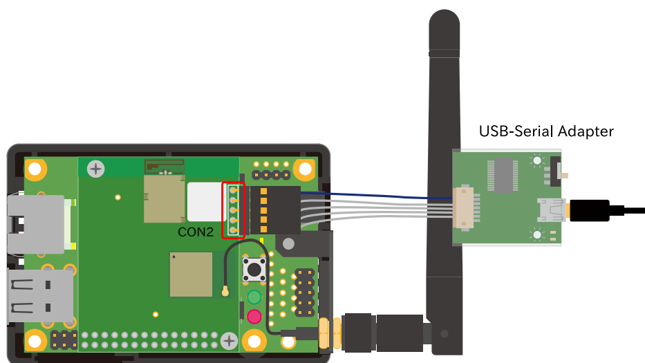
図 6.223 オプションモジュールの CON2 をシリアルコンソールとして使用する場合の接続例
