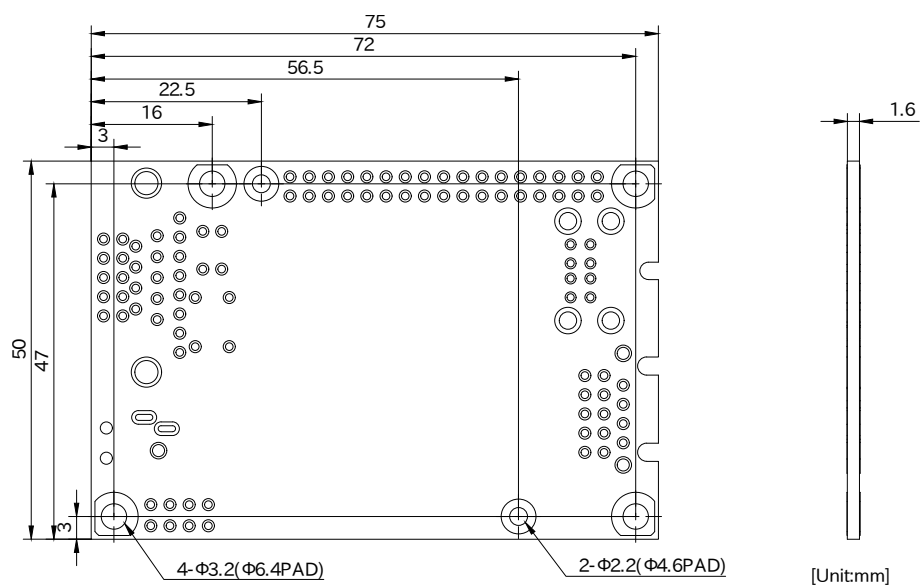
図 3.53 基板形状および固定穴寸法
