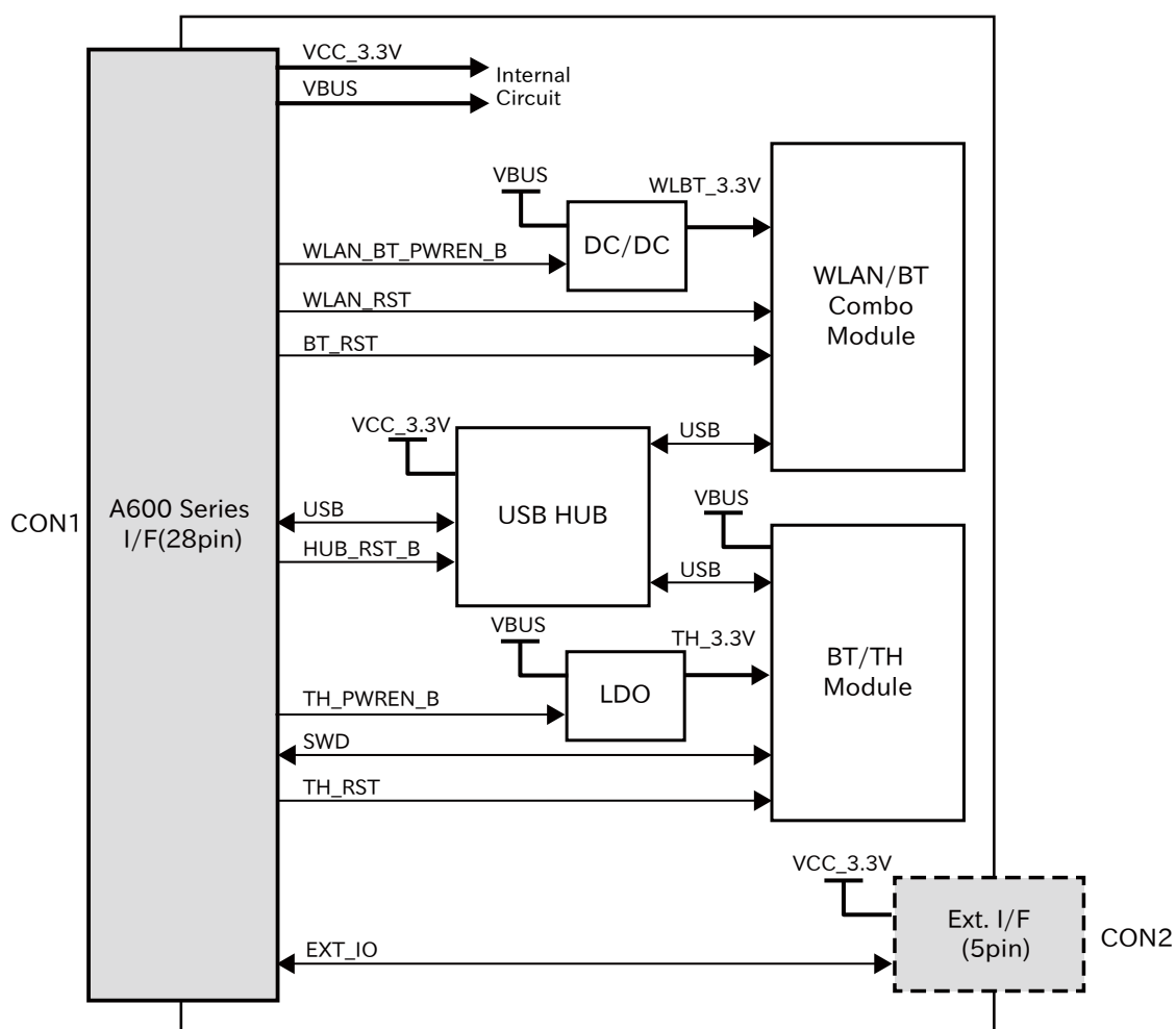
図 6.216 WLAN コンボ、BT/TH オプションモジュールのブロック図
