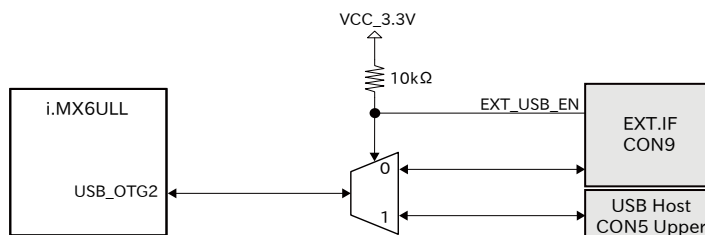
図 3.80 USB_OTG2 の接続先の変更
