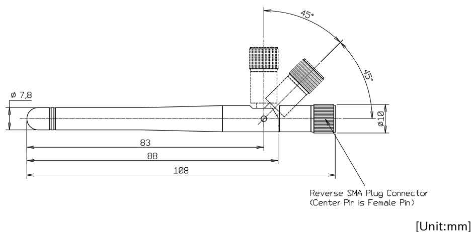
図 6.231 無線 LAN 用 外付けアンテナ 08 形状図
