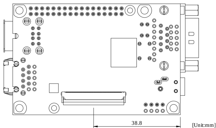
図 3.55 コネクタ中心寸法(B 面側)
