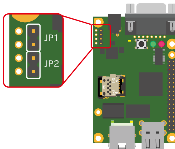
図 3.14 ジャンパピンの位置
