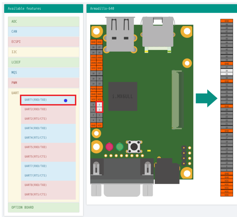
図 3.61 UART1(RXD/TXD)のドラッグ
