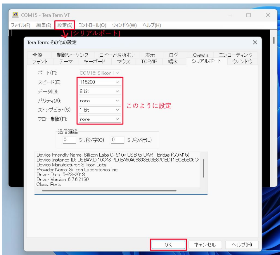
図 3.47 Armadillo を接続しているシリアルポートの設定
