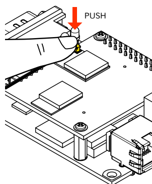
図 6.230 アンテナケーブルコネクタの嵌合
