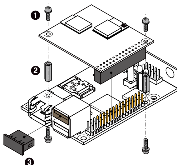
図 6.220 WLAN コンボ、BT/TH オプションモジュールの組み立て
