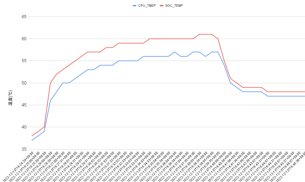
図 6.148 Armadillo-IoT ゲートウェイ G4 で取得した温度のグラフ
