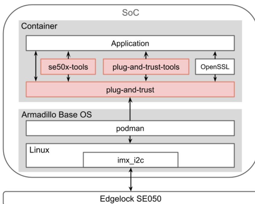
図 6.191 Plug & Trust Middleware の周辺のソフトウェアスタック
