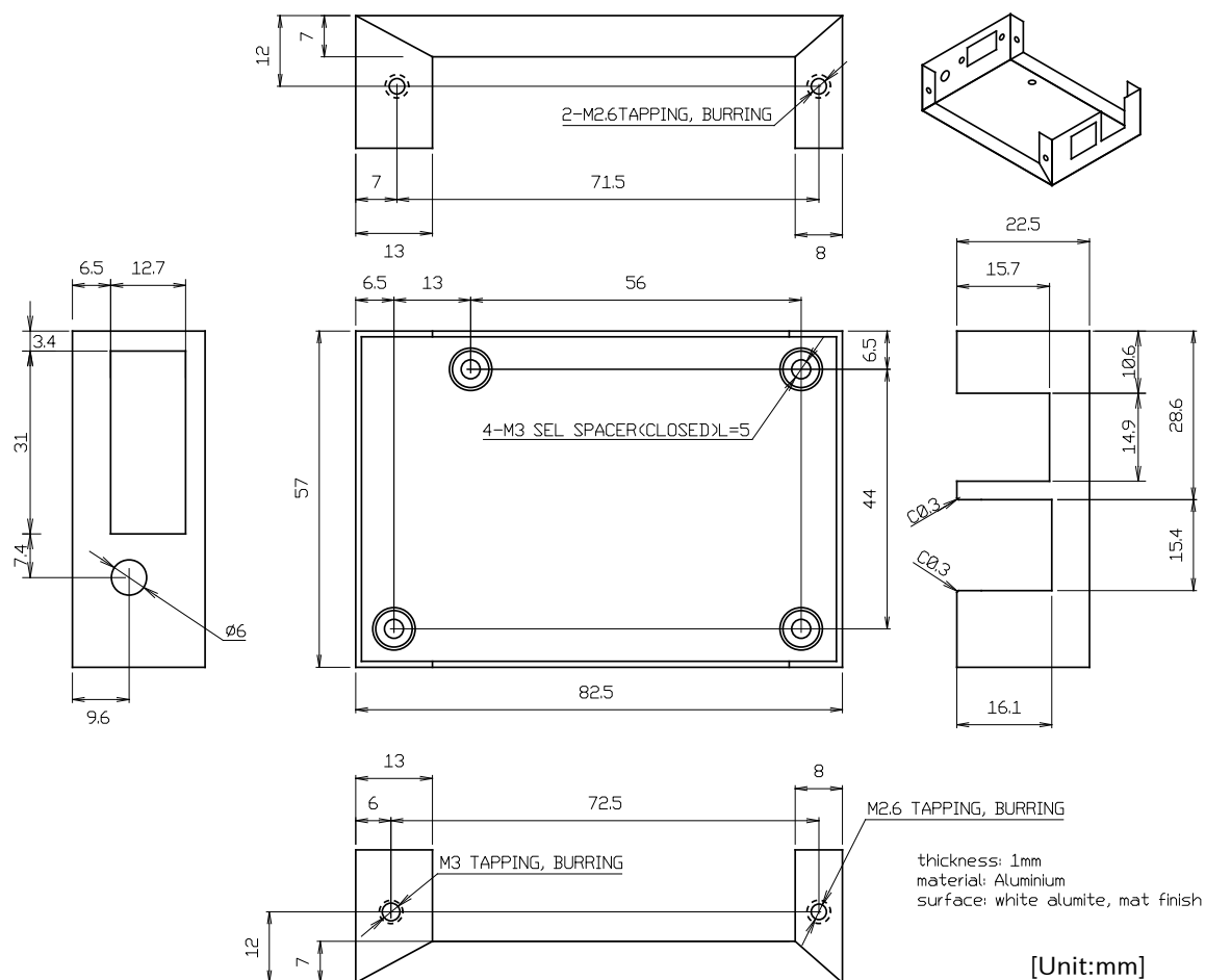
図 6.205 金属ケース(下板)寸法図
