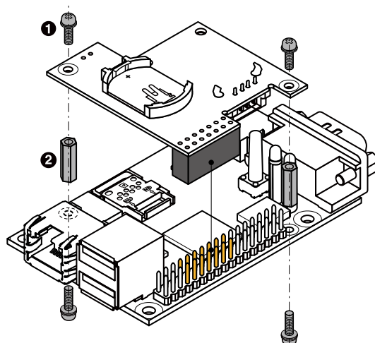
図 6.209 RTC オプションモジュールの組み立て
