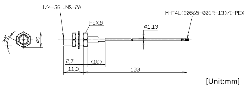
図 6.233 無線 LAN 用 外付けアンテナケーブル 08 形状図
