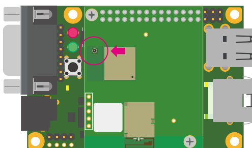
図 6.227 Sterling LWB5+上のコネクタの位置
