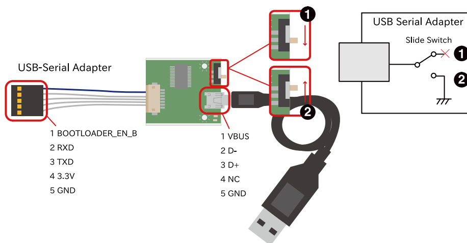
図 6.199 USB シリアル変換アダプタの配線
