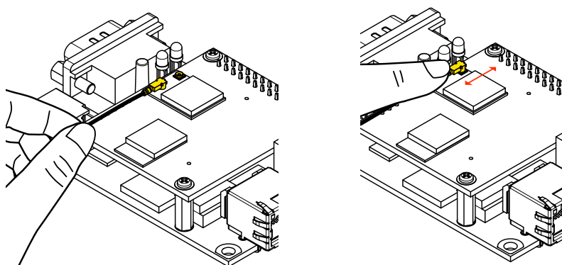
図 6.229 アンテナケーブルコネクタのセット
