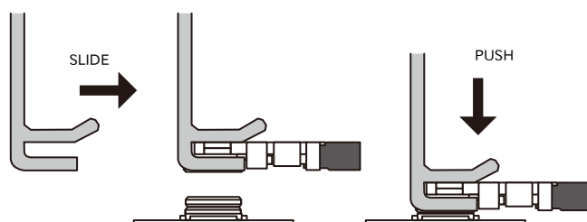
図 6.228 挿抜治具によるアンテナケーブルコネクタの嵌合
