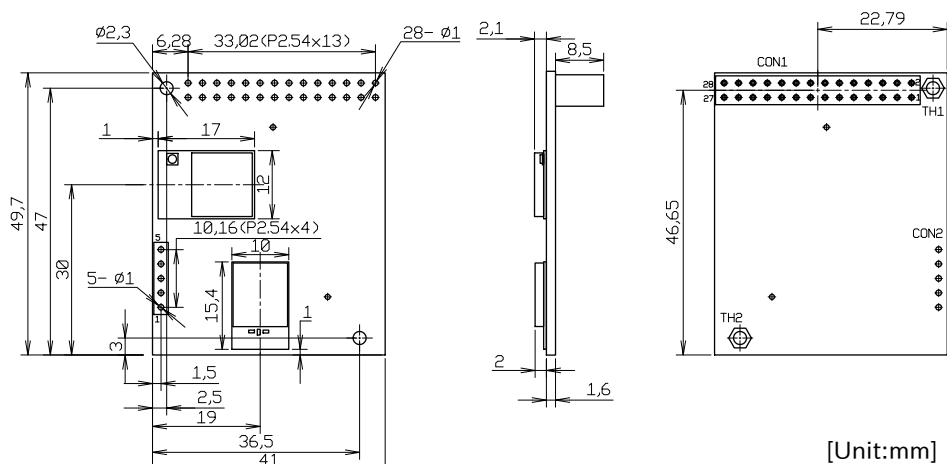
図 6.219 WLAN コンボ、BT/TH オプションモジュール形状図
