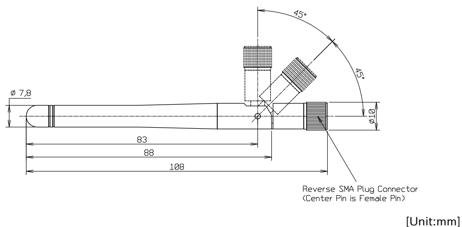
図 6.232 無線 LAN 用 外付けアンテナ 08 形状図
