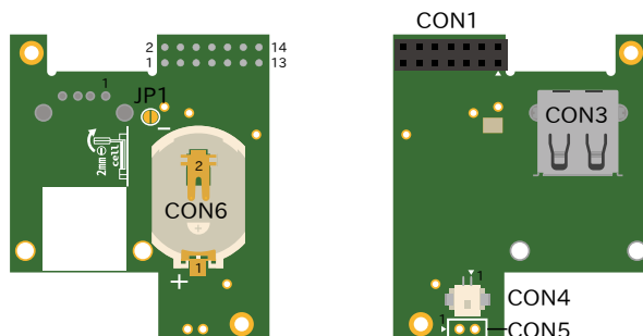
図 6.207 RTC オプションモジュールのインターフェース
