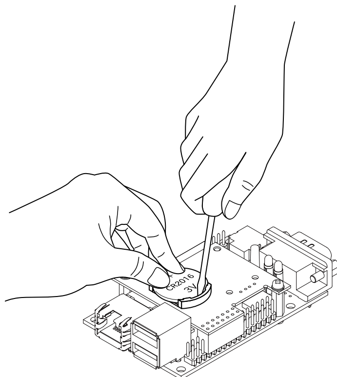
図 6.211 電池ホルダから電池を取り外す
